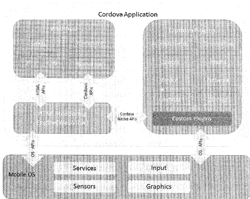
图 10.3 Cordova 架构图
