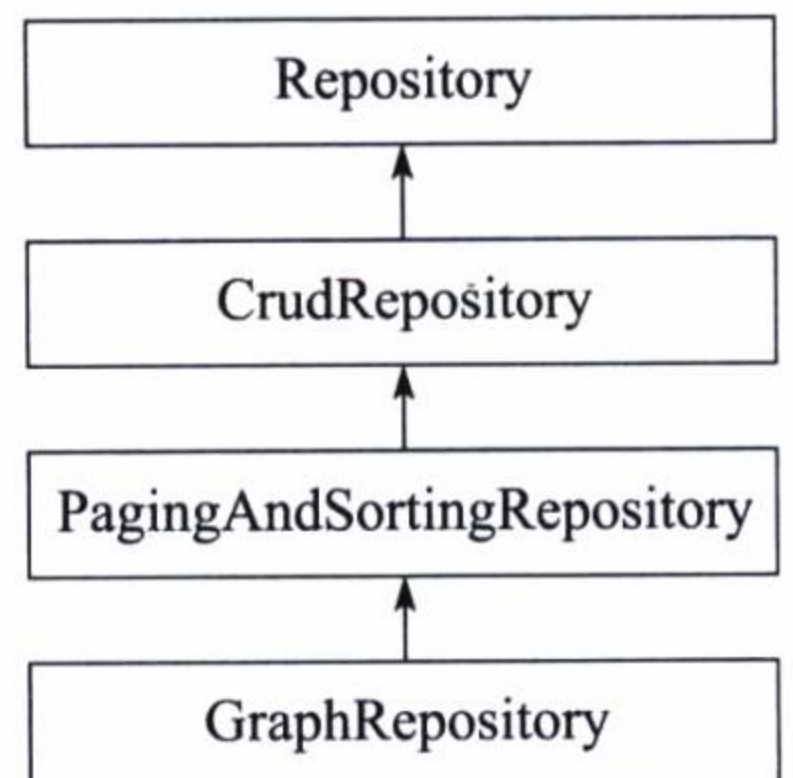
图 2-6 GraphRepository 接口继承关系
