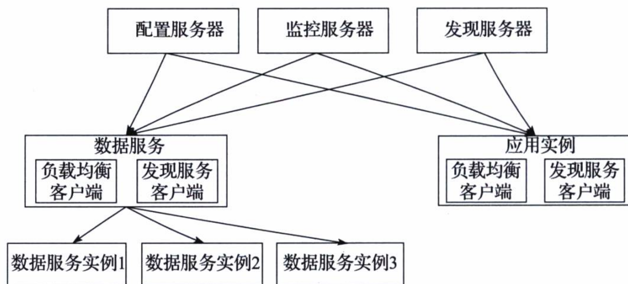
图 9-4 微服务高可用服务体系结构图
