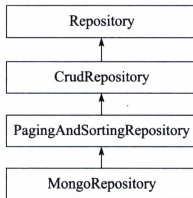
图 2-4 MongoRepository 接口继承关系
