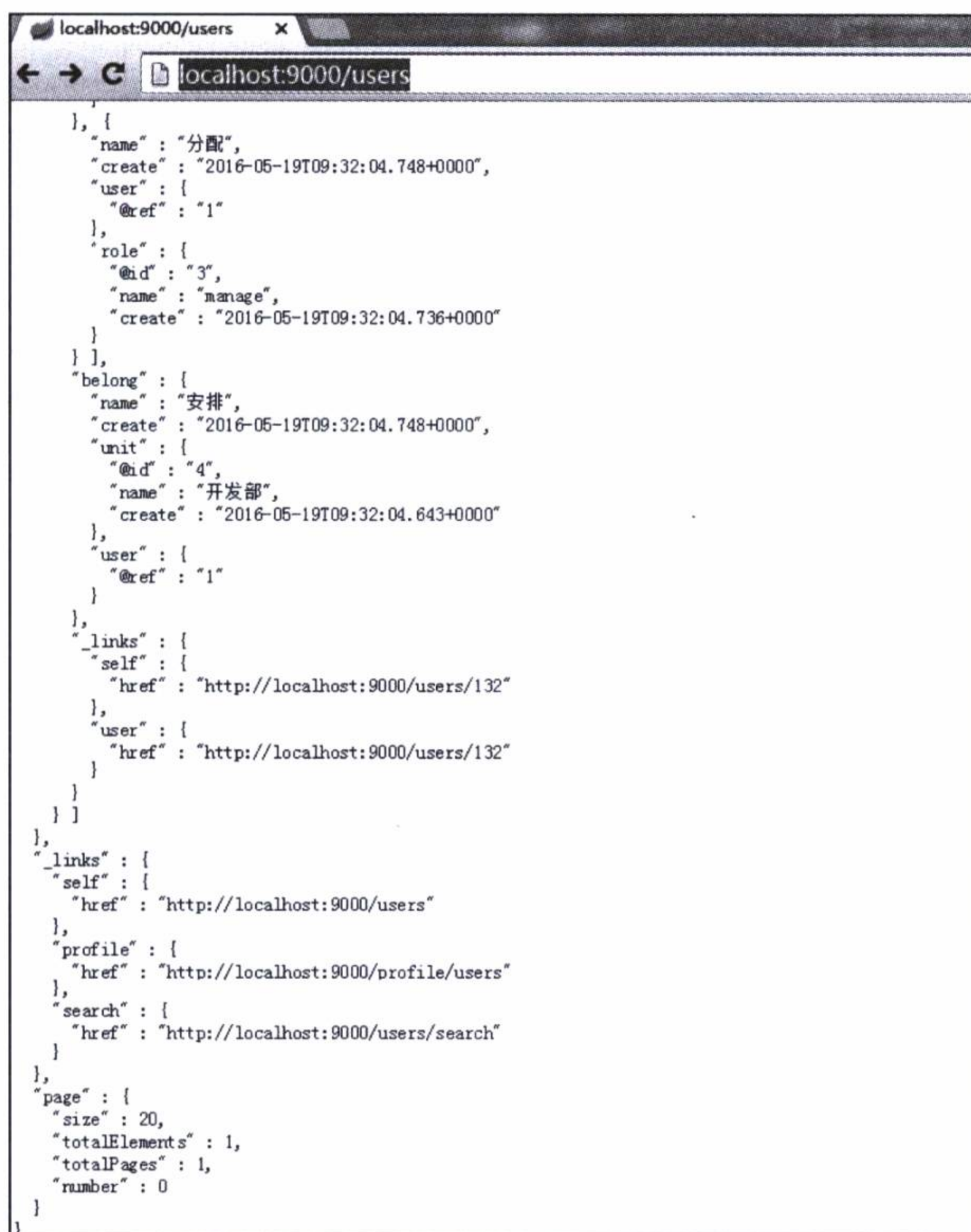
图 8-3 节点实体 User 的 REST 资源
