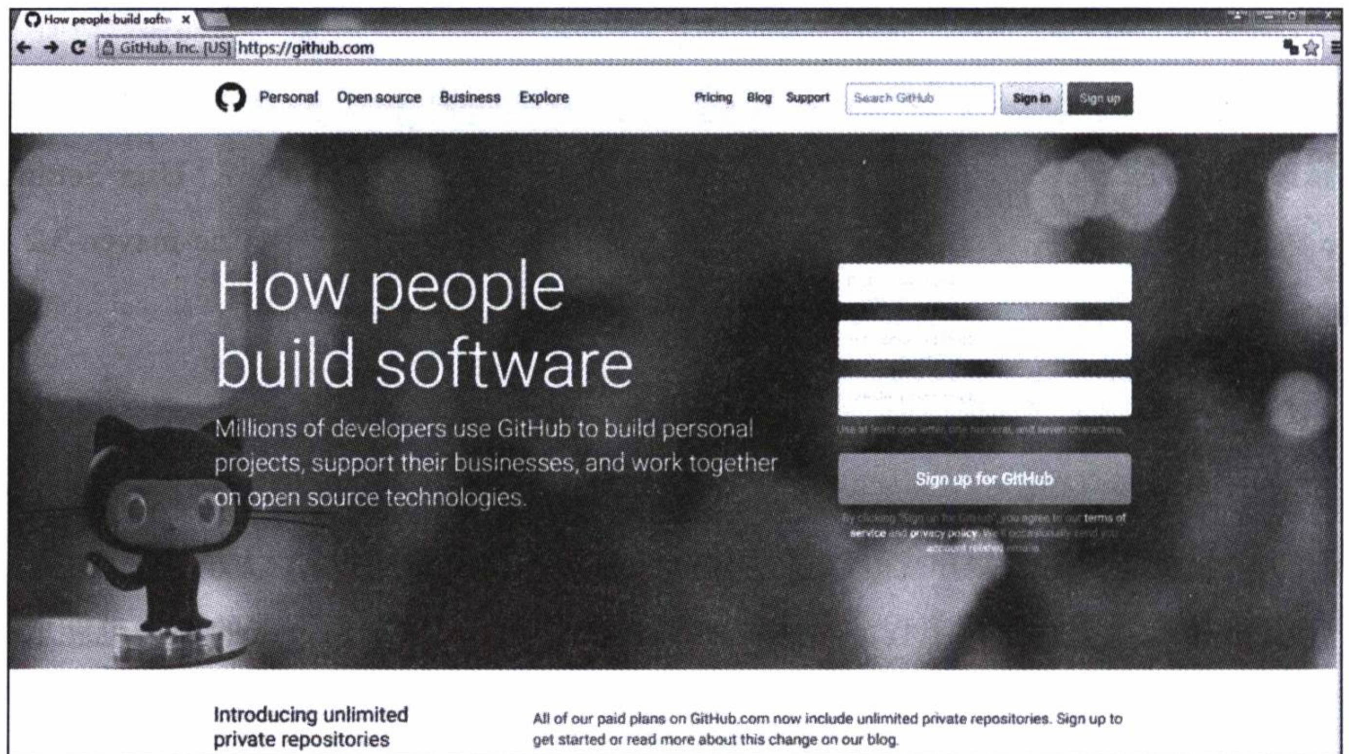
图 1-3 GitHub 首页
