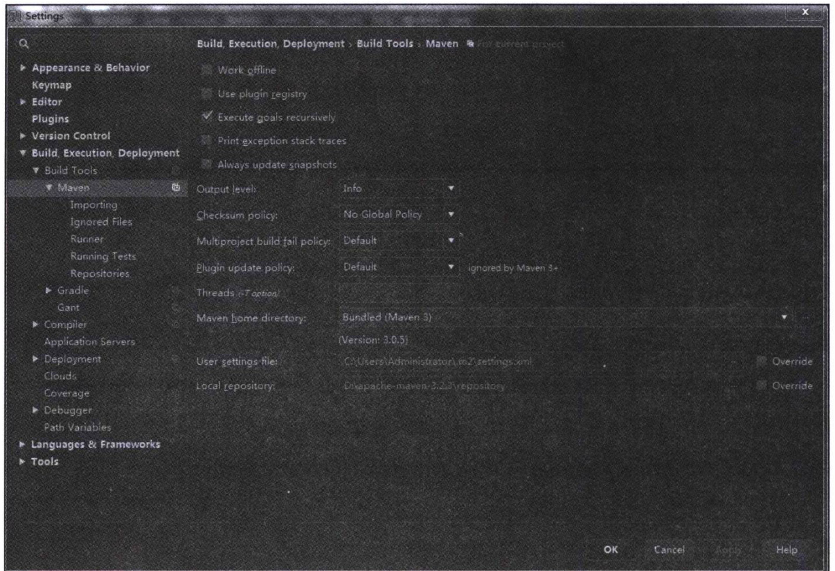
图 1-2 Maven 设置
