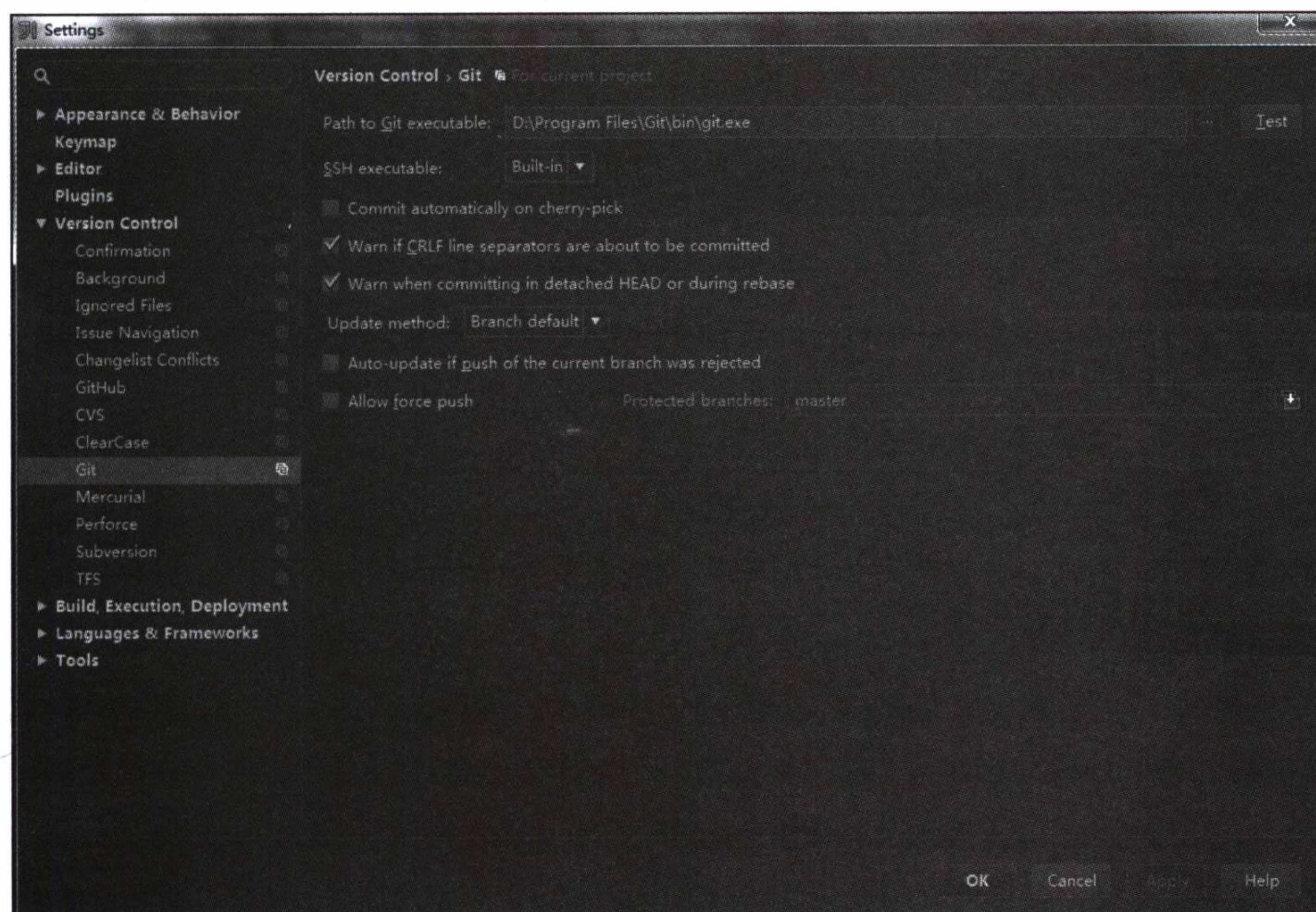
图 1-4 Git 设置
