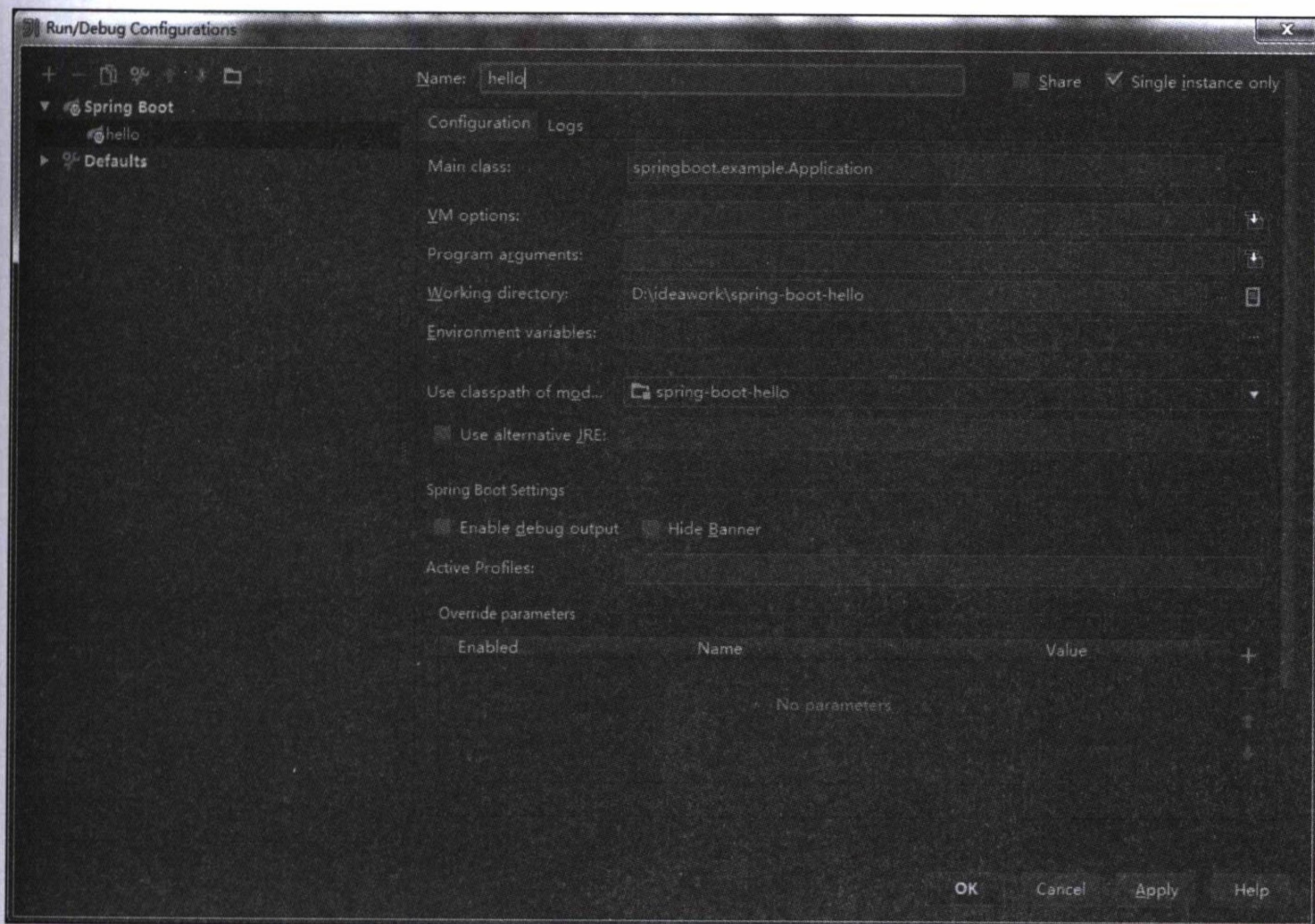
图 1-16 Spring Boot 应用配置
