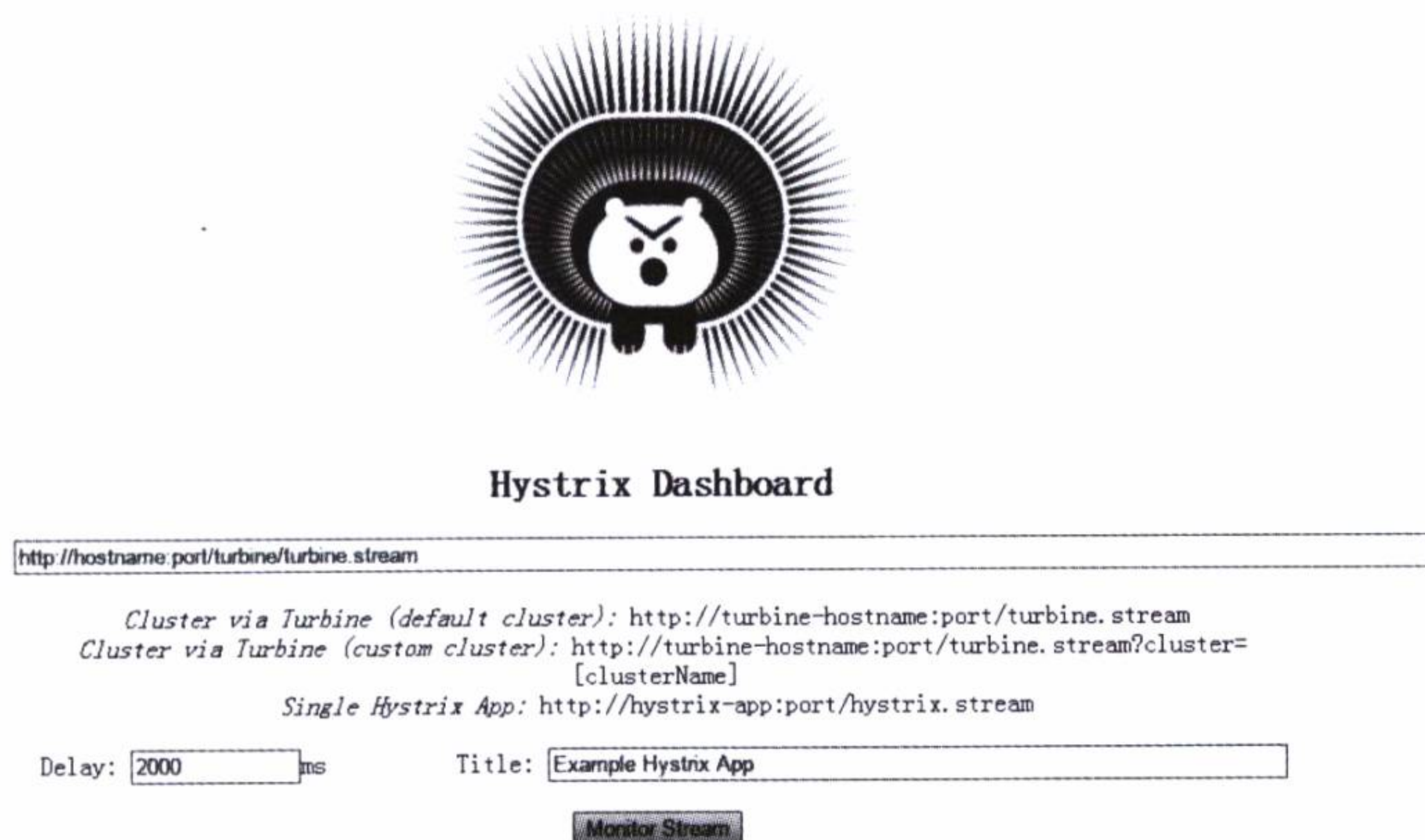
图 8-7 监控服务器首页
