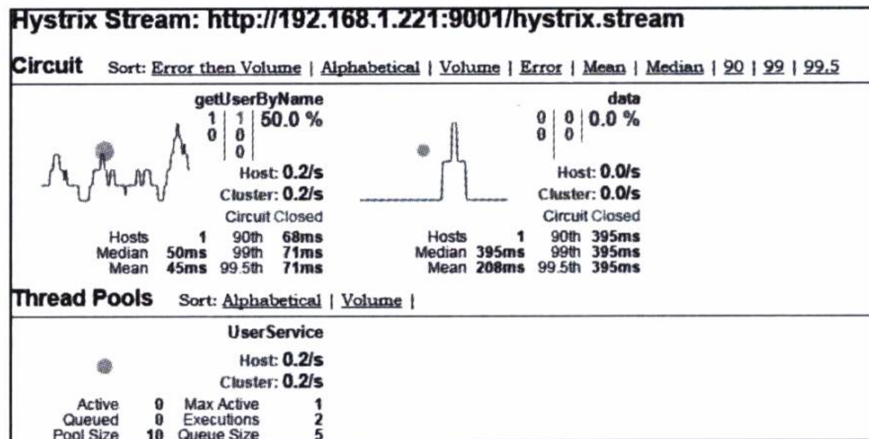
图 9-3 监控服务器中显示出现故障的情况
