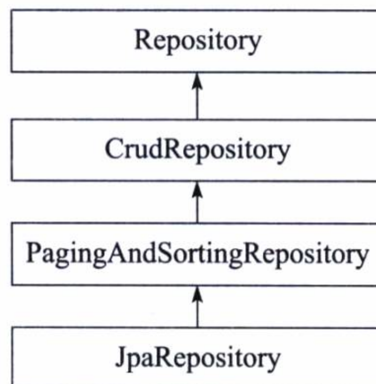
图 2-2 JpaRepository 接口继承关系
