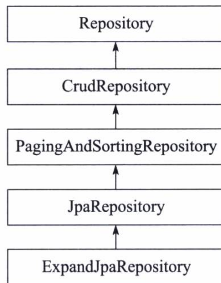
图 4-3 扩展 JPA 接口的继承关系
