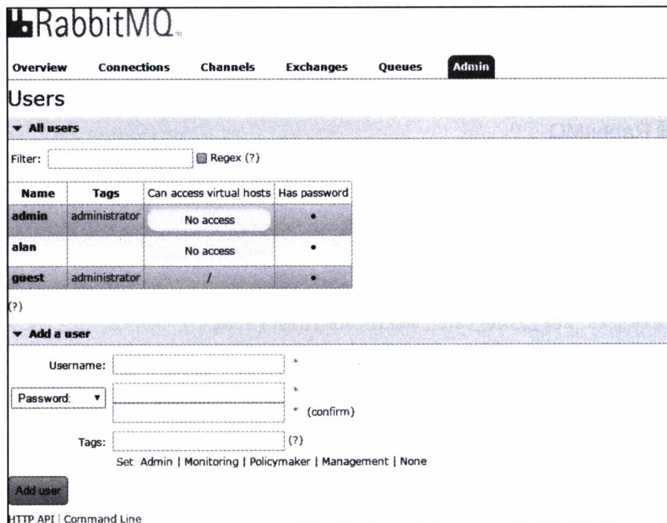
图 D-2 新增加的用户 alan
