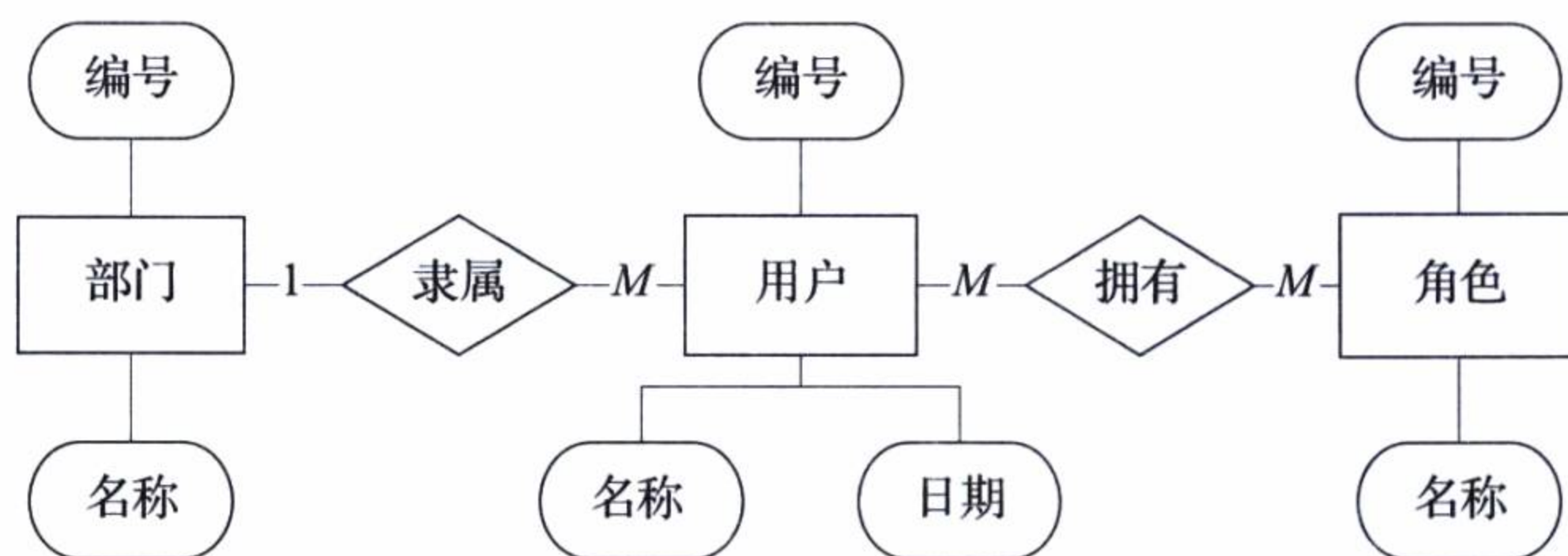
图 4-4 实体 - 关系模型设计
