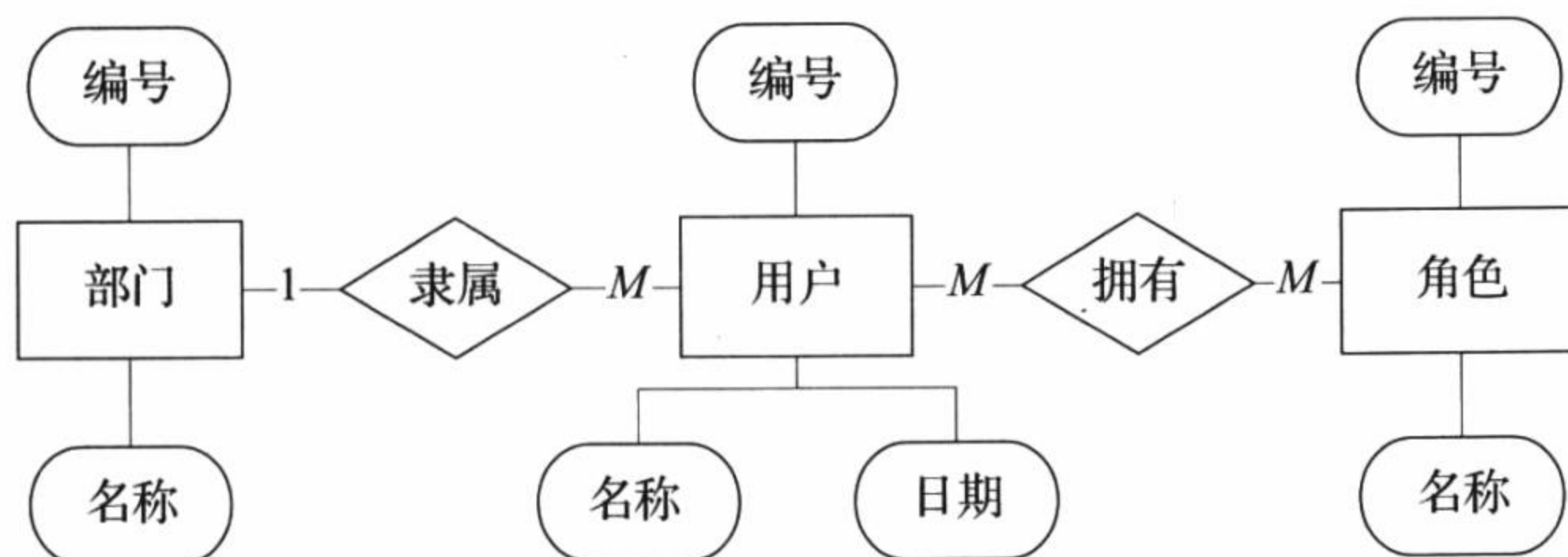
图 2-1 MySQL 实体 - 关系模型示例
