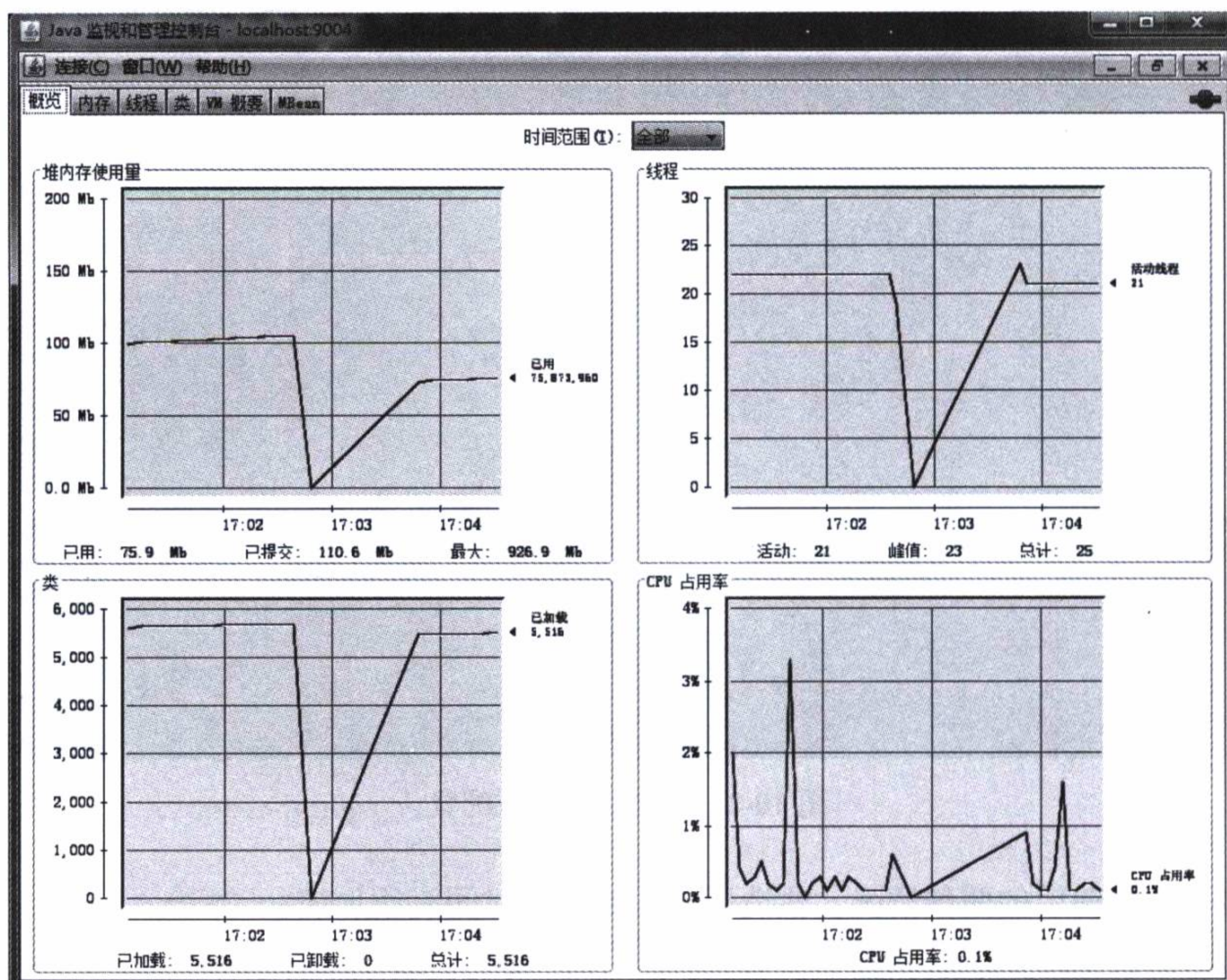
图 10-4 改造前后的两种运行情况对照图
