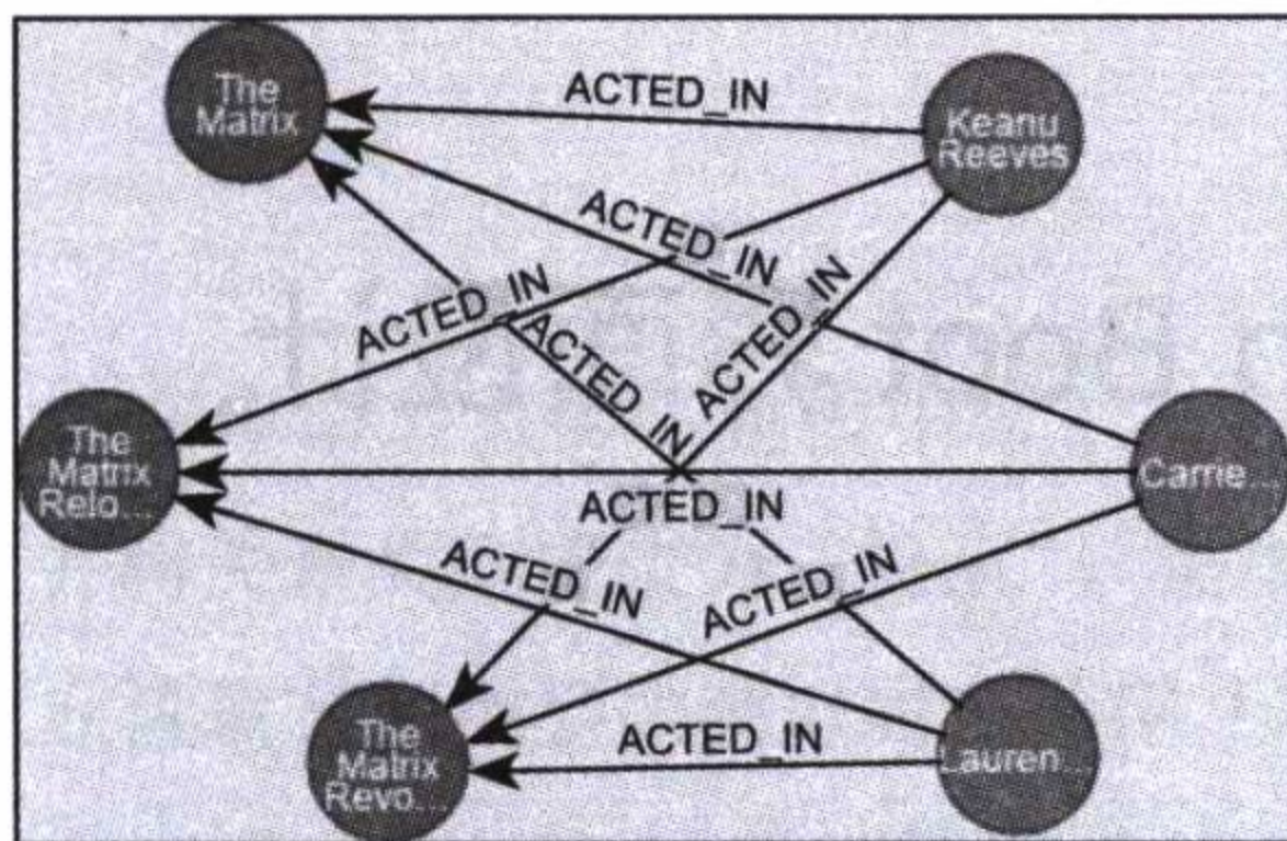
图 2-7 演员和电影的角色关系图
