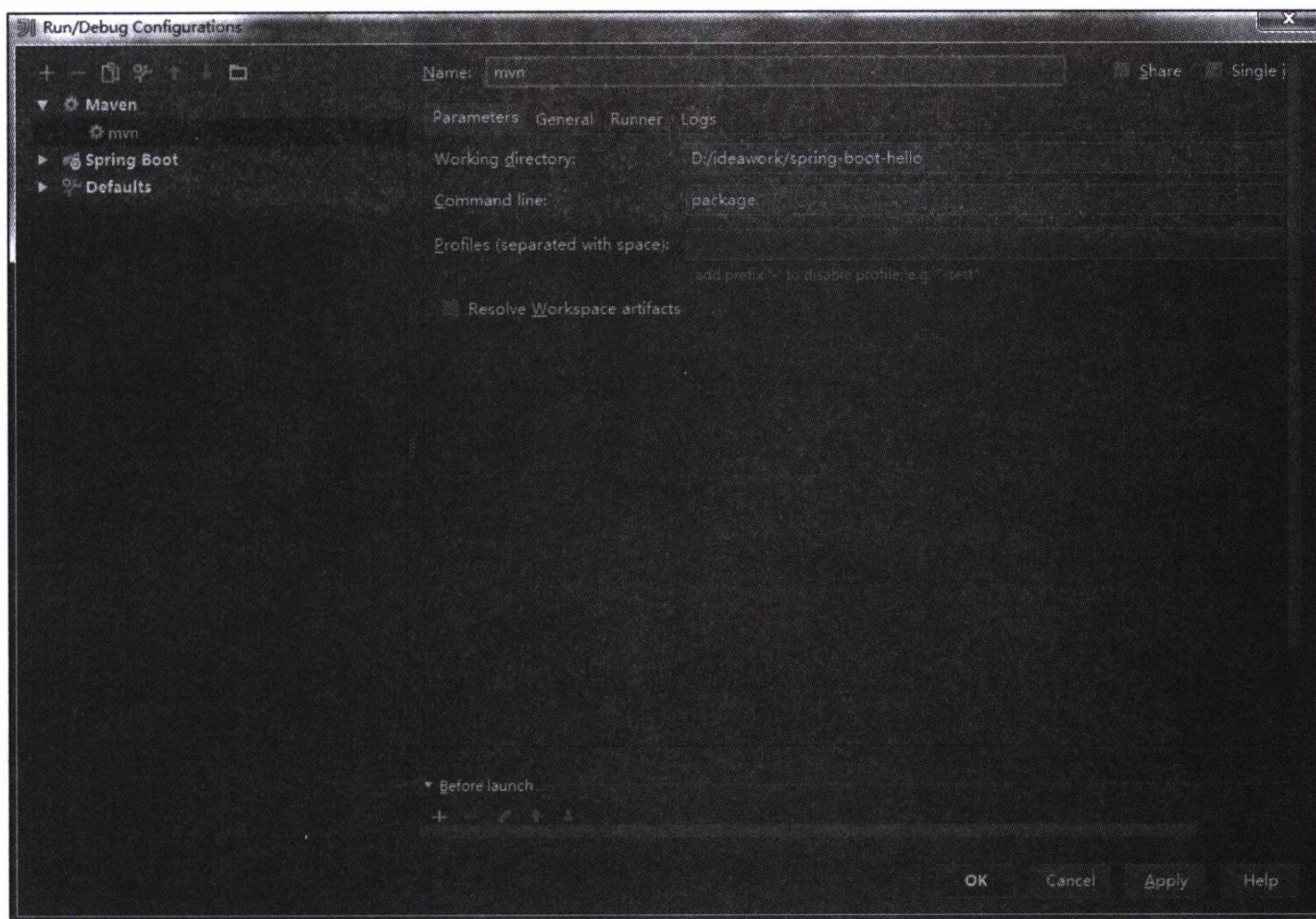
图 1-17 Maven 打包配置
