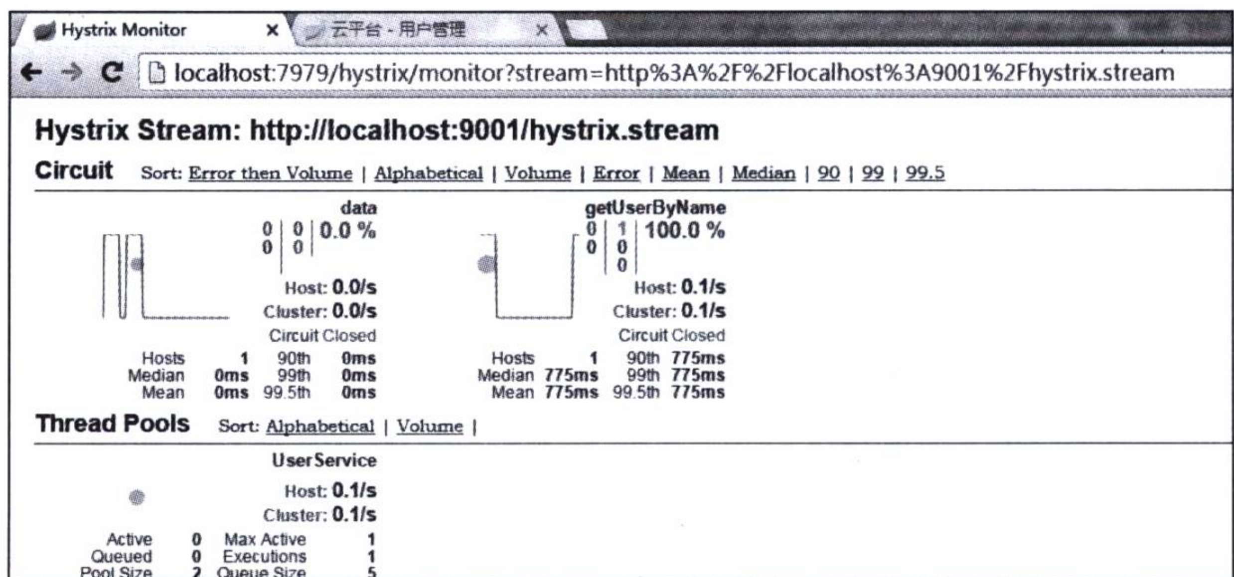
图 8-9 监控中 web 服务的异常情况
