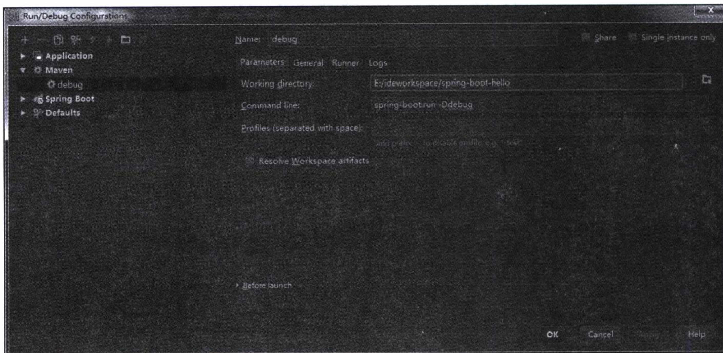
图 10-1 使用 Maven 调试的配置
