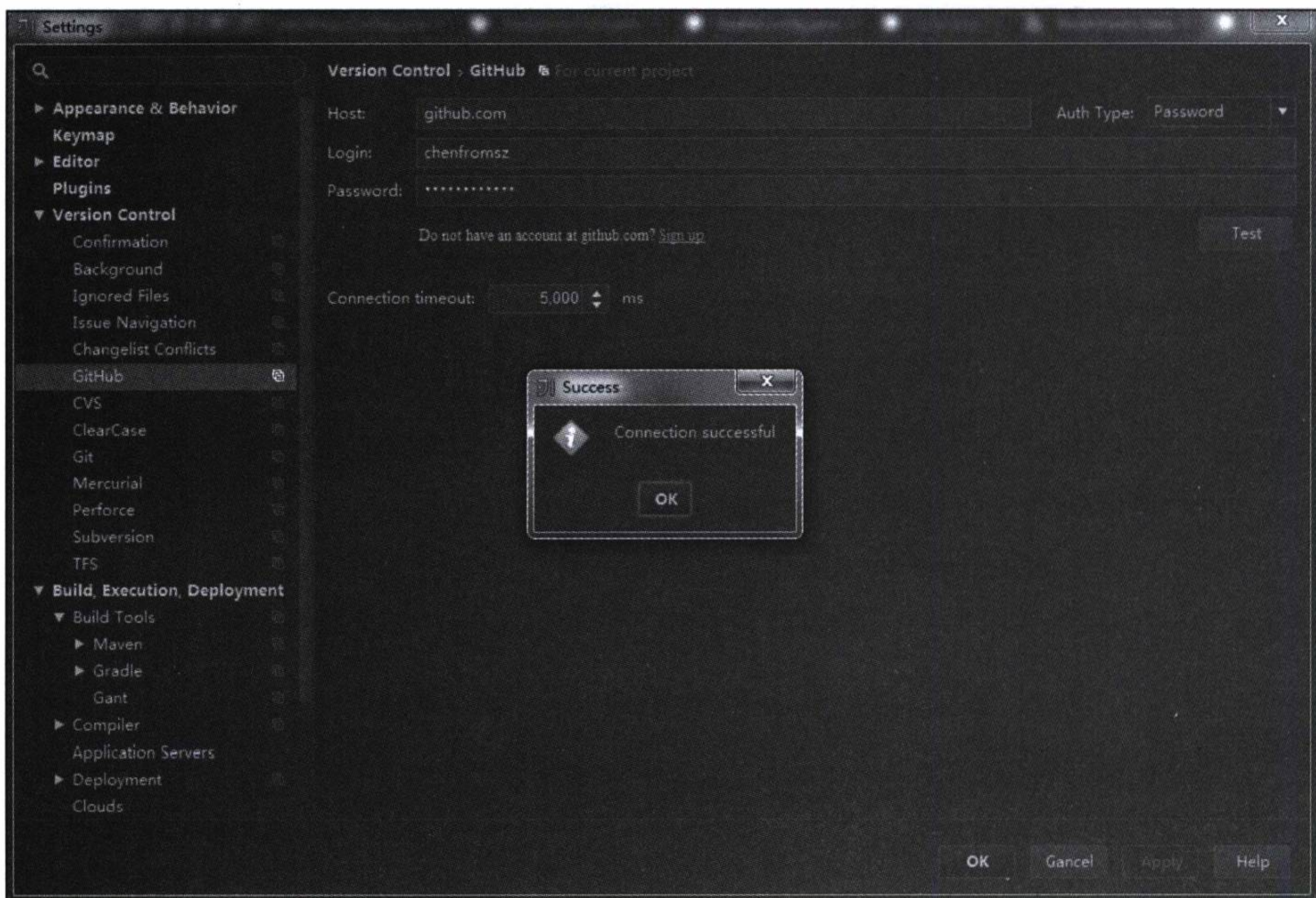
图 1-5 GitHub 配置
