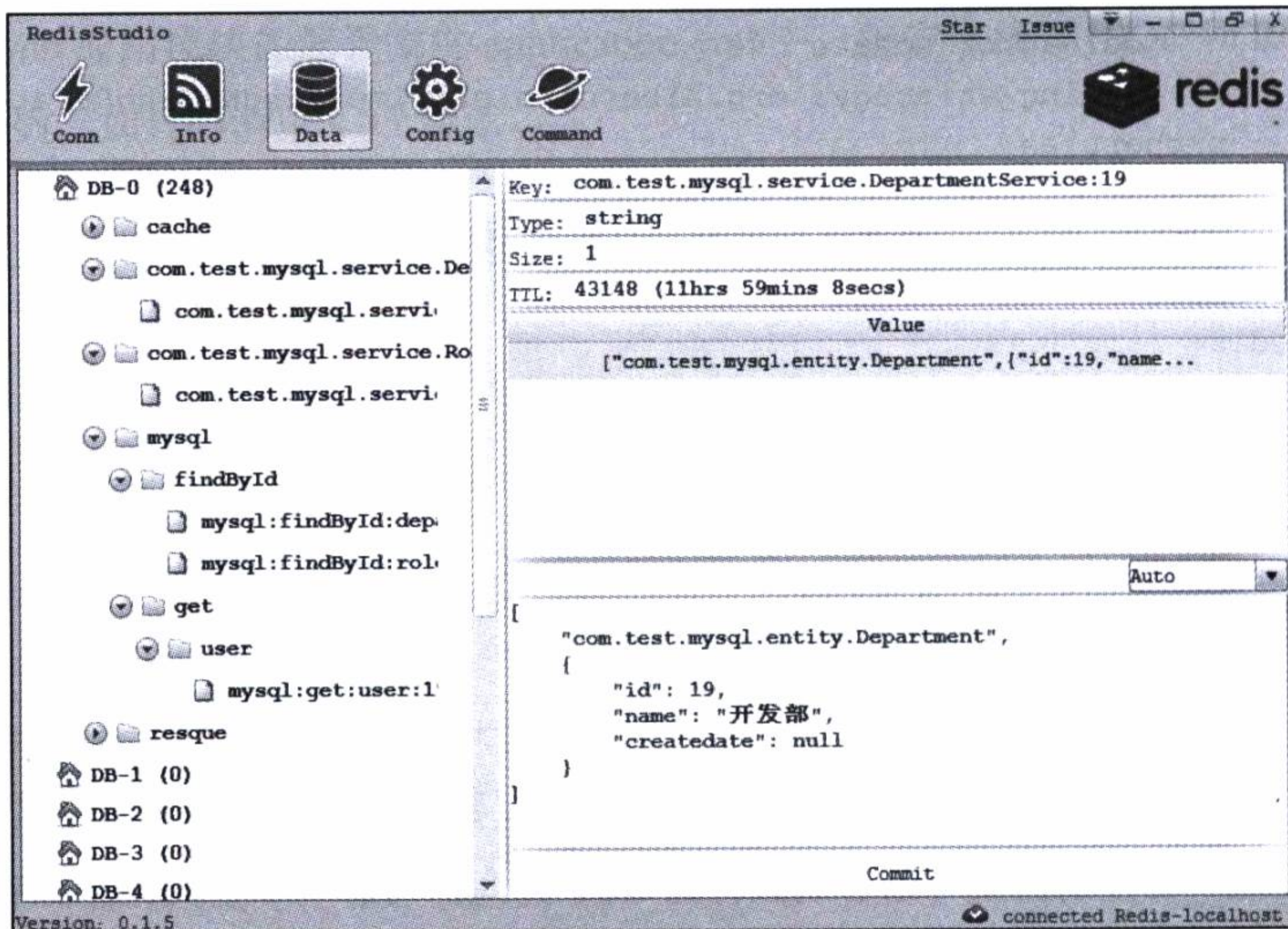
图 4-6 Redis 客户端
