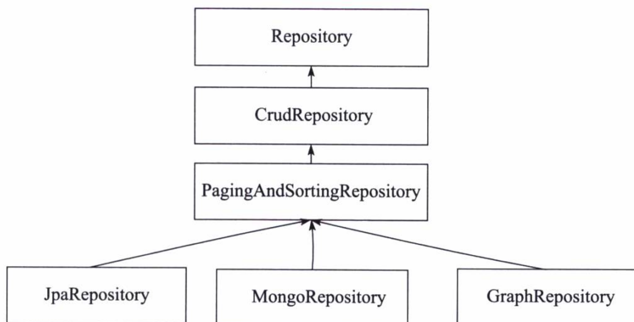
图 11-1 数据库资源库接口的继承关系
