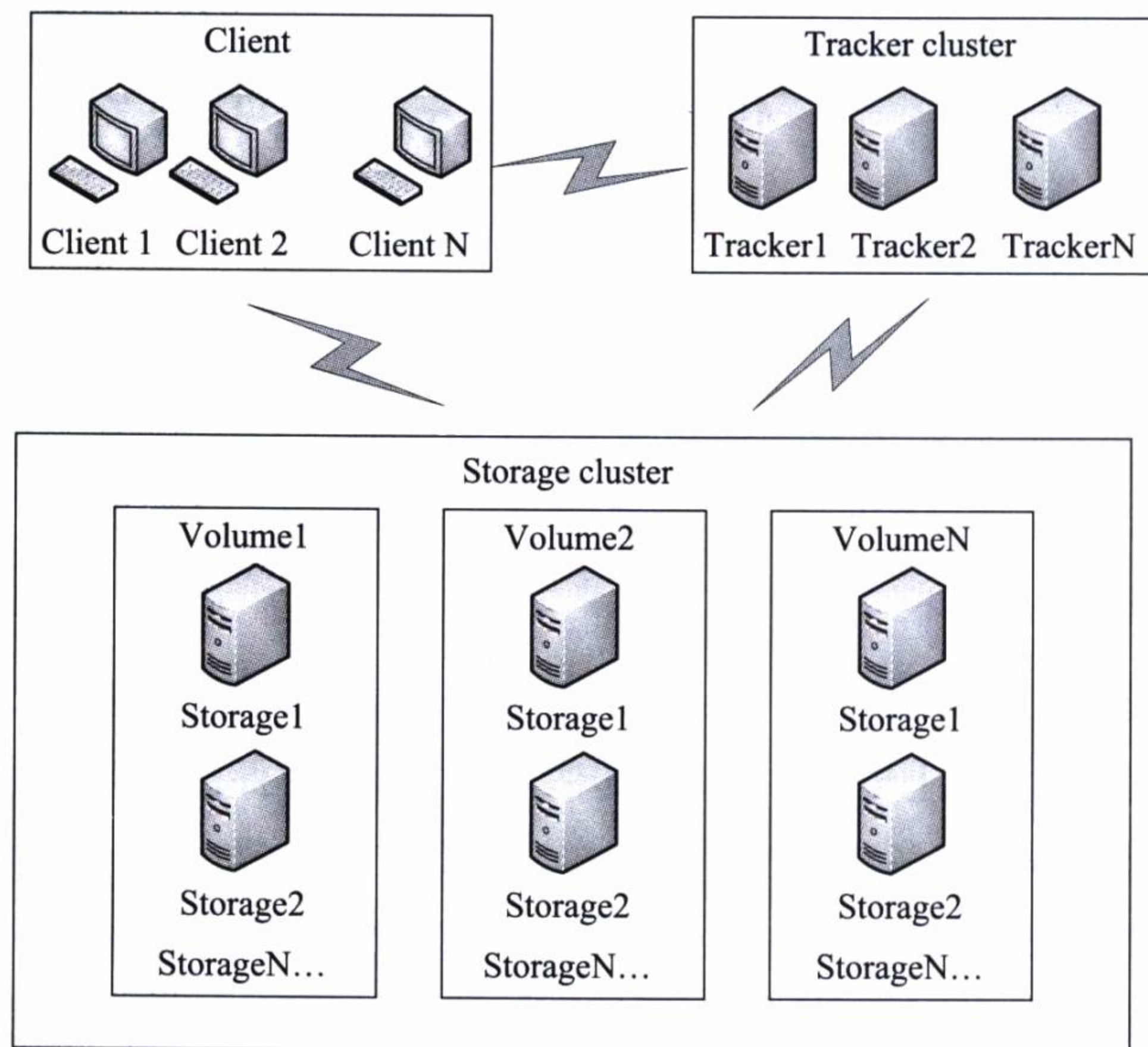
图 7-1 FastDFS 服务器网络拓扑
