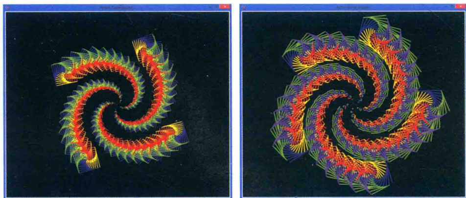
图 4-7 由（在每个拐角处的）正方形螺旋线组成的一个正方形螺旋线（左图）和由五边形螺旋线组成的一个五边形螺旋线（右图）都是由 ViralSpiral.py 程序生成的
