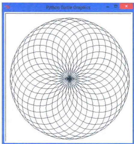
图 4-3 30 个圆组成的用户定义的玫瑰花瓣
