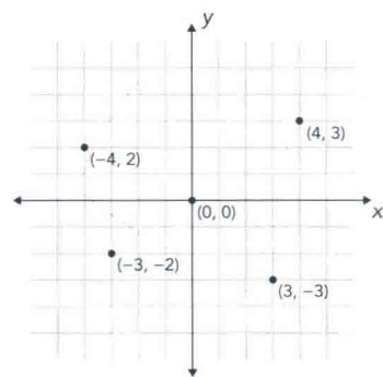
图 6-3 4 个点及其笛卡尔坐标的一幅图
