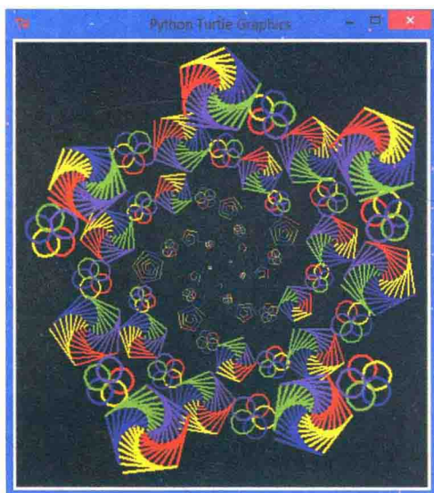
图5-1 通过一条if语句实现的由玫瑰花瓣和小螺旋线组成的螺旋线
