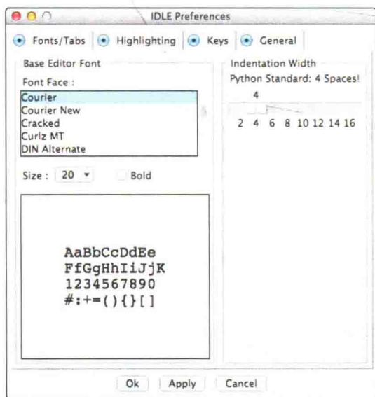
图 A-22 IDLE 中的配置选项
