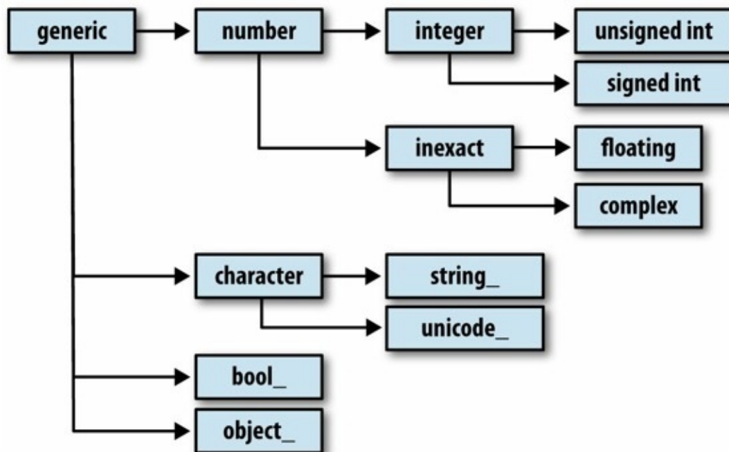
图A-2 NumPy的dtype体系
