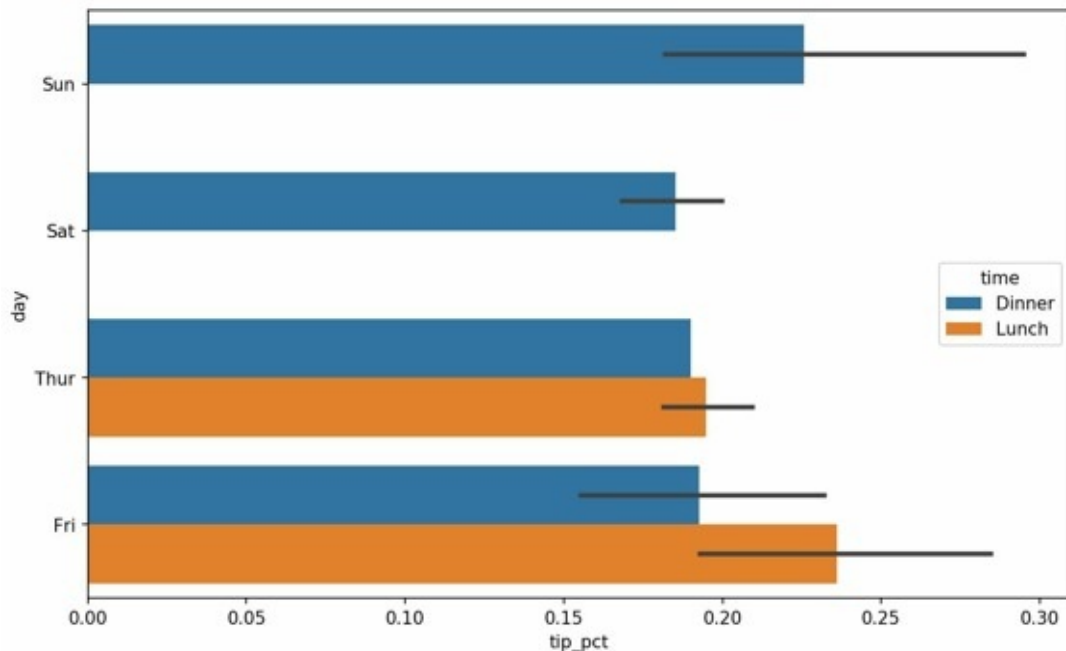
图9-20 根据天和时间的的小费比例
