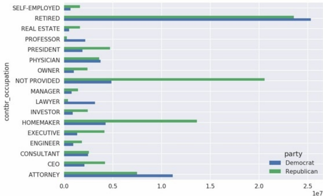
图14-12 对各党派总出资额最高的职业
