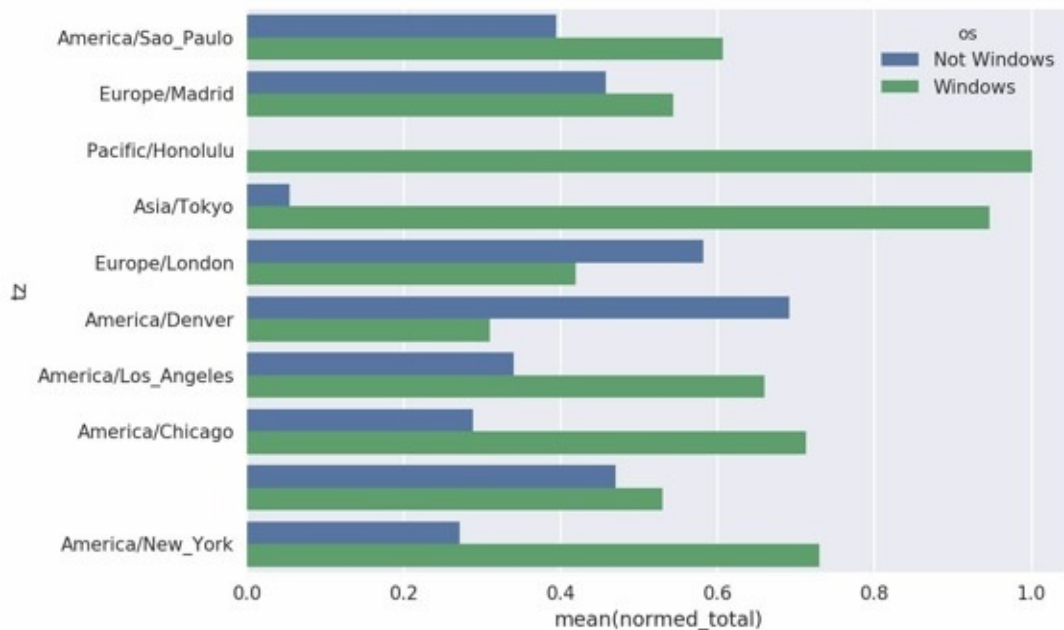
图14-3 最常出现时区的Windows和非Windows用户的百分比
