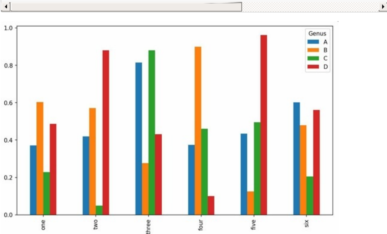
图9-16 DataFrame的柱状图
