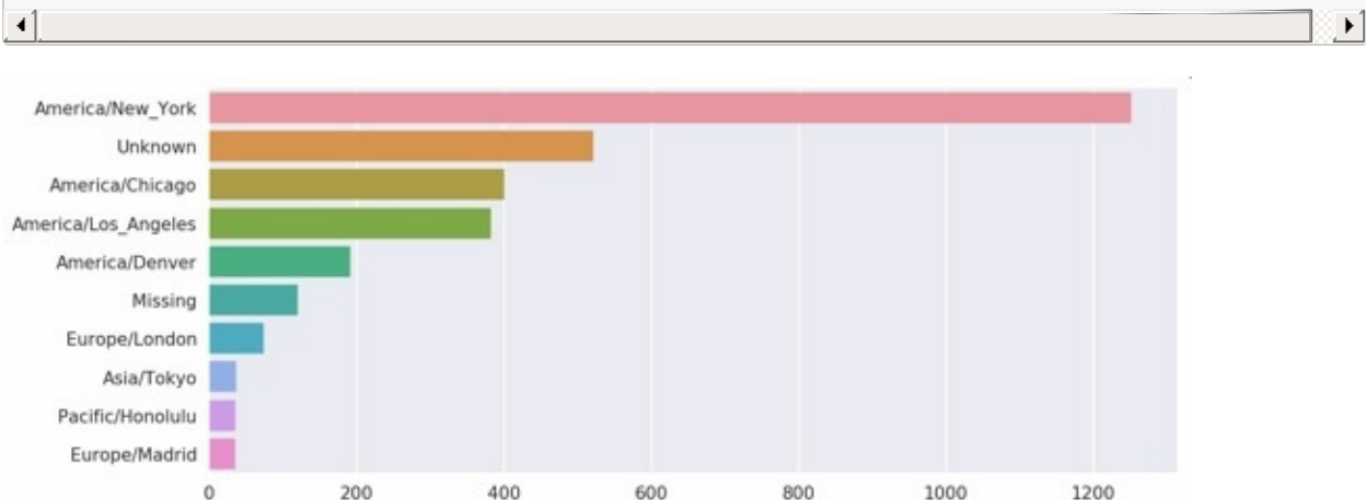
图14-1 usa.gov示例数据中最常出现的时区
