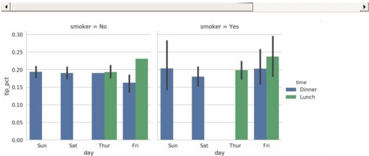
图9-26 按照天/时间/吸烟者的小费百分比
