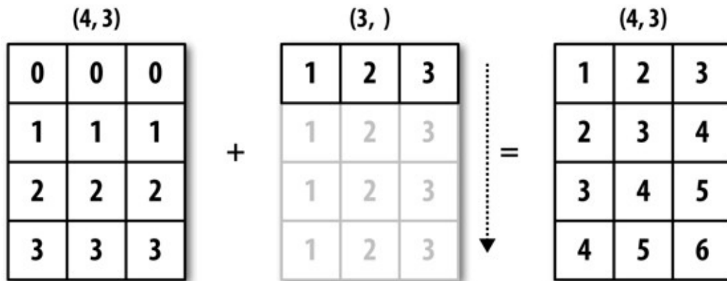
图A-4 一维数组在轴0上的广播
