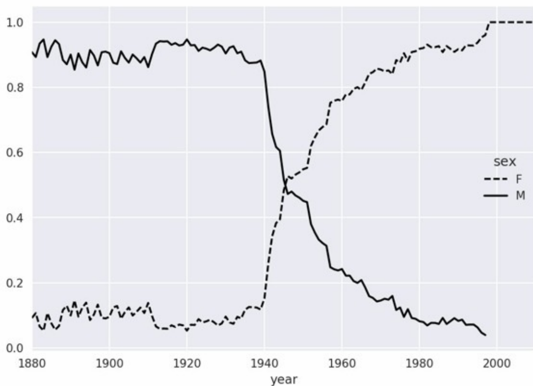
图14-10 各年度使用“Lesley型”名字的男女比例
