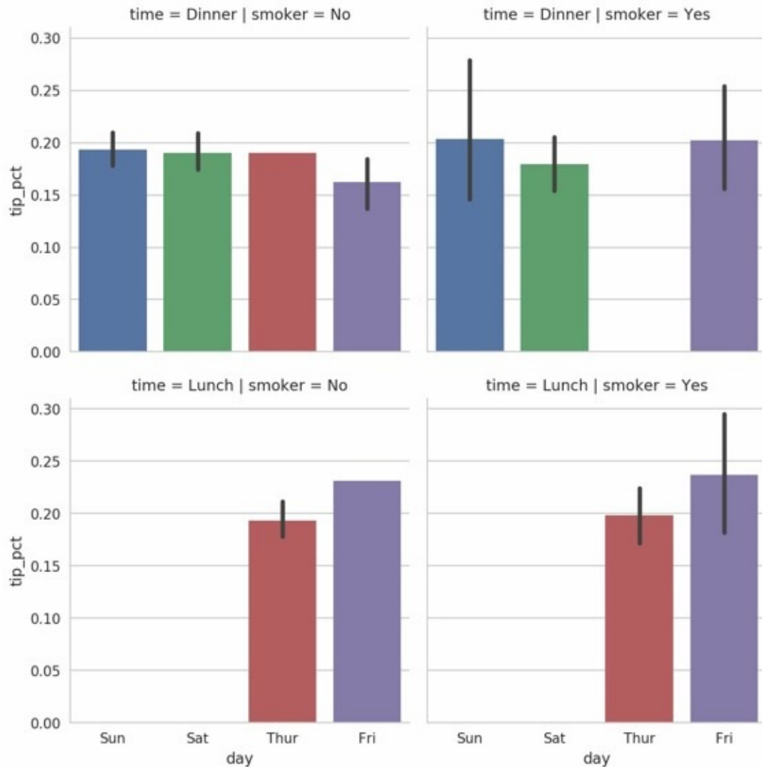
图9-27 按天的tip_pct，通过time/smoker分面
