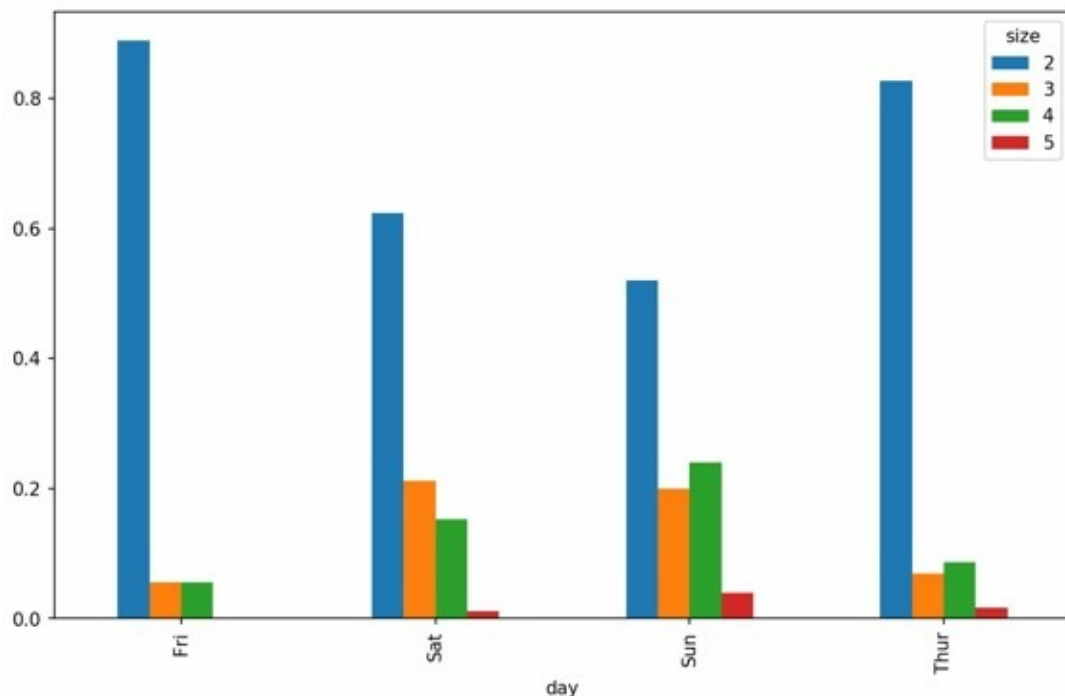
图9-18 每天各种聚会规模的比例
