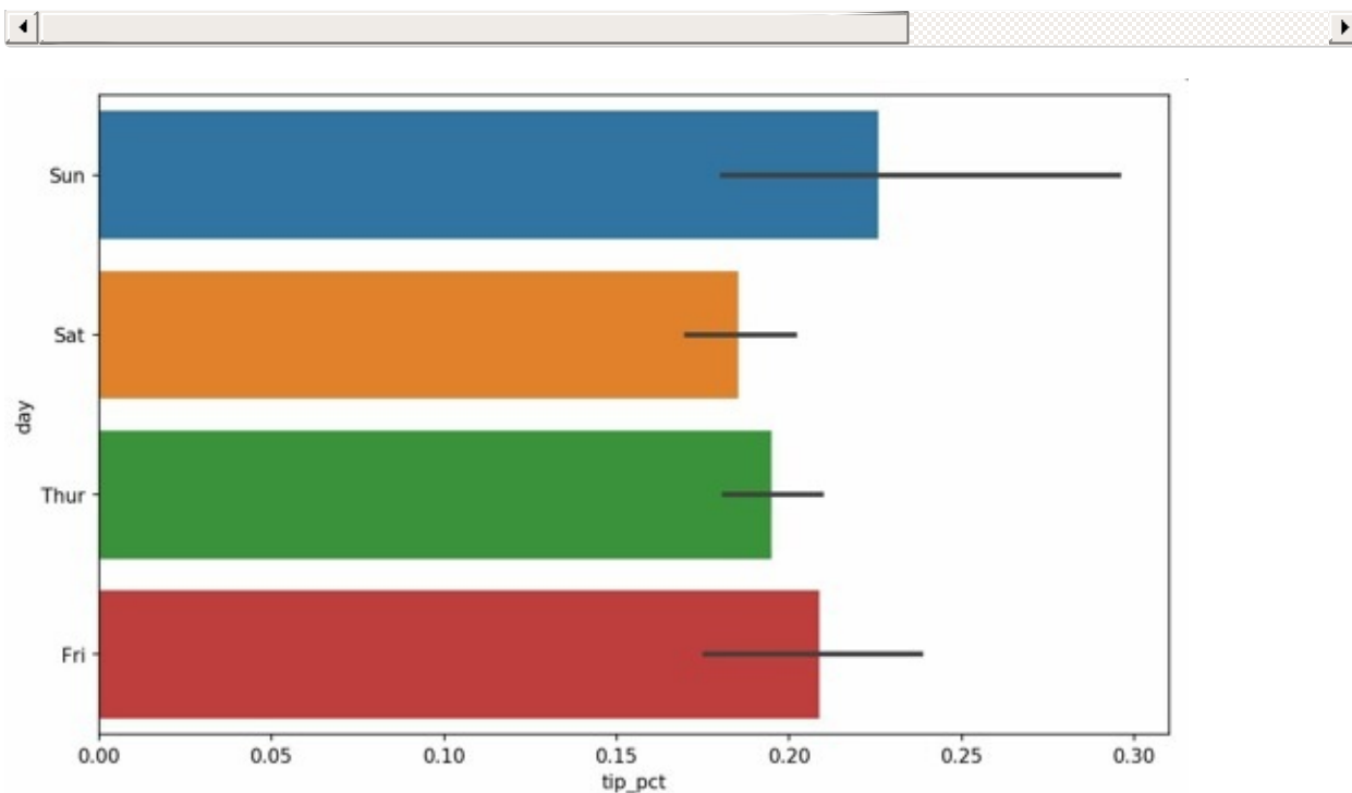
图9-19 小费的每日比例，带有误差条
