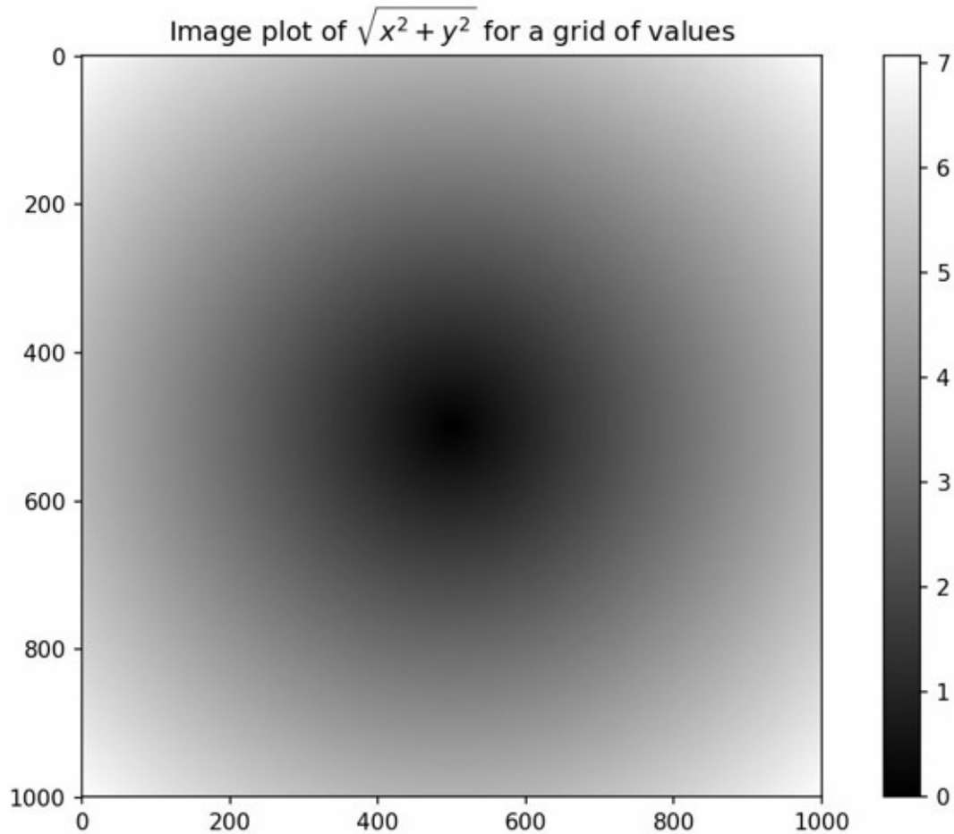
图4-3 根据网格对函数求值的结果
