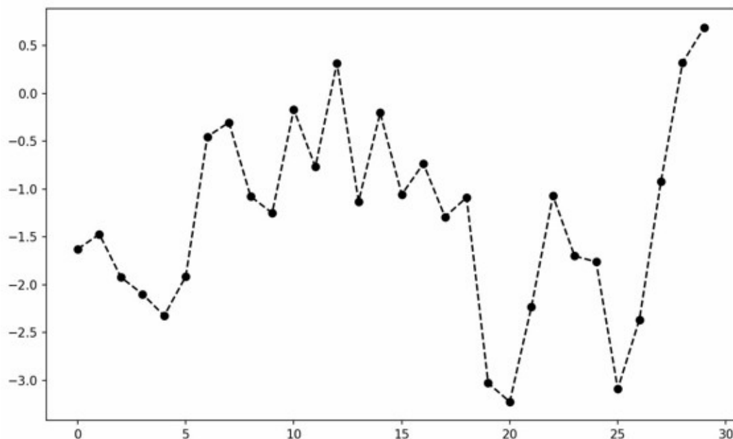
图9-6 带有标记的线型图示例
