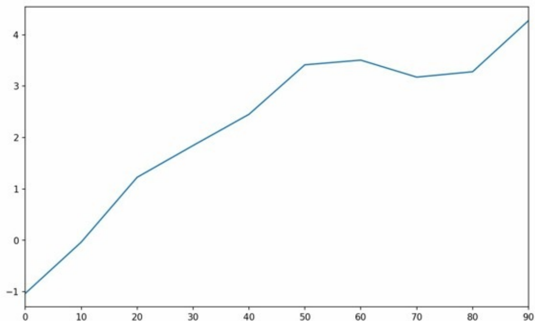
图9-13 简单的Series图表示例
