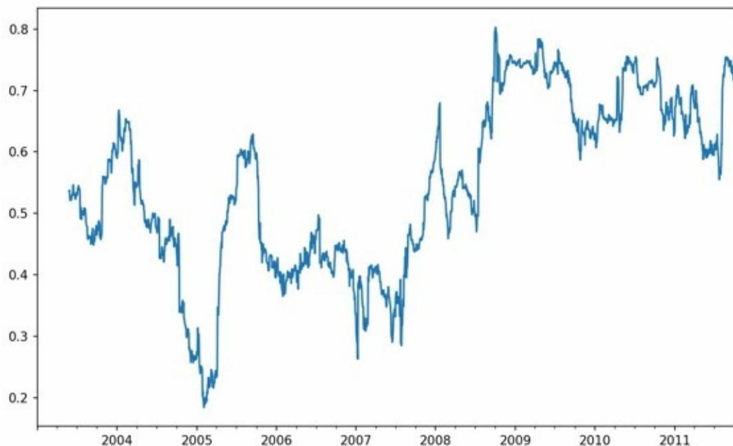
图11-8 AAPL 6个月的回报与标准普尔500指数的相关系数
