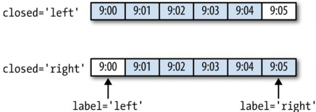
图11-3 各种closed、label约定的“5分钟”重采样演示
