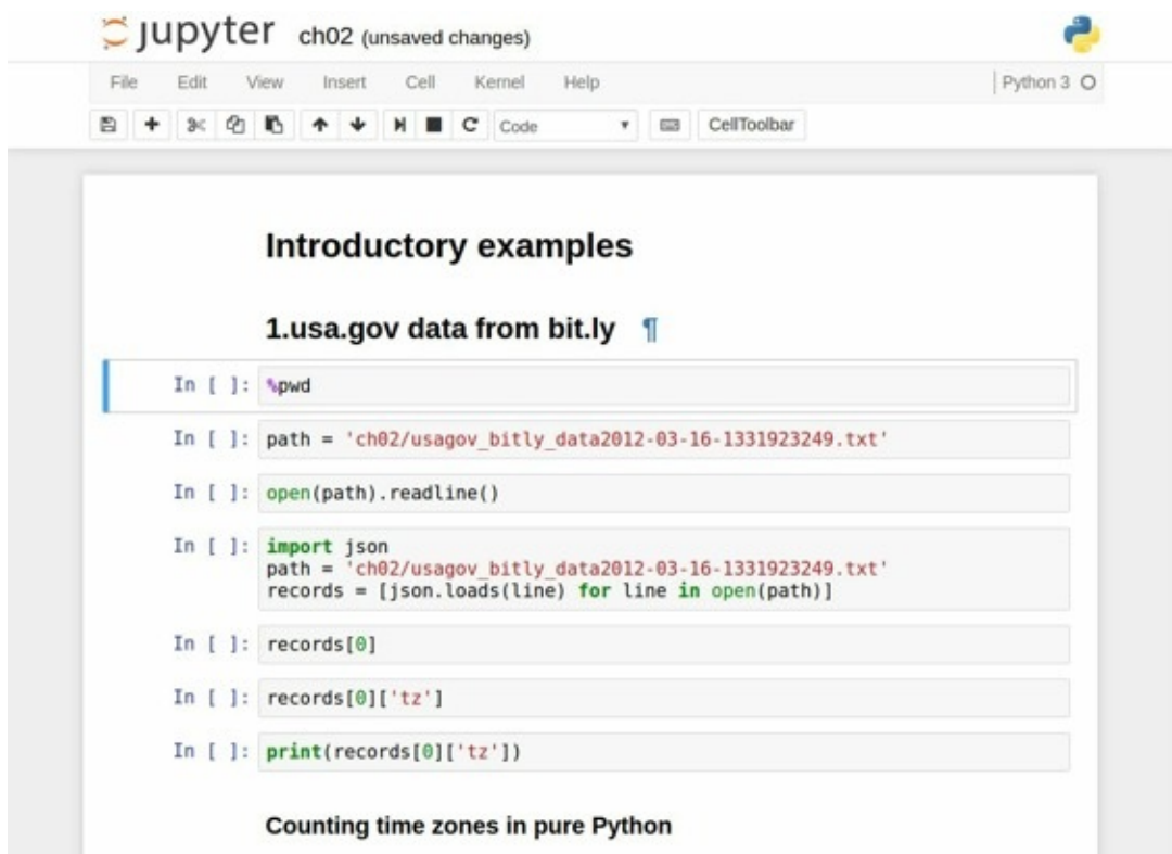
图2-3 Jupyter查看一个存在的notebook的页面
