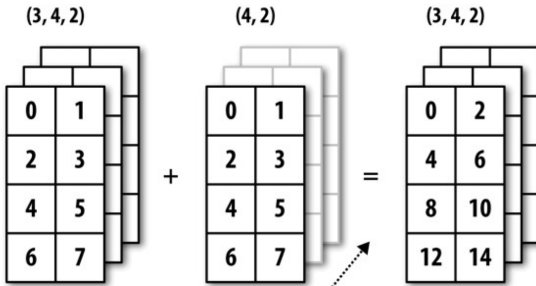
图A-6 三维数组在轴0上的广播
