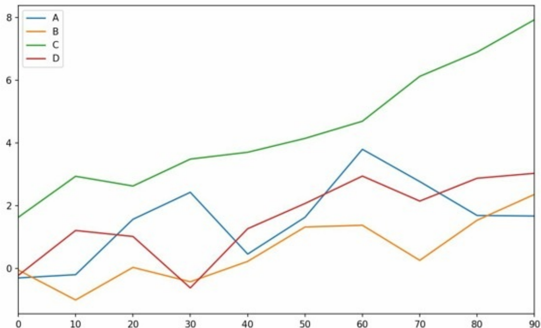
图9-14 简单的DataFrame绘图
