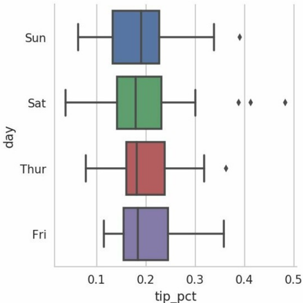
图9-28 按天的tip_pct的盒图
