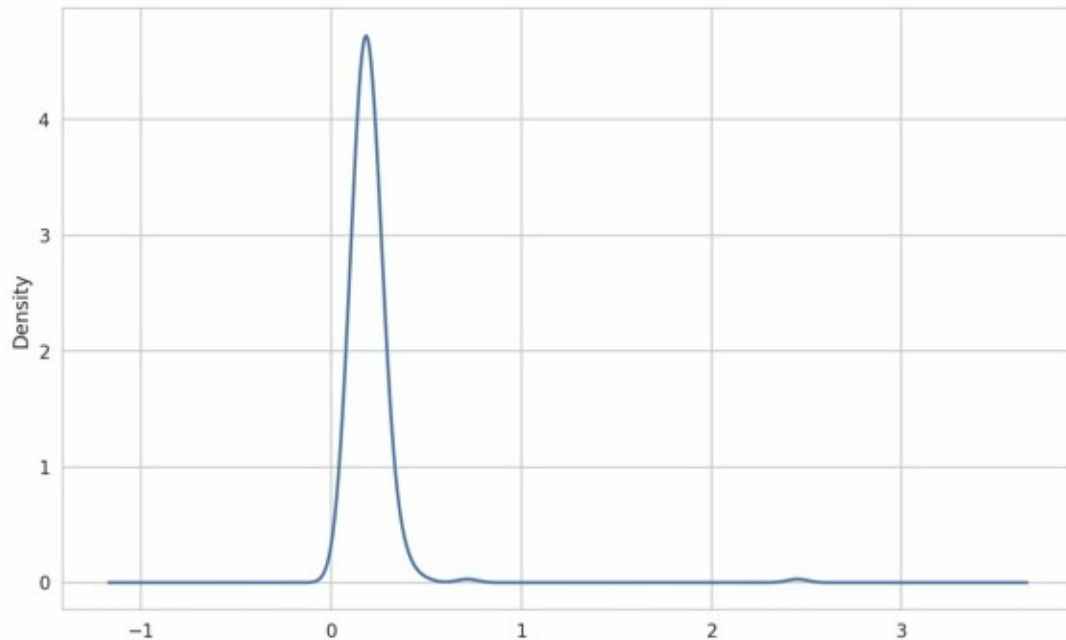
图9-22 小费百分比的密度图
