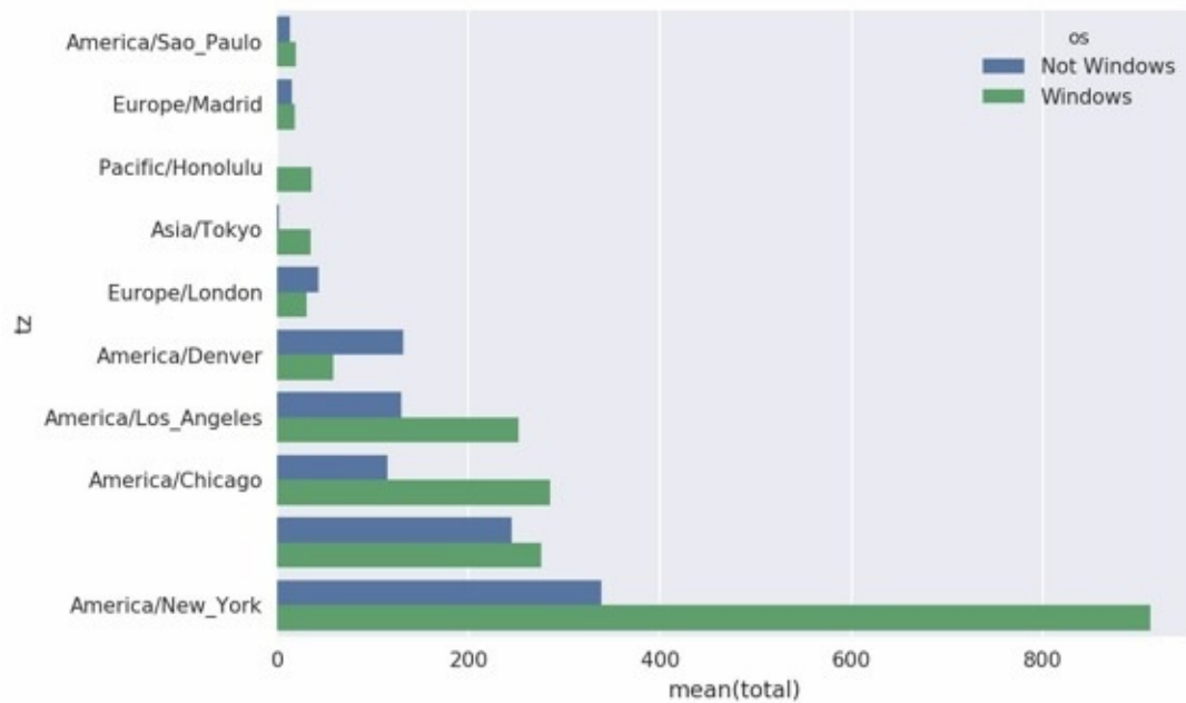
图14-2 最常出现时区的Windows和非Windows用户
