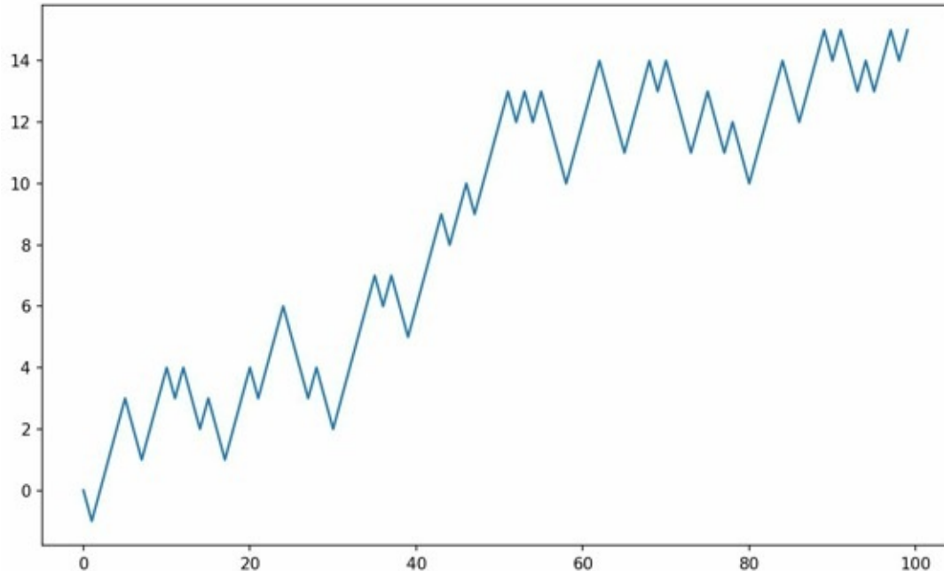
图4-4 简单的随机漫步
