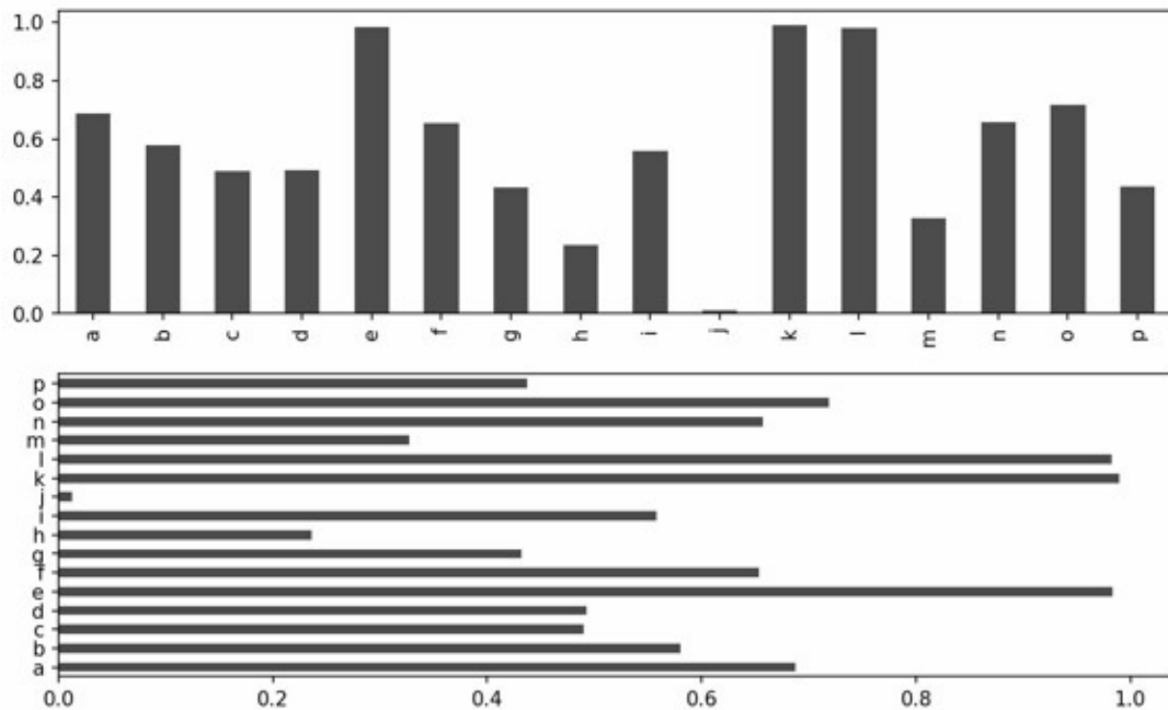
图9-15 水平和垂直的柱状图
