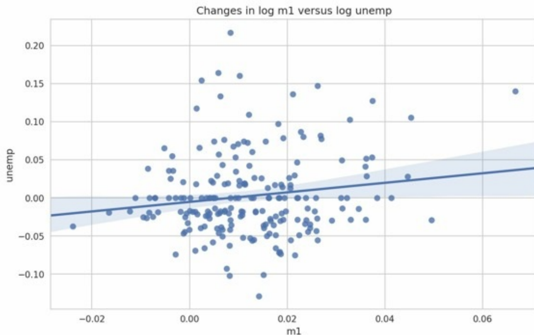
图9-24 seaborn的回归/散布图
