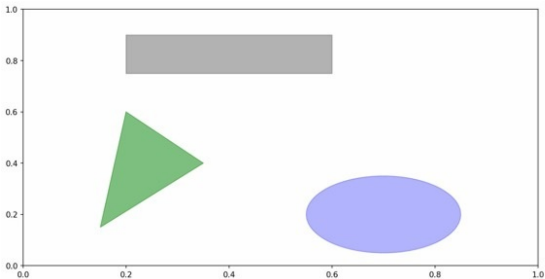
图9-12 由三个块图形组成的图
