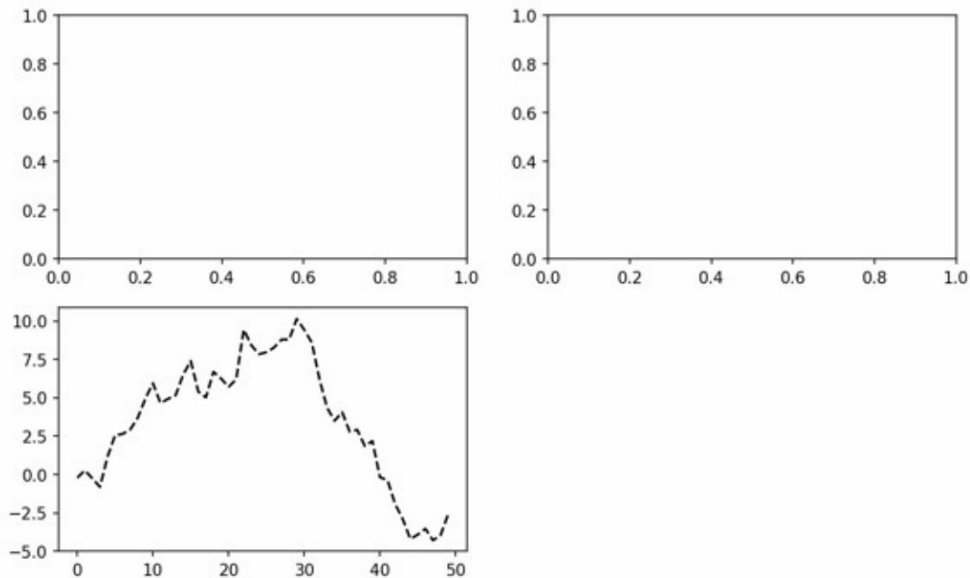
图9-3 绘制一次之后的图像
