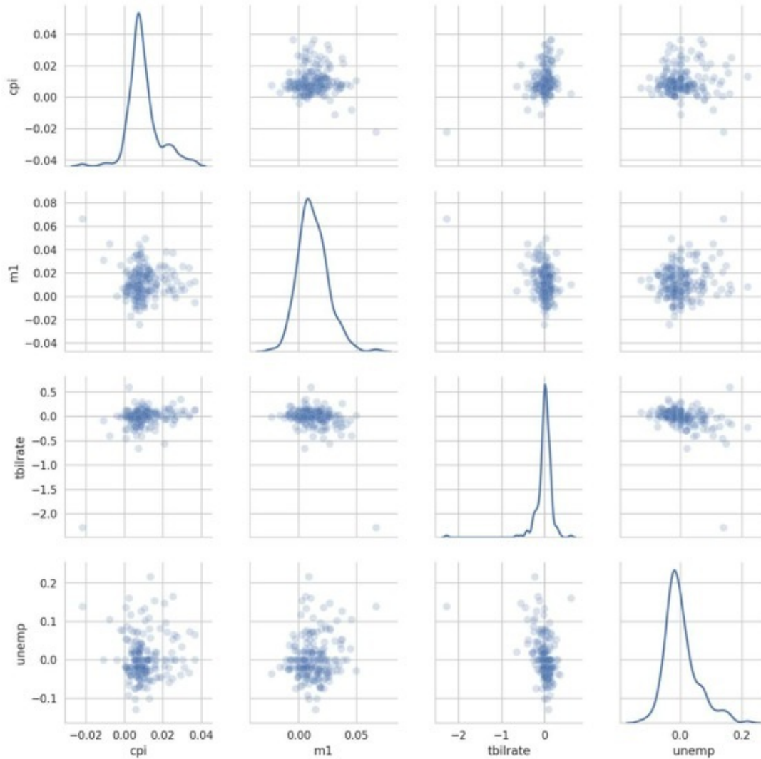
图9-25 statsmodels macro data的散布图矩阵
