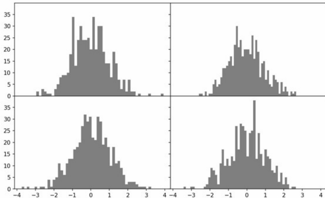
图9-5 各subplot之间没有间距
