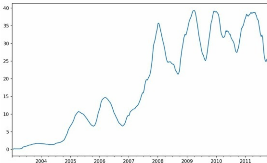
图11-5 苹果公司250日每日回报标准差
