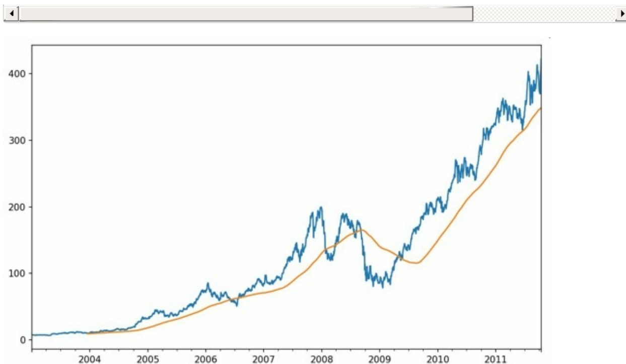
图11-4 苹果公司股价的250日均线
