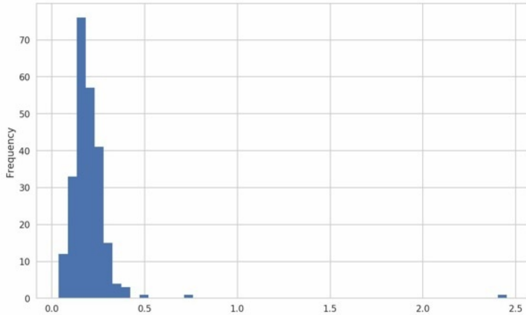
图9-21 小费百分比的直方图
