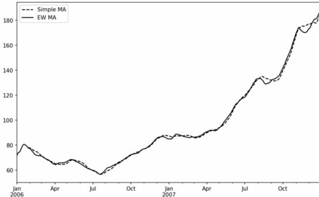
图11-7 简单移动平均与指数加权移动平均
