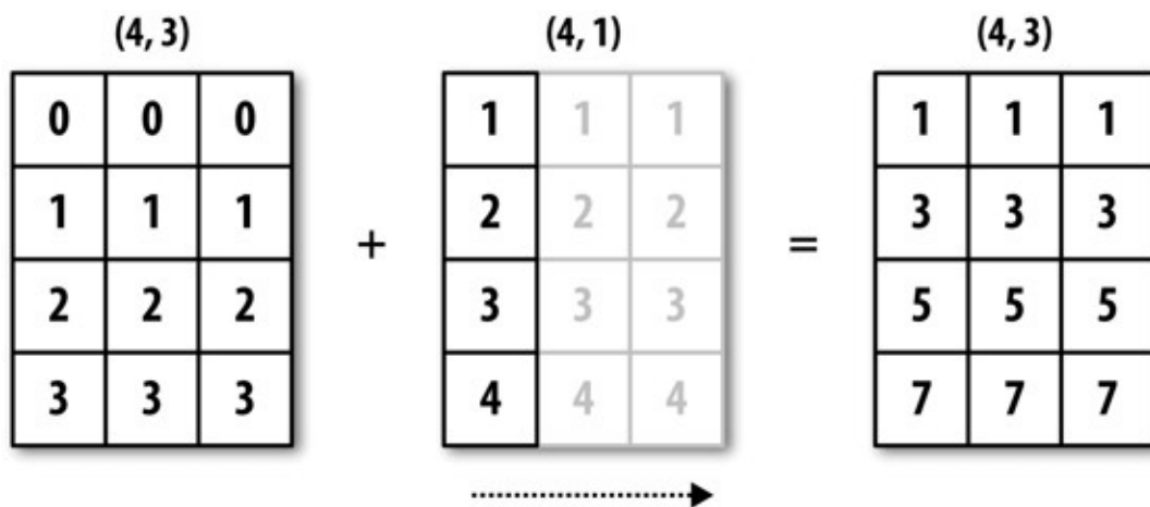
图A-5 二维数组在轴1上的广播
