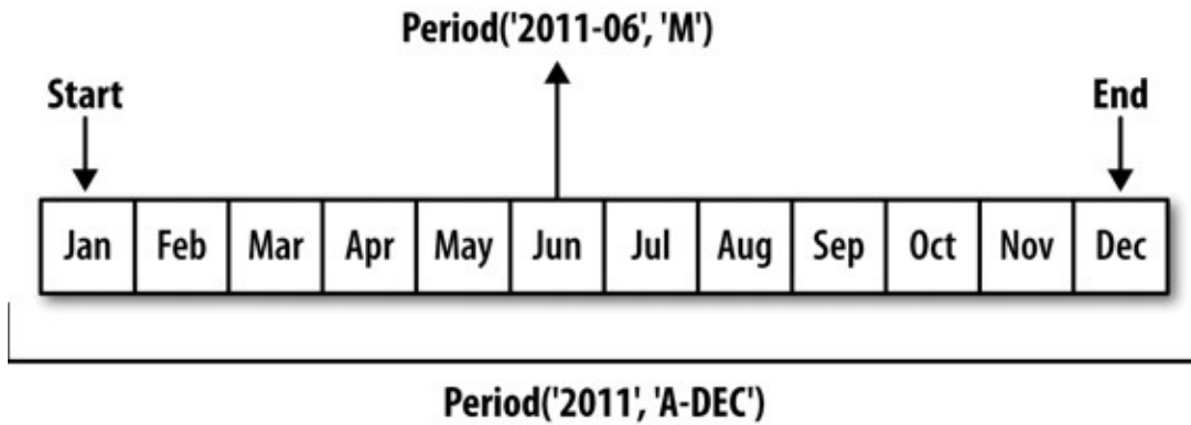
图11-1 Period频率转换示例
