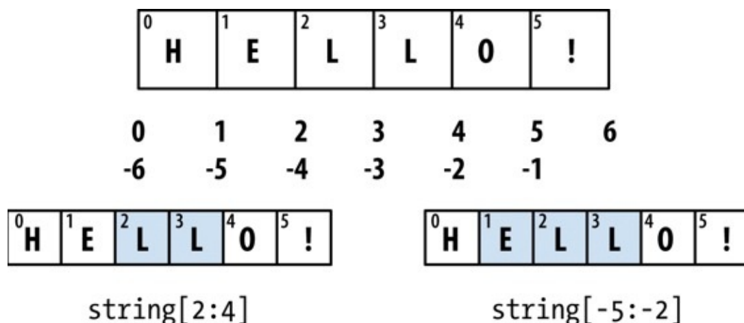
图3-1 Python切片演示
