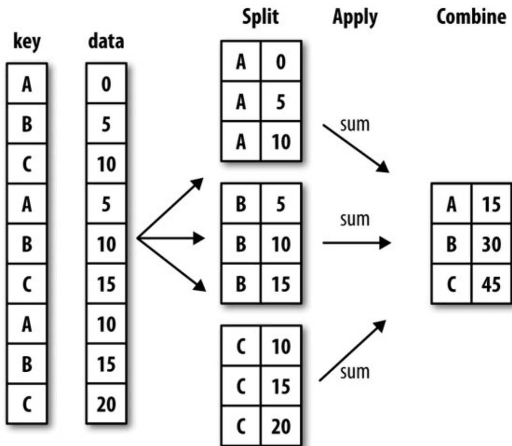
图10-1 分组聚合演示
