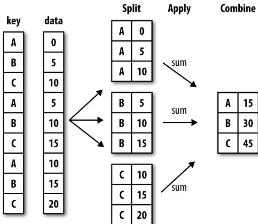
图10-2 分组聚合示例
