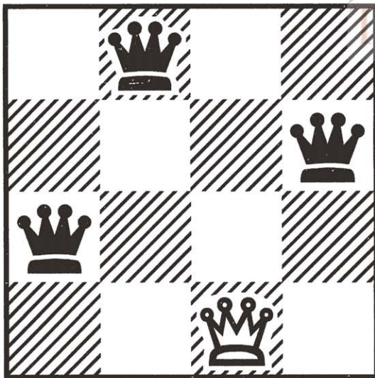
图9-1 在一个4×4的棋盘上放4个皇后
