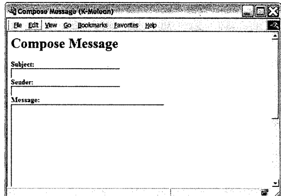
图26-3 消息撰写器
