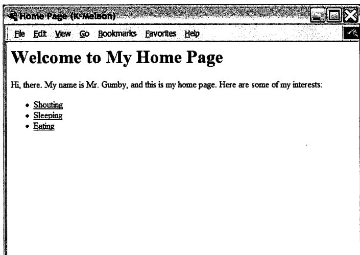
图22-1 生成的网页
