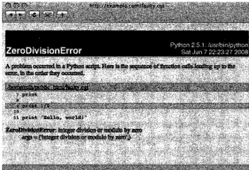
图15-1 利用cgi模块获得的回溯
