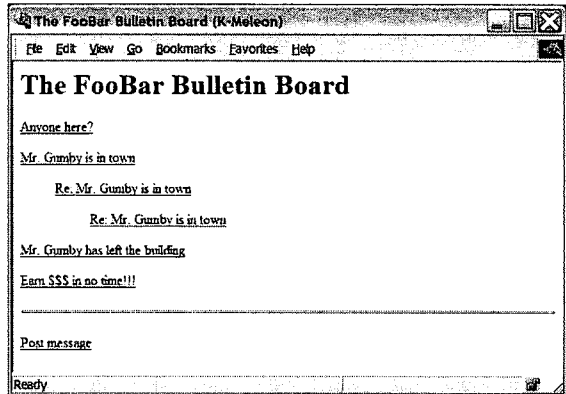
图26-1 主页
