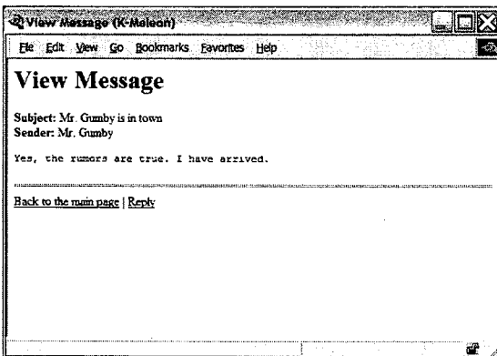
图26-2 消息查看器
