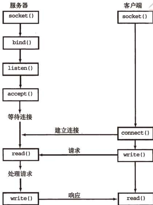
图21-1 TCP连接协议
