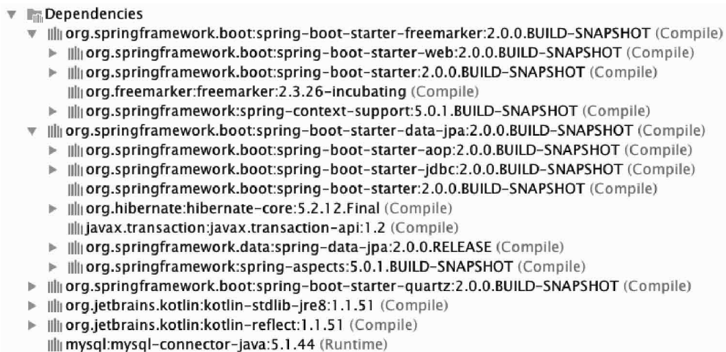
图13-8 整个项目的依赖情况
