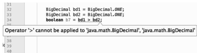
图11-1 对象类型上不允许使用比较运算符
