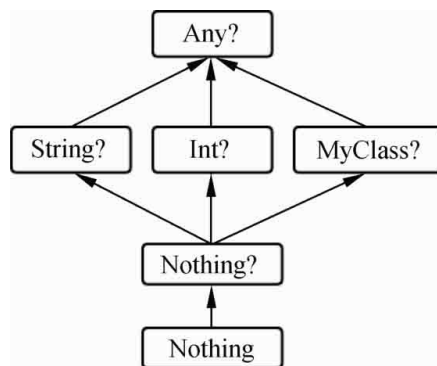
图3-4 Nothing类型层次结构
