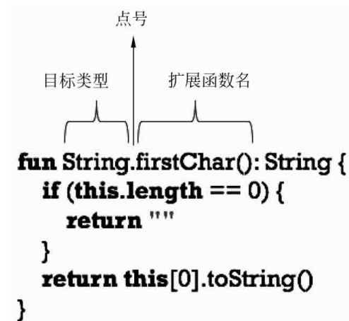
图6-1 给String类型扩展一个firstChar()函数
