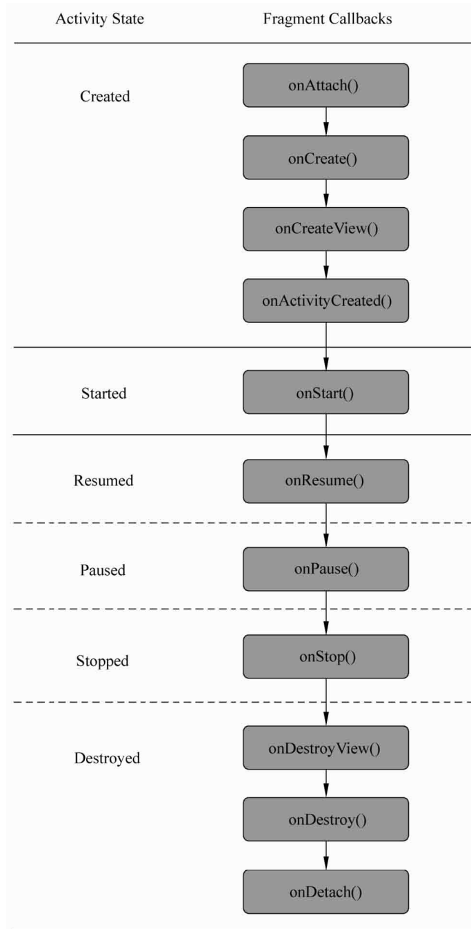
图14-35 Fragment与Activity的生命周期对比
