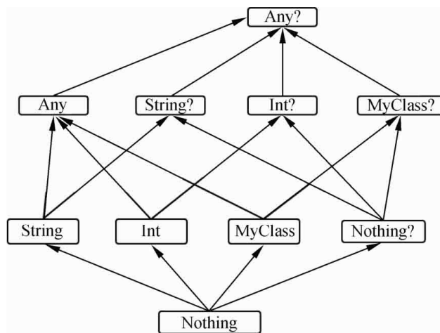
图3-2 Kotlin类型层次结构
