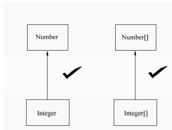
图8-2 Java中的数组是协变的
