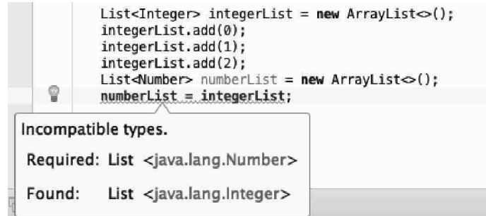
图8-4 编译错误：类型不兼容
