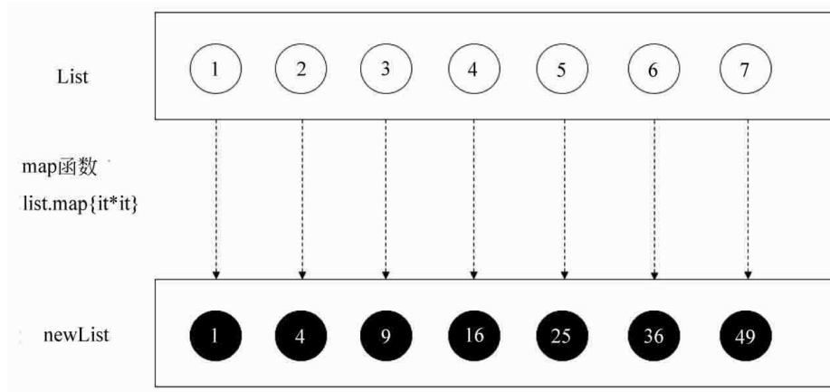
图7-9 map函数的映射图
