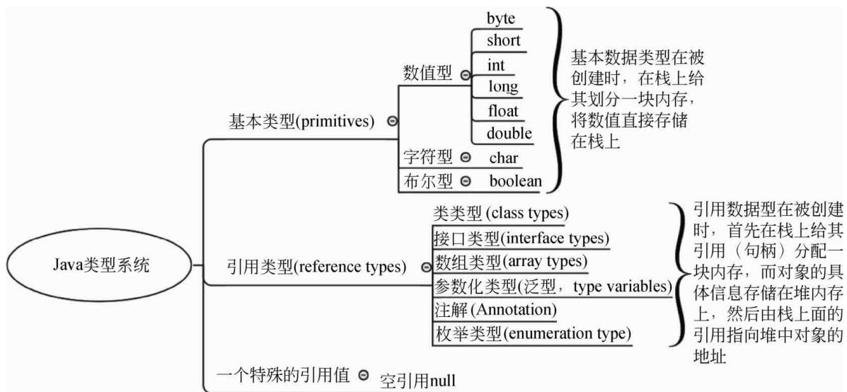
图3-1 Java类型系统
