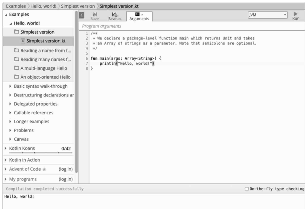
图1-1 Kotlin云端IDE
