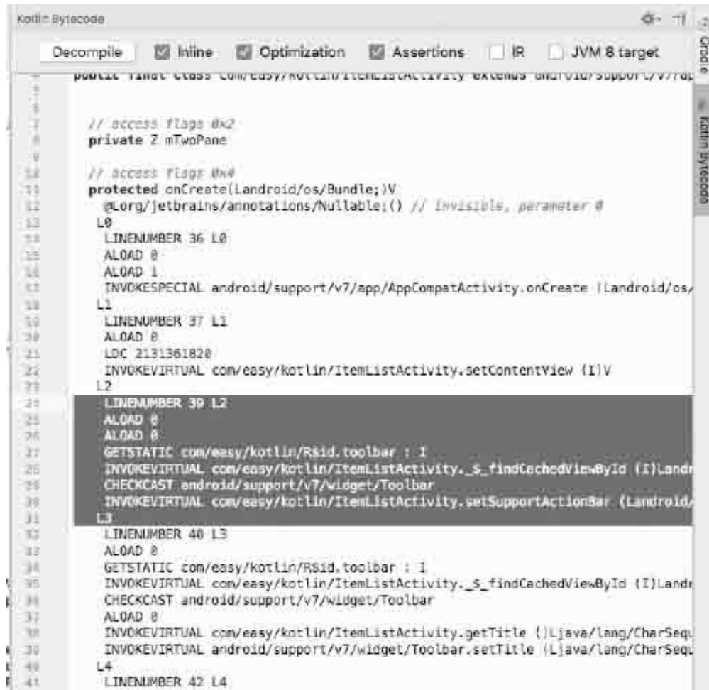
图14-29 Kotlin Bytecode界面
