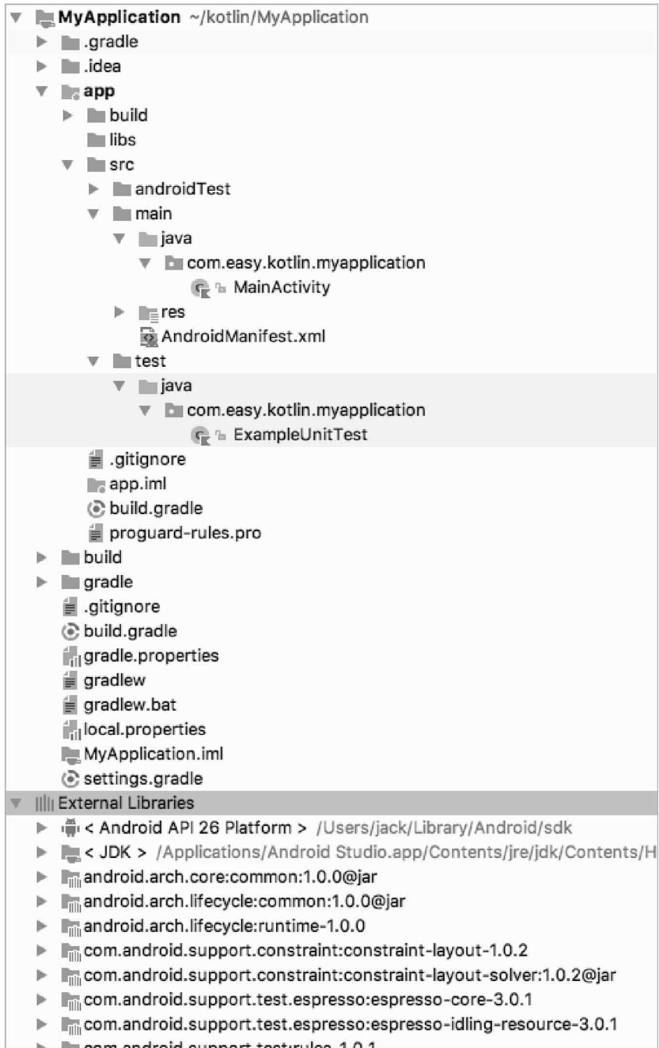
图14-13 工程目录
