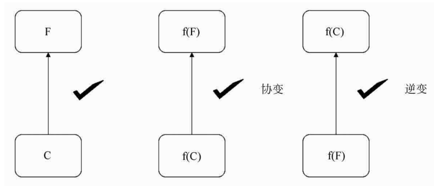
图8-1 协变与逆变
