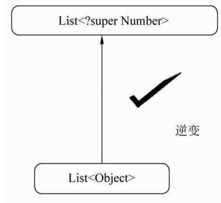
图8-8 逆变
