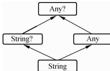
图3-5 Any 类型层次结构
