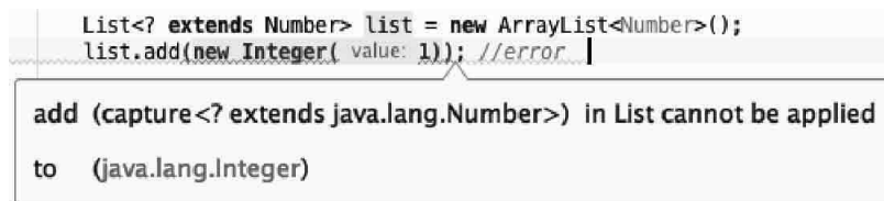
图8-5 类型不兼容的报错信息
