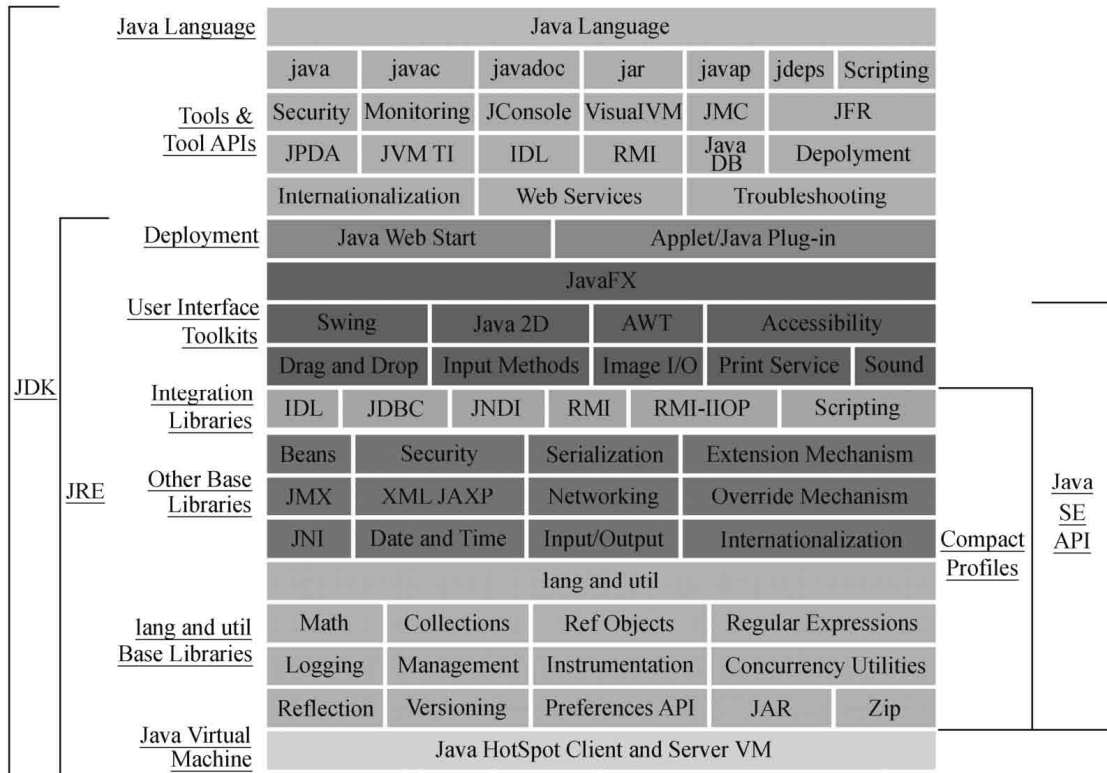
图1-3 Java技术模块架构图
