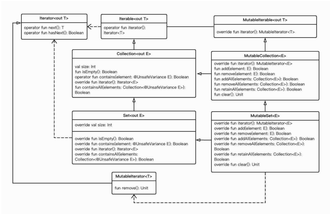
图7-4 Set集合的类型层次结构
