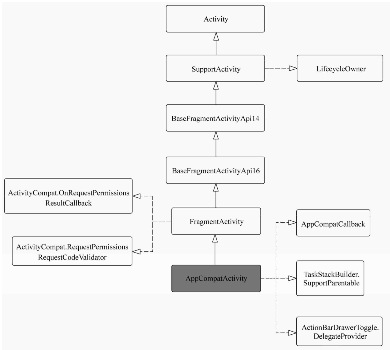
图14-25 AppCompatActivity的类图继承层次
