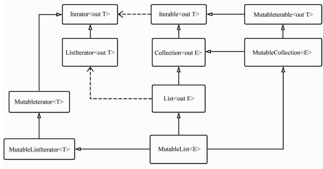
图7-3 List列表的类型层次结构
