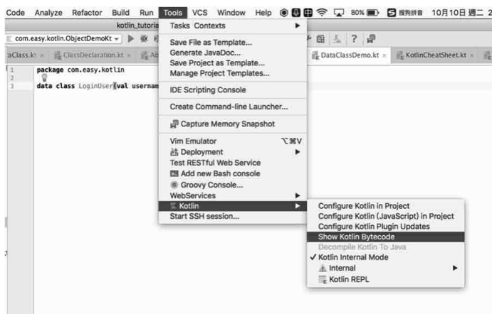
图4-10 选择菜单栏中的Show Kotlin Bytecode命令
