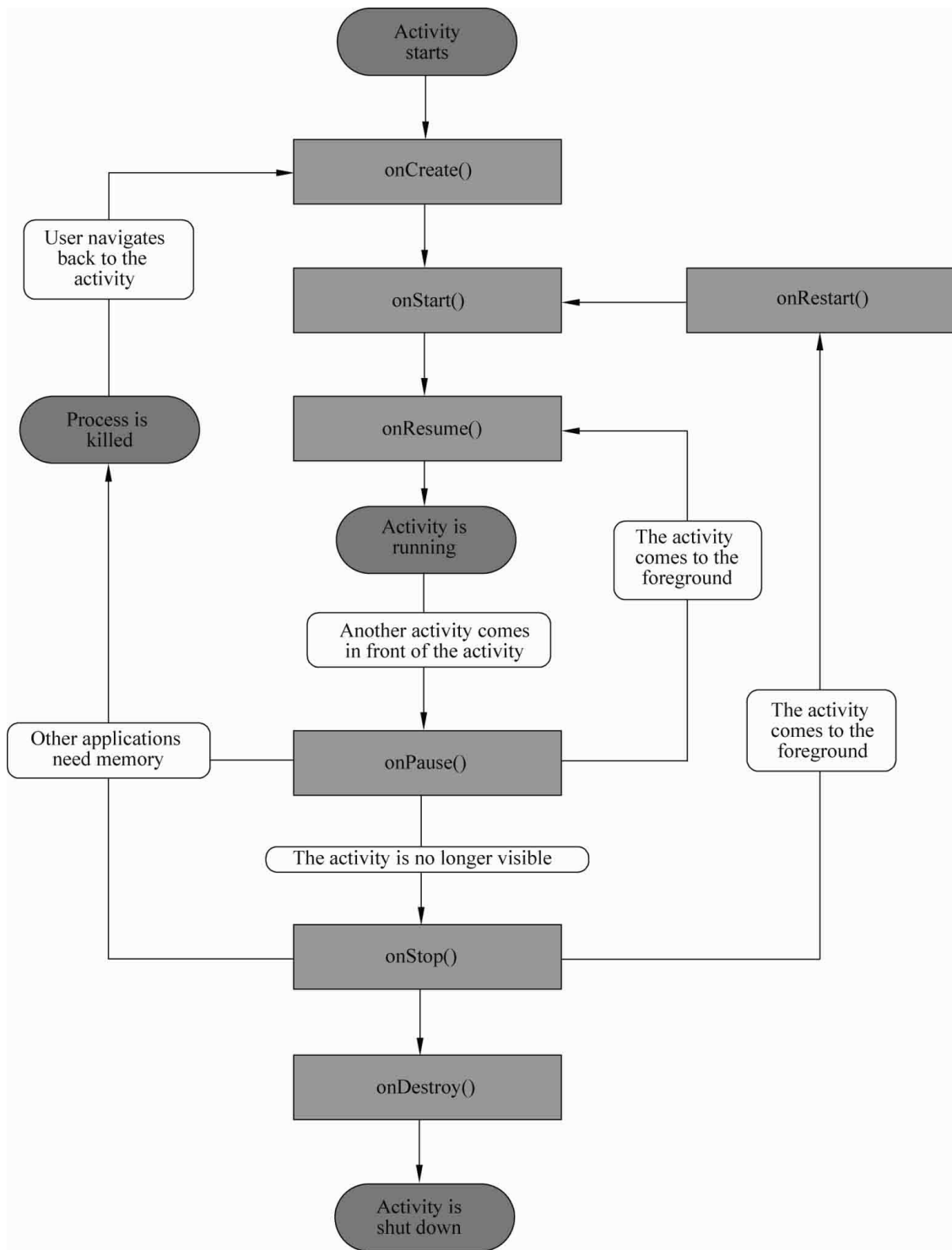
图14-26 Activity的生命周期
