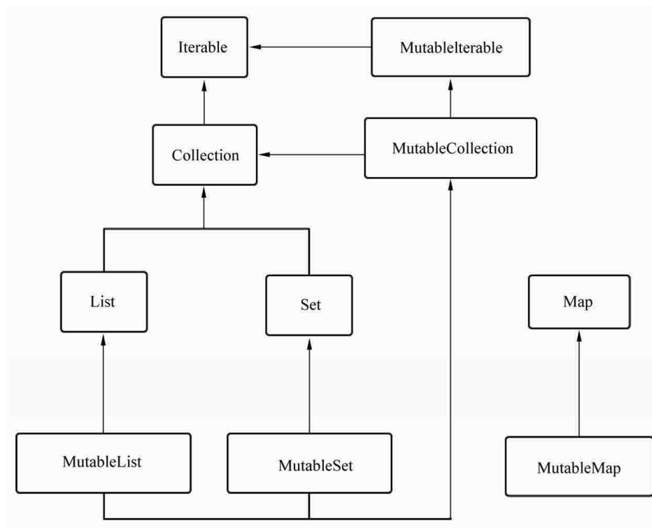
图7-2 集合类接口结构层次
