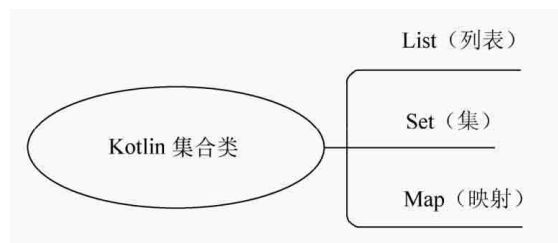
图7-1 Kotlin集合类
