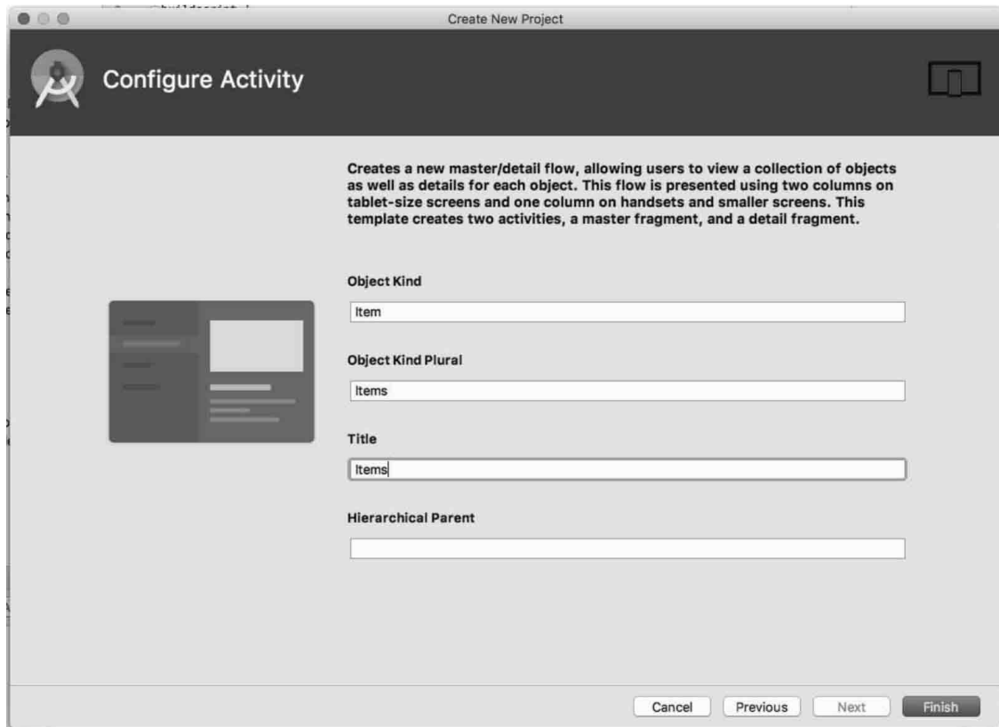
图14-20 配置Activity
