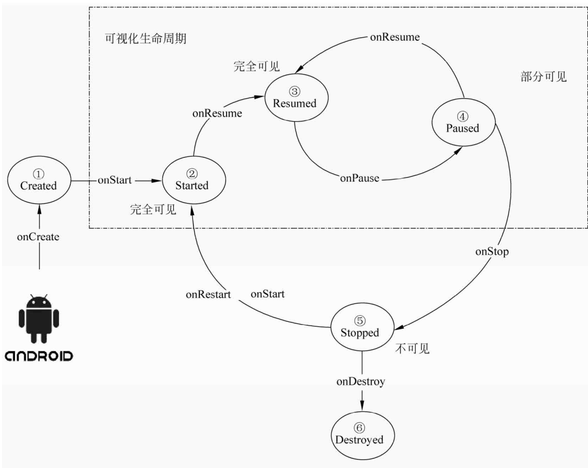
图14-27 Activity状态图
