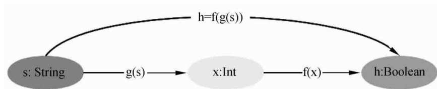
图5-3 复合函数h的映射关系
