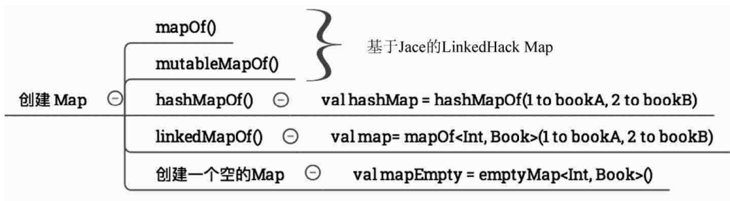
图7-8 创建Map
