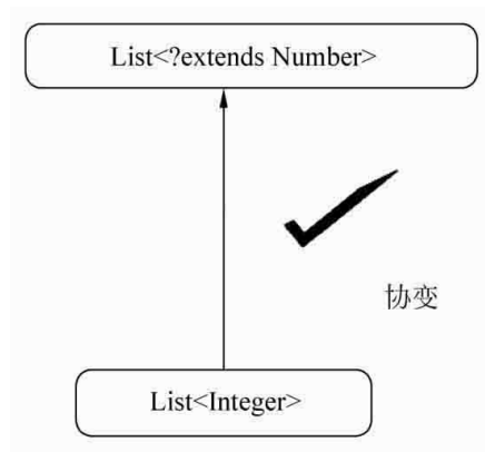
图8-6 协变
