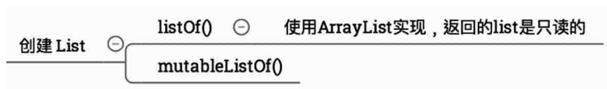
图7-6 创建List
