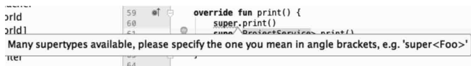
图4-9 覆盖冲突
