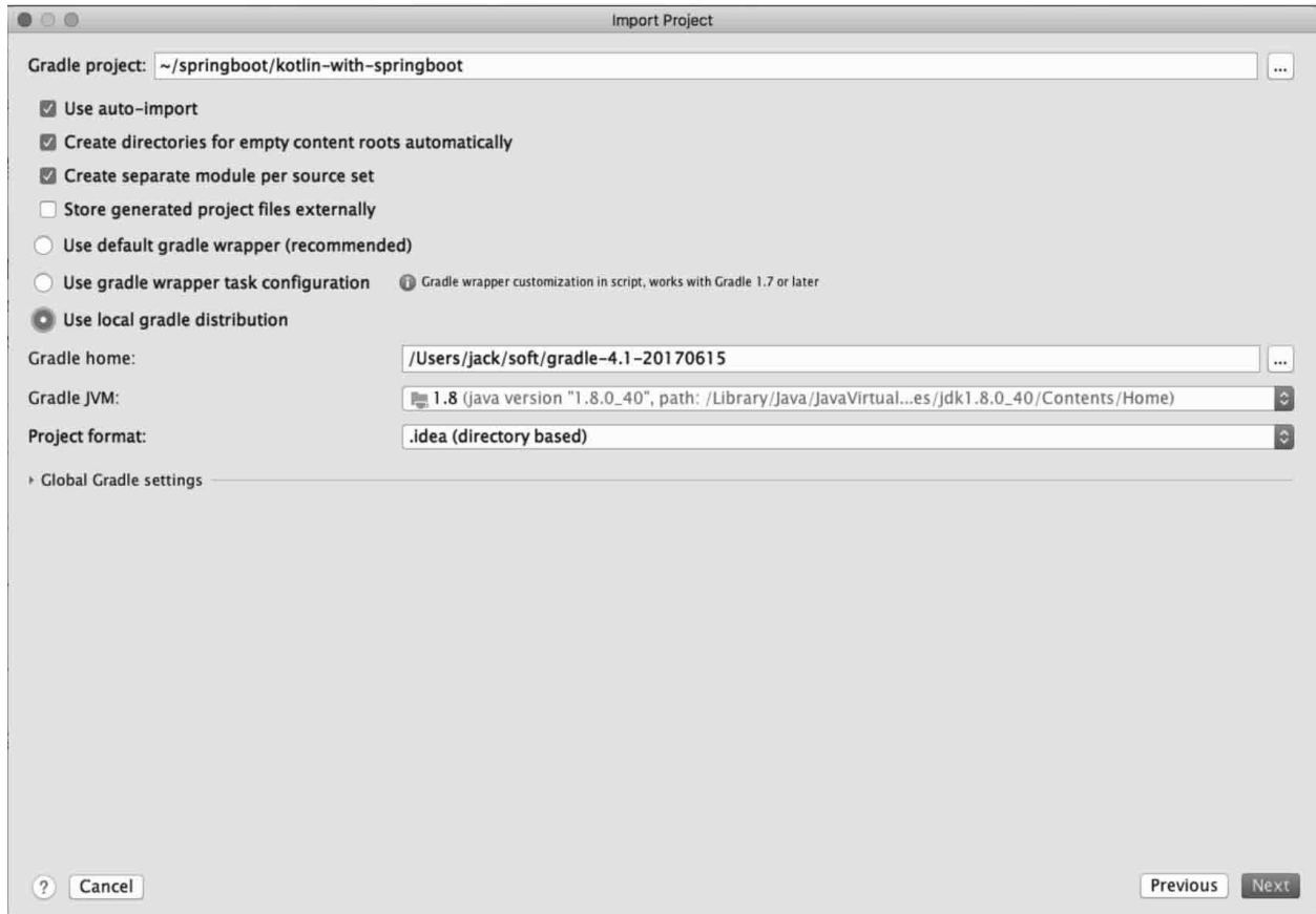
图13-3 解压工程导入IDEA中
