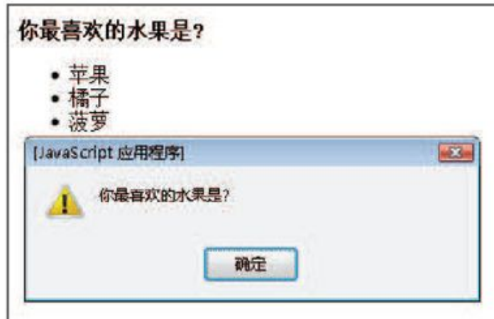
图3-29 获取<p>元素的文本内容
