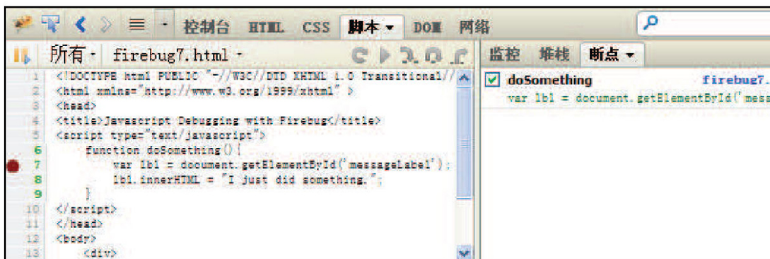
图B-24 设置断点
