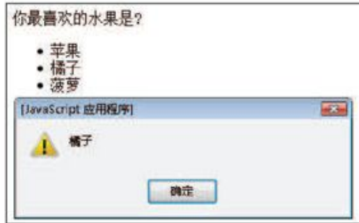
图3-3 查找元素节点
