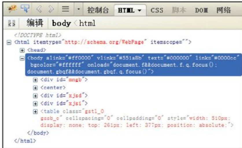
图B-3 Firebug面板
