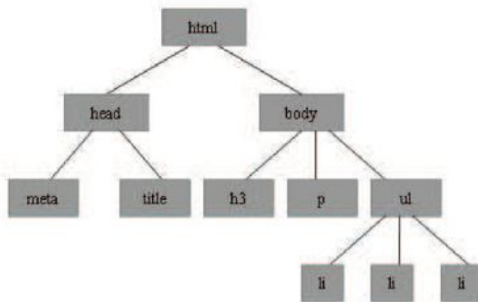
图1-14 把网页元素表示为DOM树
