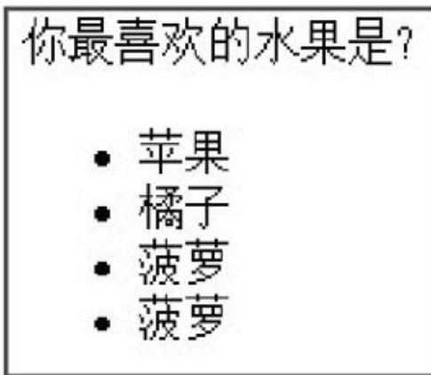
图3-20 复制节点
