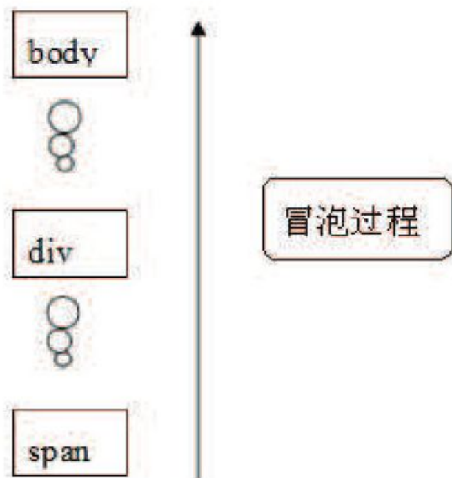
图4-12 冒泡过程
