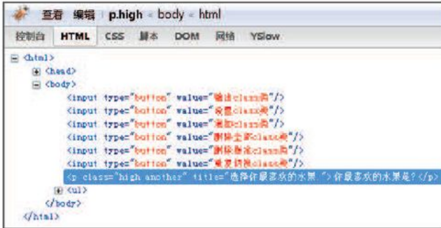
图3-27 class代码
