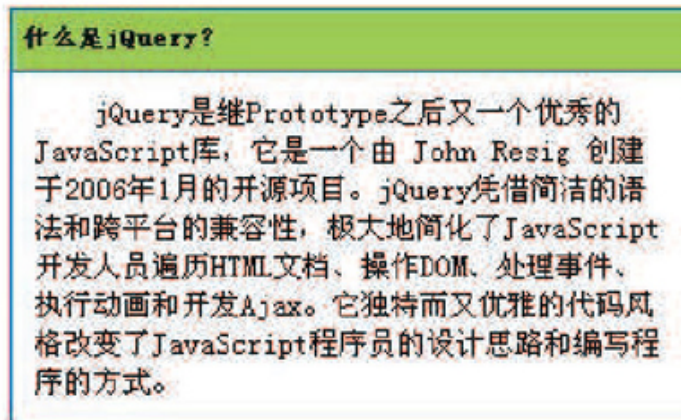
图4-6 内容显示
