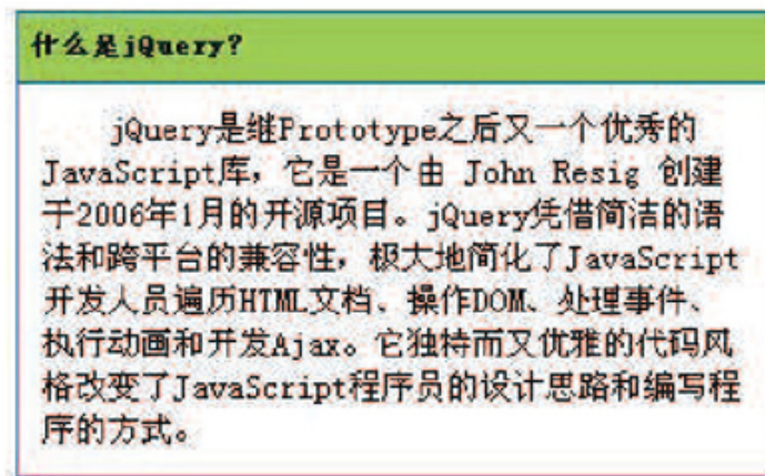
图4-5 显示内容
