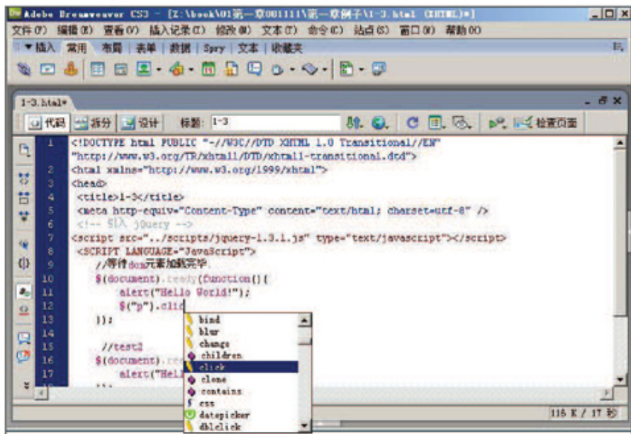
图1-19 自动提示
