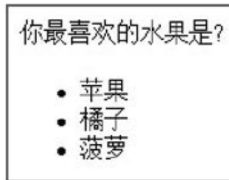
图3-11 移动之前
