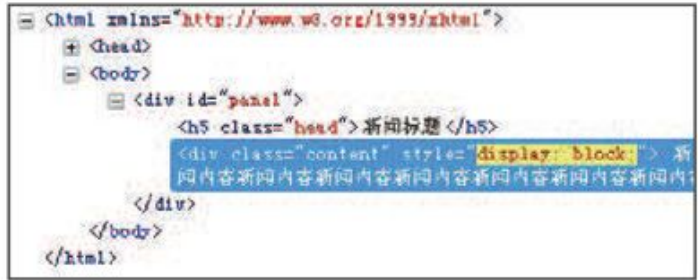
图4-22 执行show()方法
