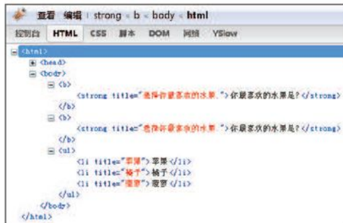
图3-23 用wrap()方法包裹节点源文件
