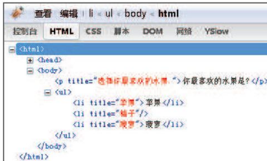
图3-18 清空后的源文件
