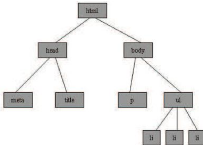
图3-36 DOM树
