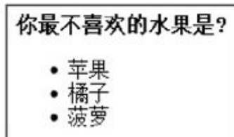
图3-21 替换节点
