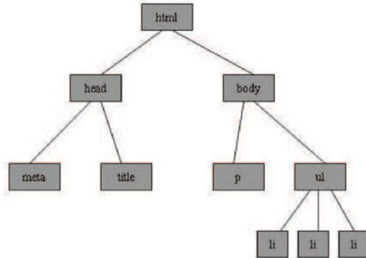
图3-2 DOM结构
