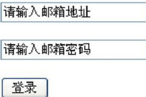
图3-33 初始化效果
