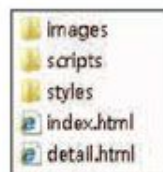
图8-1 目录结构
