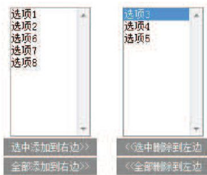
图5-13 最终效果
