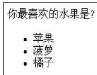
图3-12 移动之后
