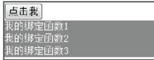
图4-18 模拟操作
