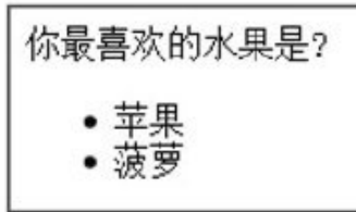
图3-13 删除节点
