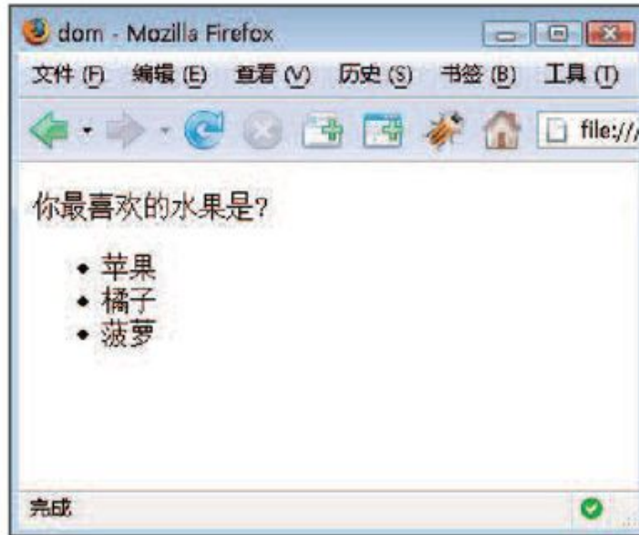
图3-1 构建的网页
