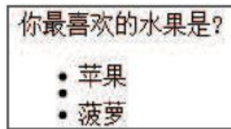
图3-17 清空元素
