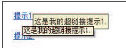
图3-38 超链接提示
