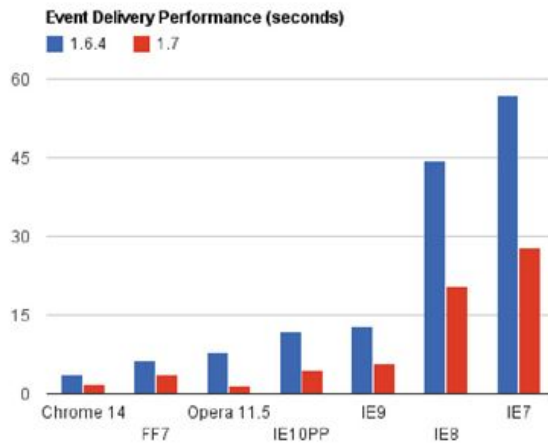
图10-1 不同版本的性能比较
