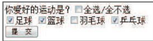
图5-10 复选框和复选框组相互影响
