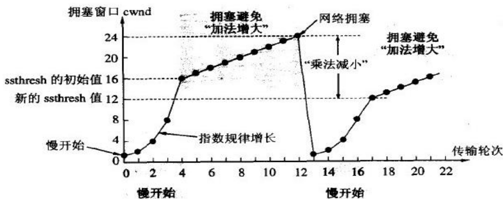
图 5-25 慢开始和拥塞避免算法的实现举例 net/sicofield
