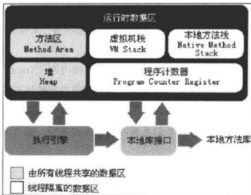
图 2-1 Java 虚拟机运行时数据区
