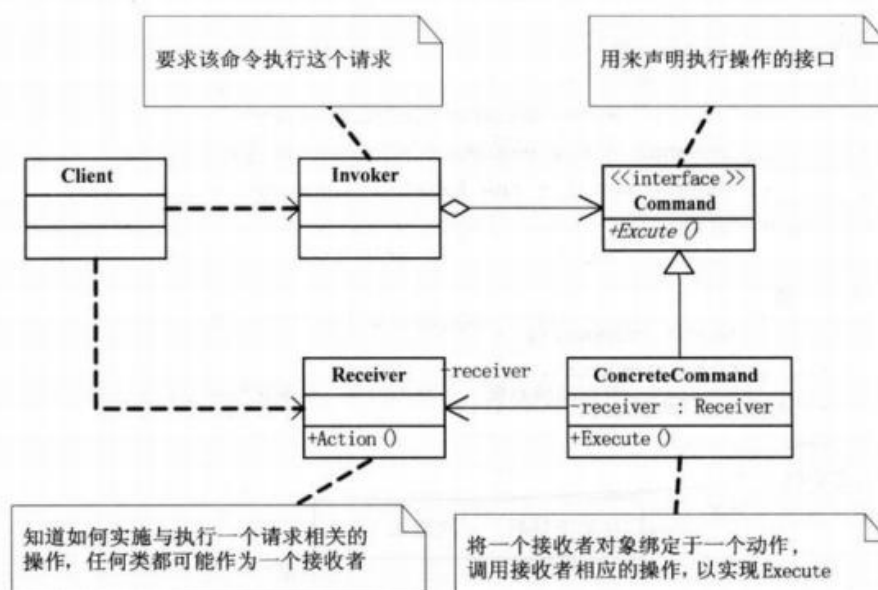
命令模式 (Command) 结构图
