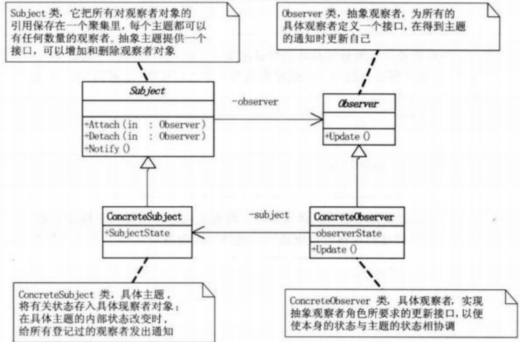
观察者模式 (Observer) 结构图
