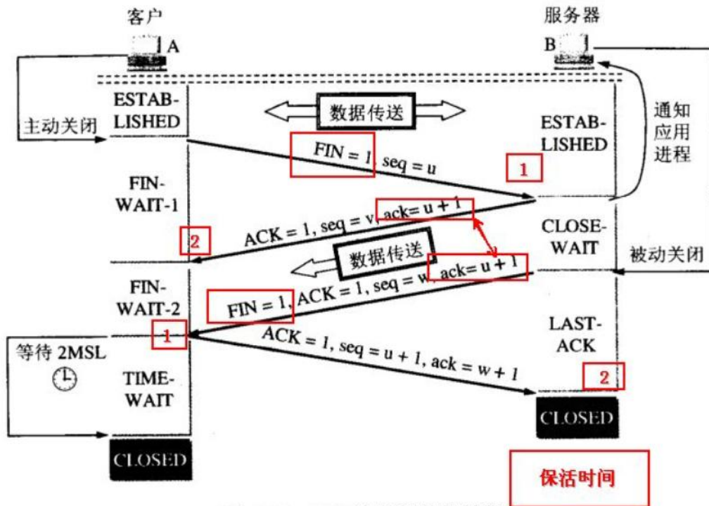
图 5-32 TCP 连接释放的过程
