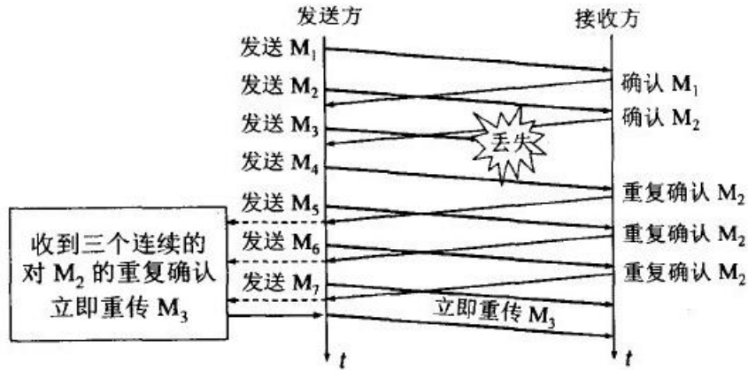
图 5-26 快重传的示意图
