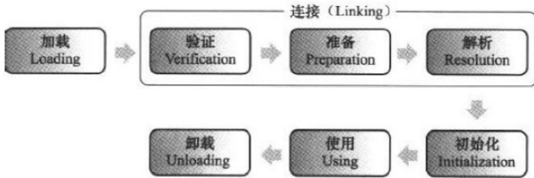
图 7-1 类的生命周期
