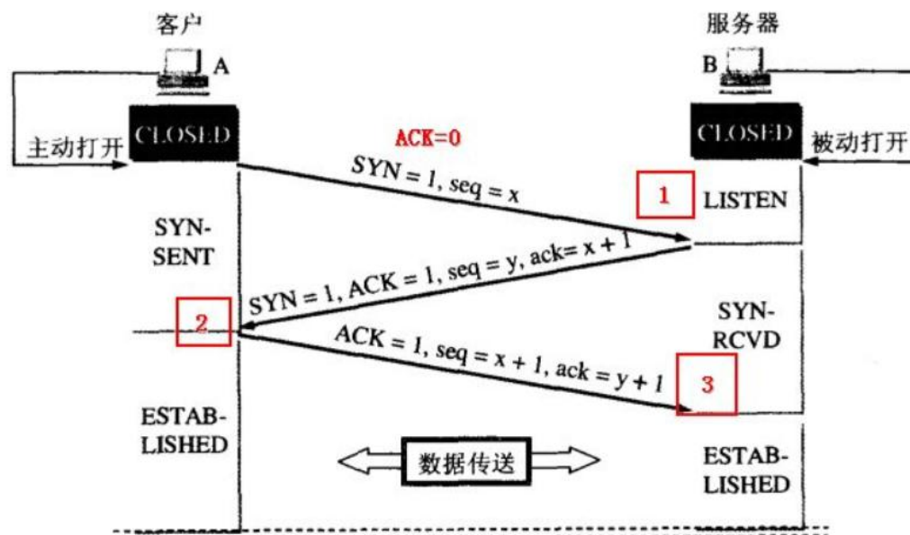
图 5-31 用三次握手建立 TCP 连接
