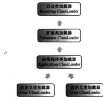
图 7-2 类加载器双亲委派模型
