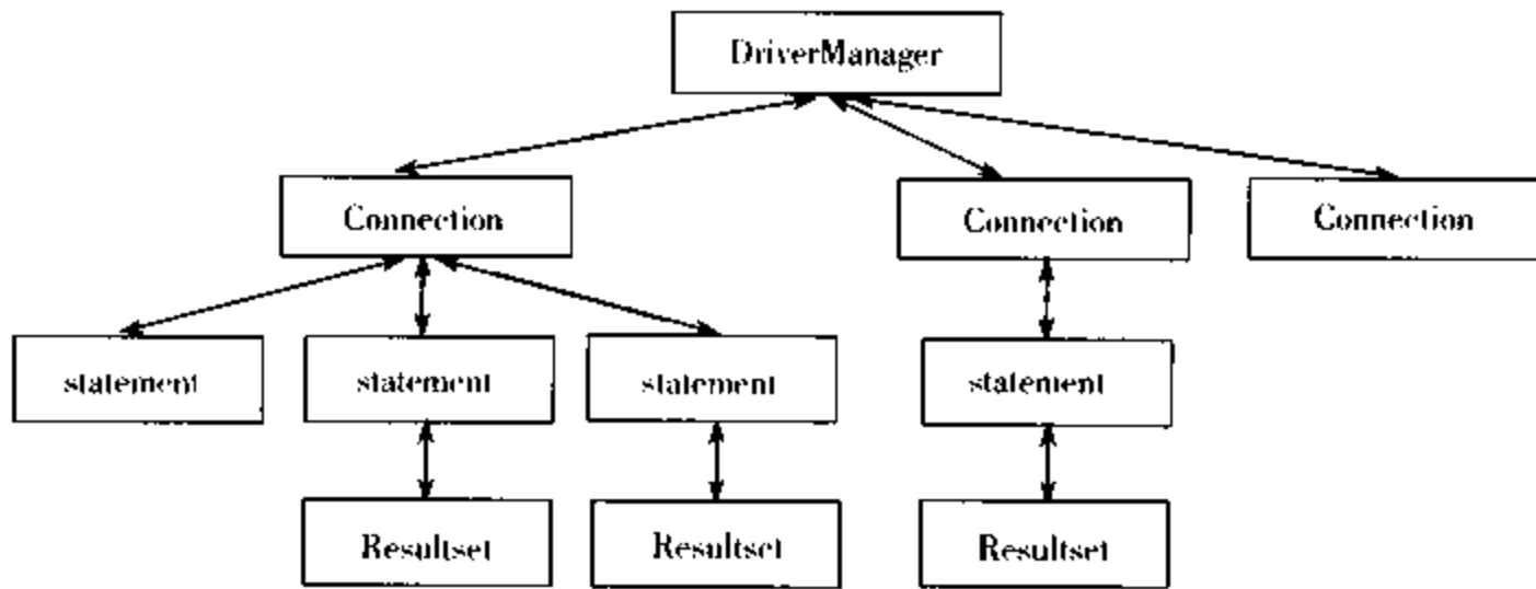
图 4.6 JDBC API 的类
