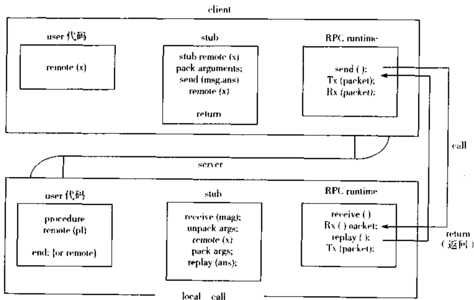
图 5.2 RPC 的实现原理
