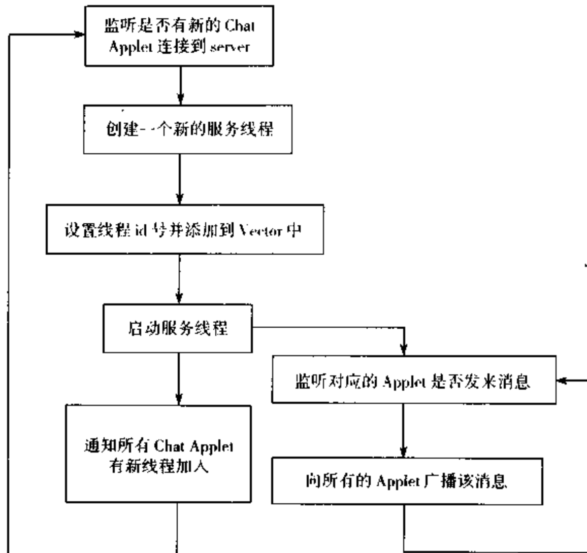
图 2.10 Chat Server 的流程图
