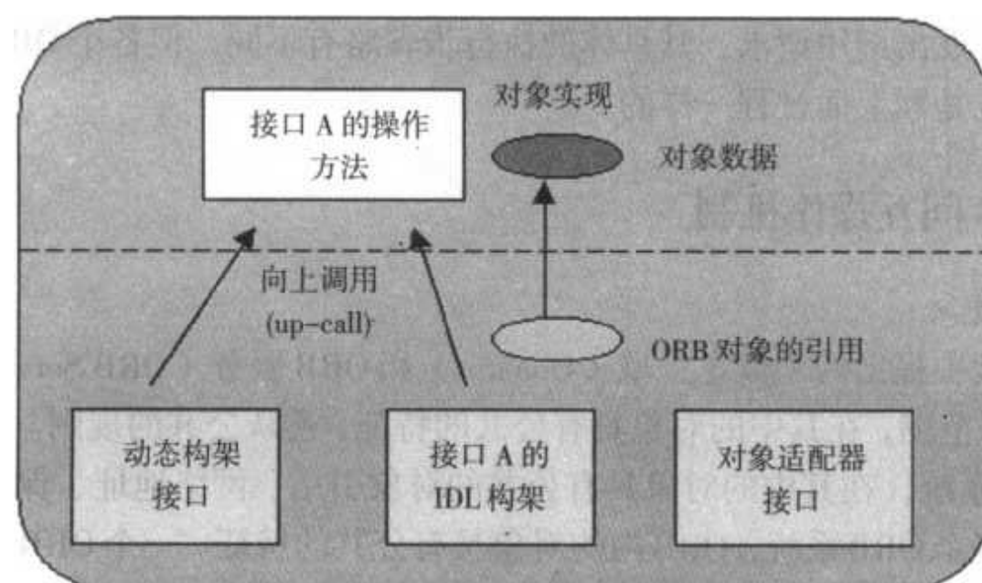
图 6.5 对象实现的组成
