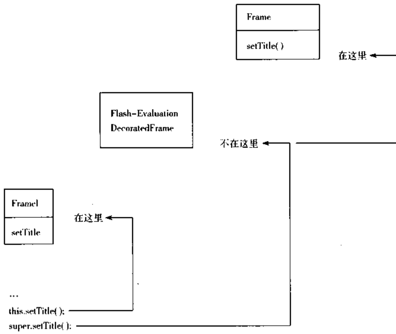
图 1.18 含有重载方法的 Frame 类层次
