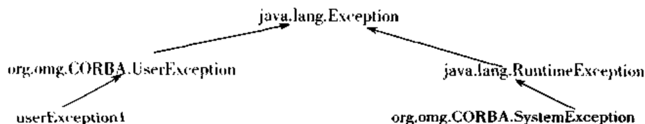
图 6.9 异常类型的继承关系
