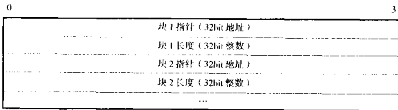
图2.3 用于writev和readv的iovec类型的iovector的格式
