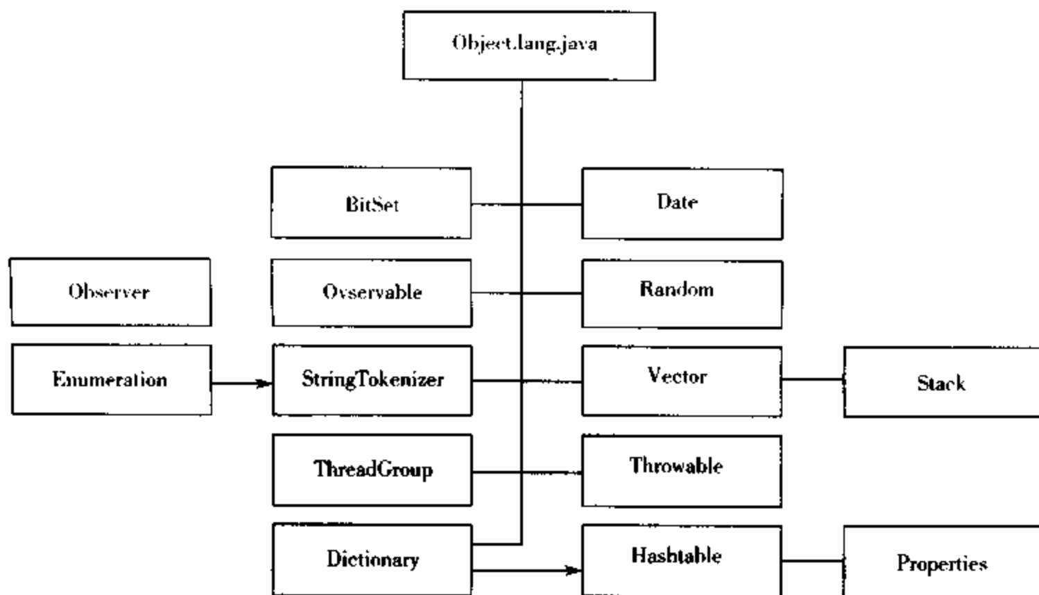
图 1.21 Utility 类库的层次结构
