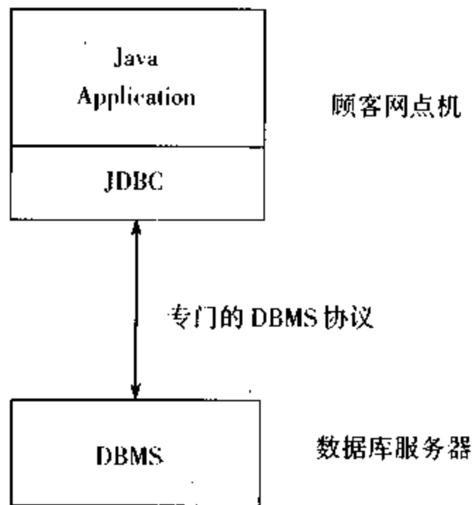
图 4.1 两层的客户/服务方式
