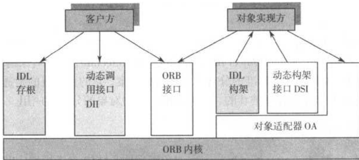
图 6.2 单个 ORB 体系结构
