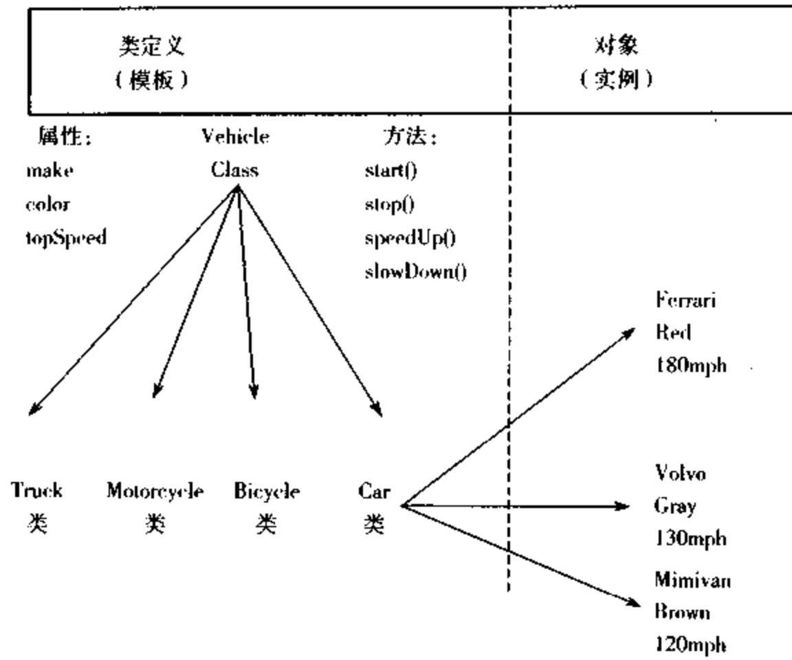
图 1.5 vehicle 类是 Truck、Motorcycle、Bicycle 和 Car 的基类
