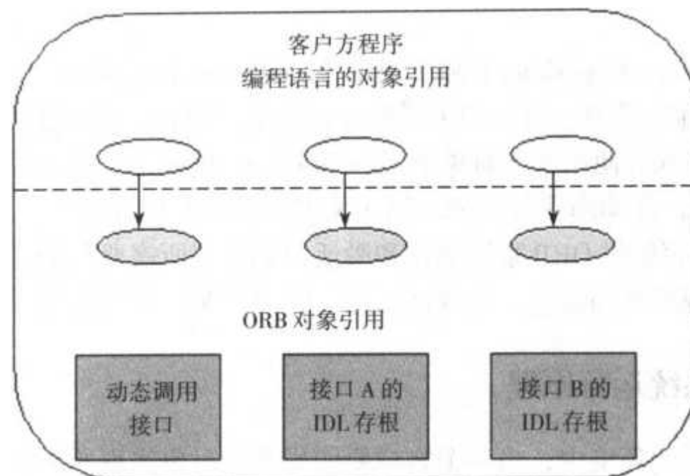
图 6.4 客户方程序的组成
