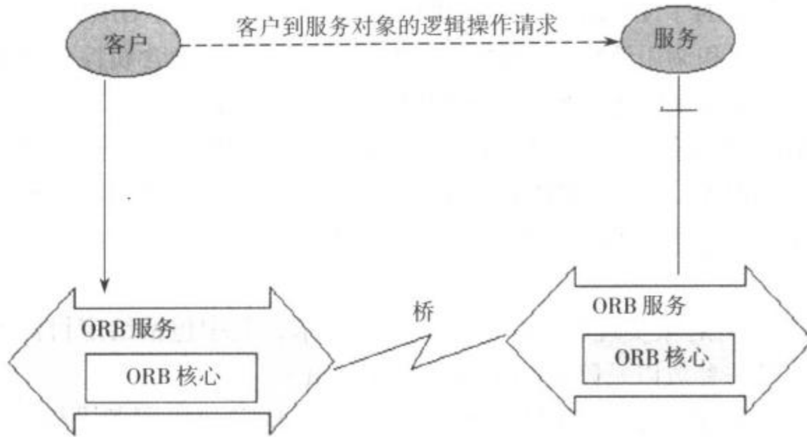
图 6.6 内嵌式桥接机制示意图
