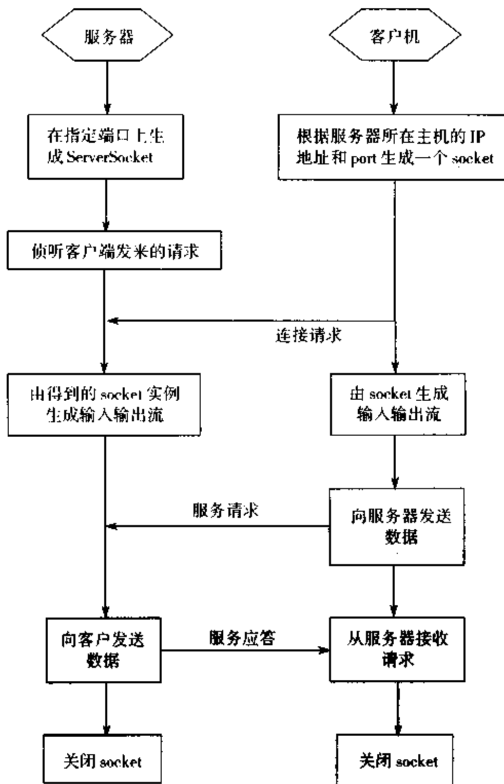
图 2.6 基于无连接的服务者客户流程图
