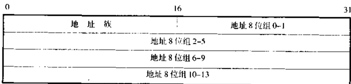
图 2.1 在给套接字接口传递 TCP/IP 地址时使用的 sockaddr 结构
