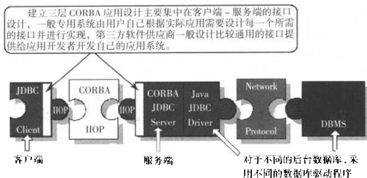
图 6.12 基于三层 CORBA 应用的信息集成原理
