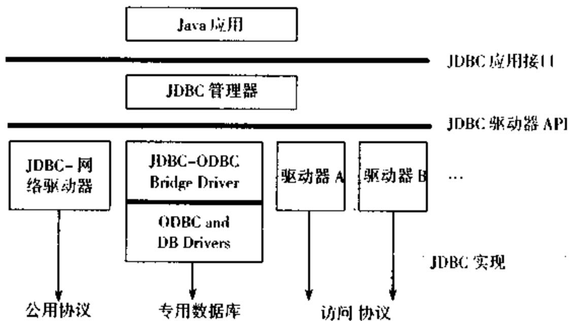
图 4.3 JDBC 总体结构
