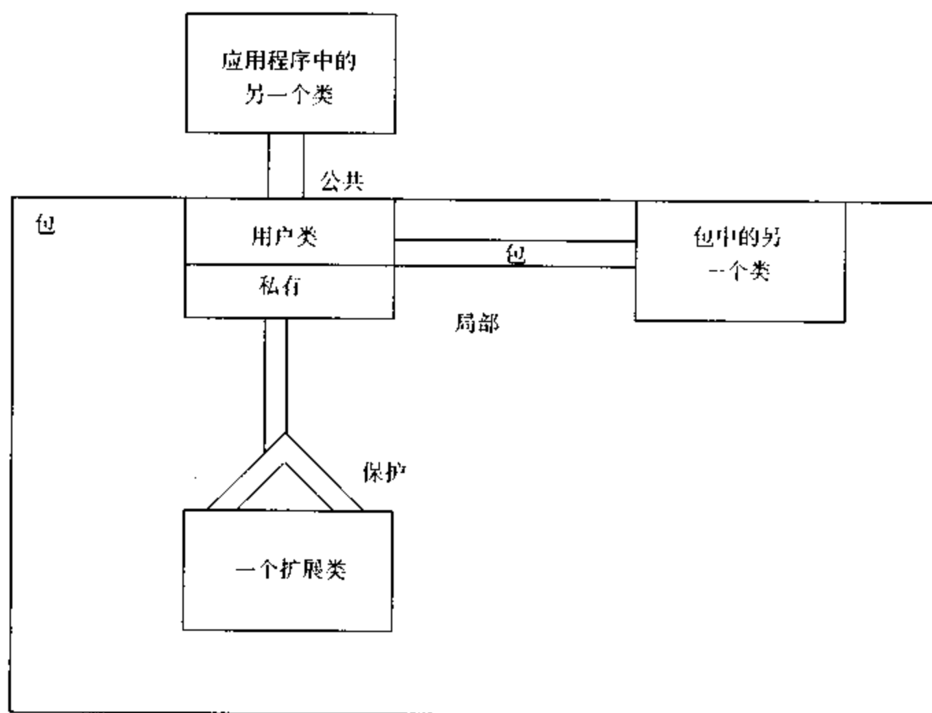
图 1.19 变量与方法的可见性级别
