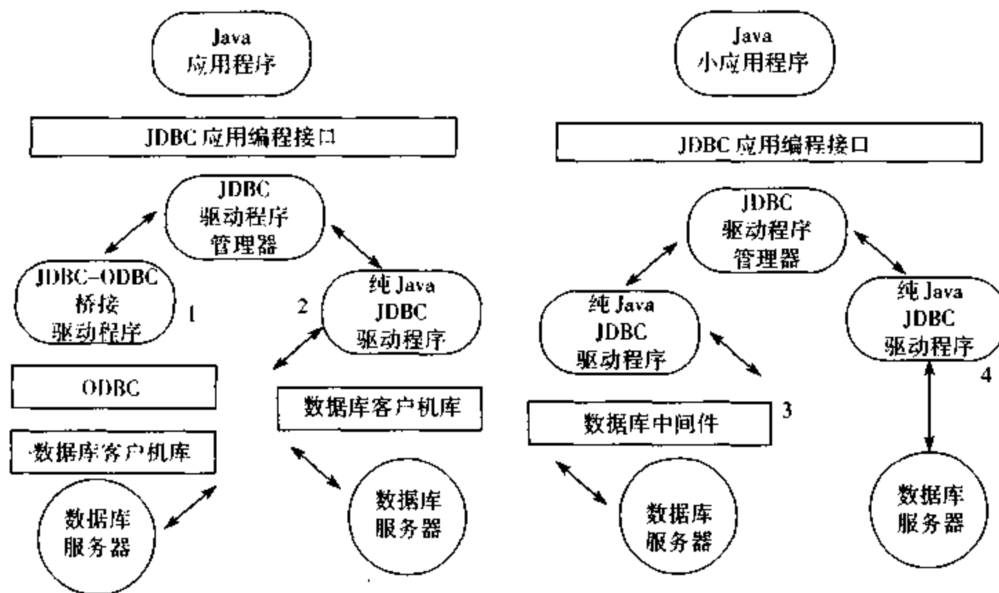
图 4.4 驱动程序的 4 种类型
