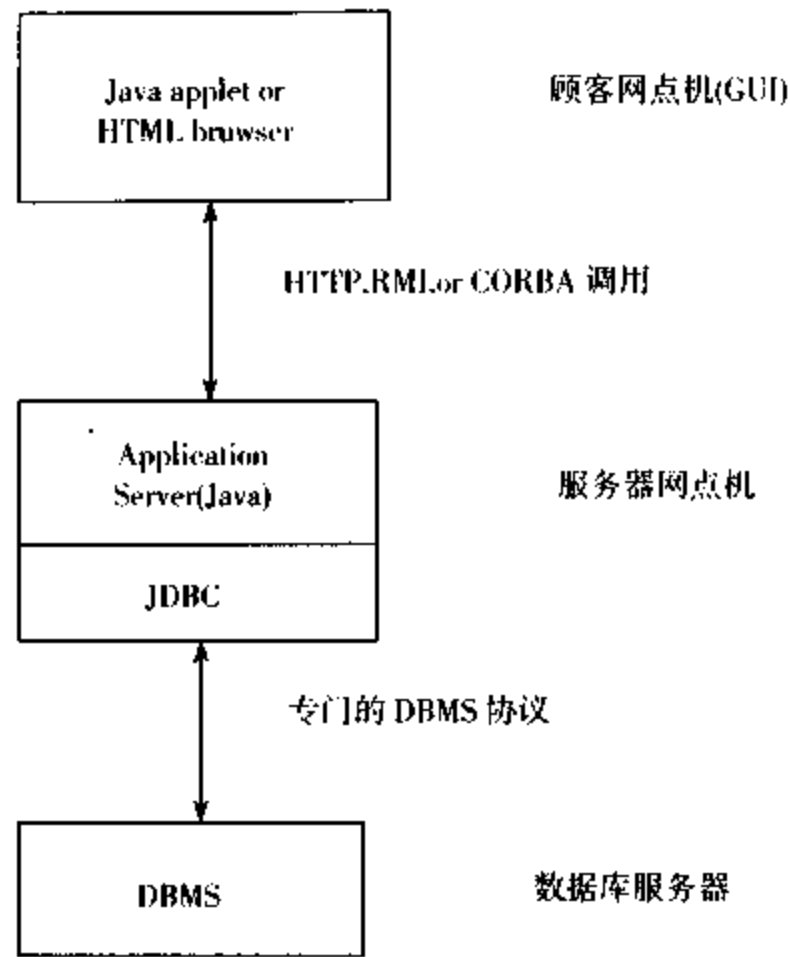
图 4.2 三层结构的客户/服务方式
