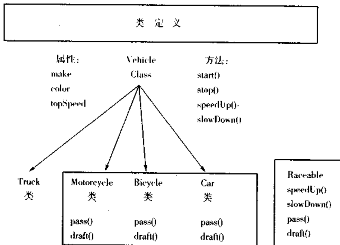
图 1.9 实现 Raceable 接口的类
