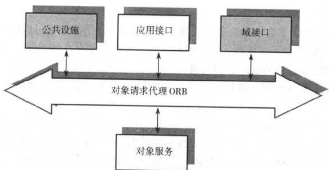
图 6.1 OMA 参考模型
