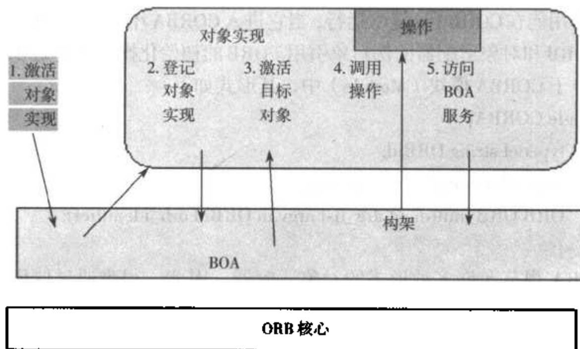
图 6.3 BOA 相关交互关系
