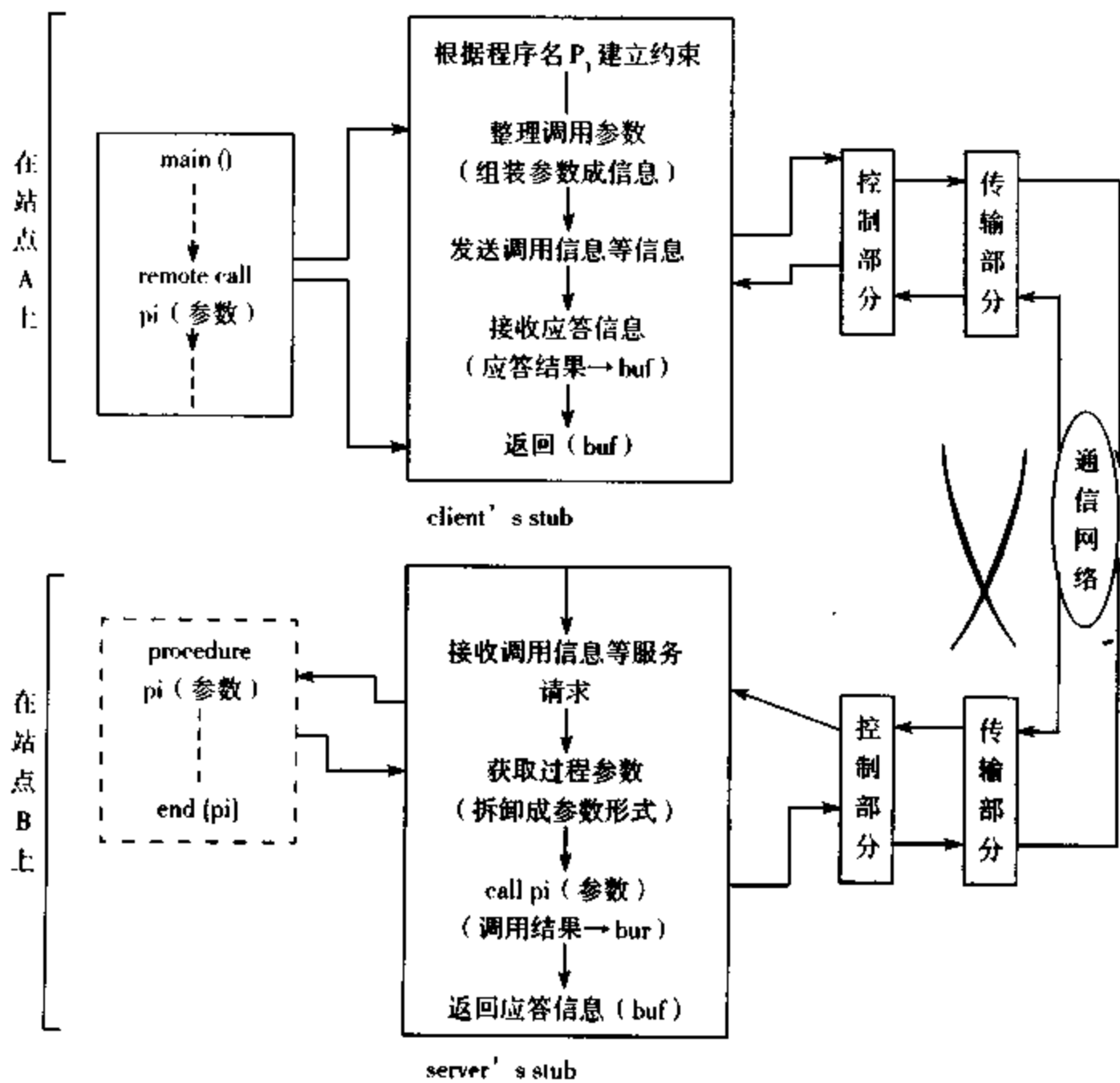
图 5.3 RPC 执行时各部分的关系图
