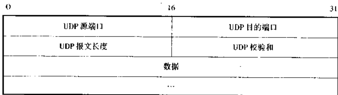
图 2.11 UDP数据报的字段格式
