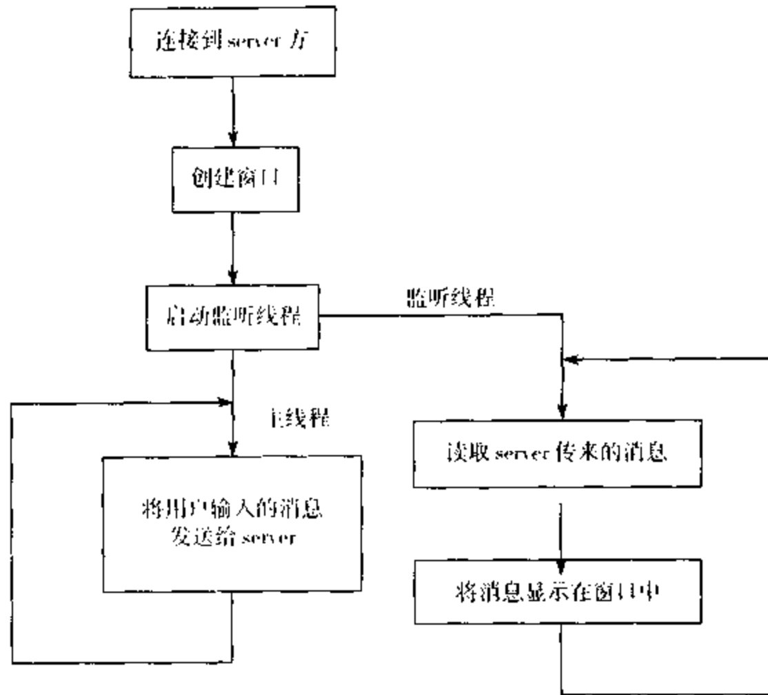
图 2.9 Chat Client 的流程图
