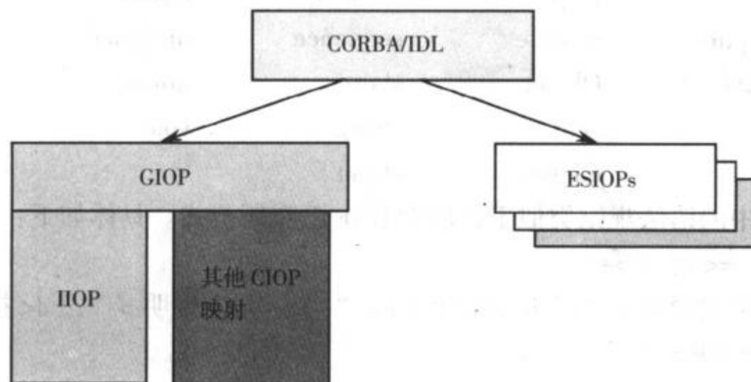
图 6.8 互操作协议之间的关系
