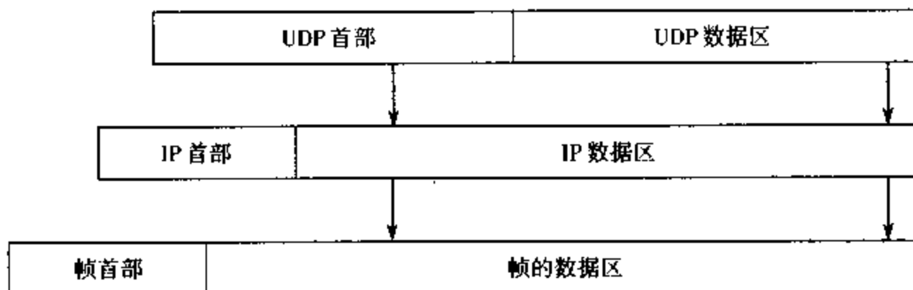
图 2.14 UDP 数据报协议
