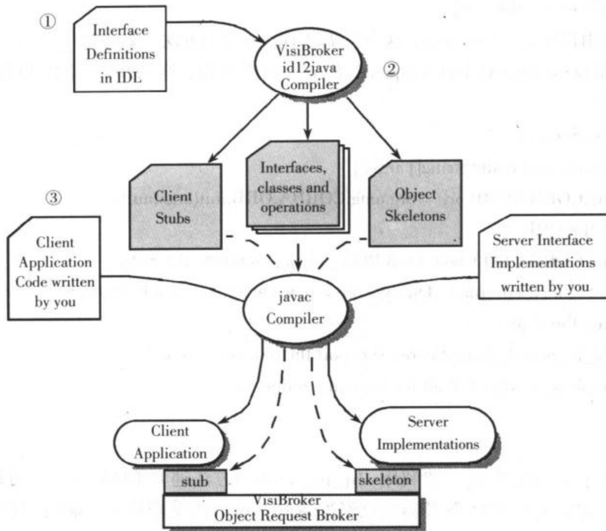
图 6.13 利用 VisiBroker 开发 CORBA 应用程序的过程
