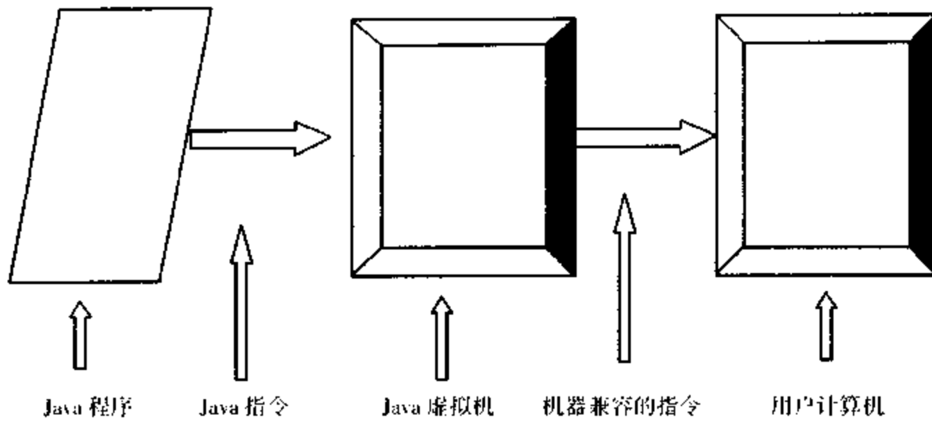
图 1.1 Java 虚拟机
