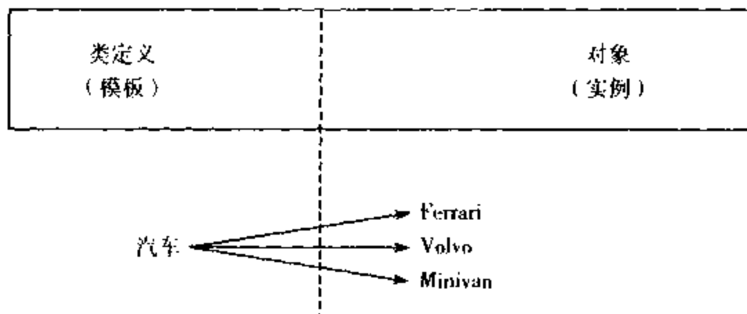
图 1.3 类和对象
