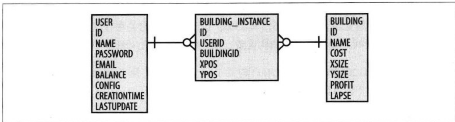
图 5-1 关联用户与建筑物的数据模型
