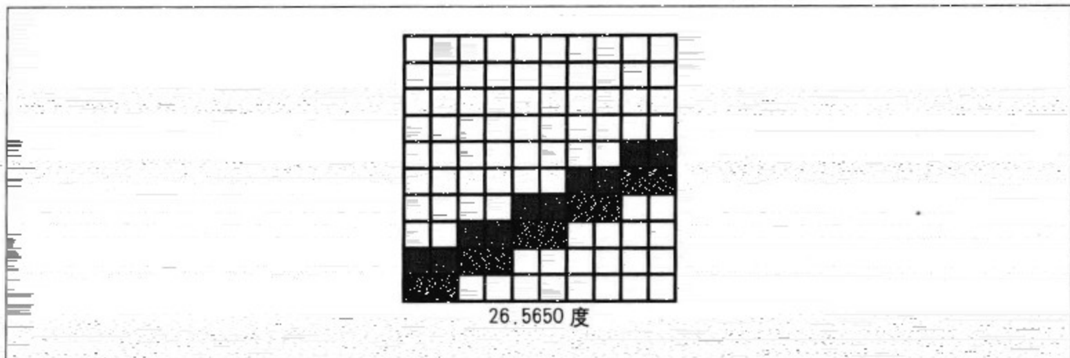
图 2-2 绘制角度为 26.5650^\circ 的直线能得到整洁的结果
