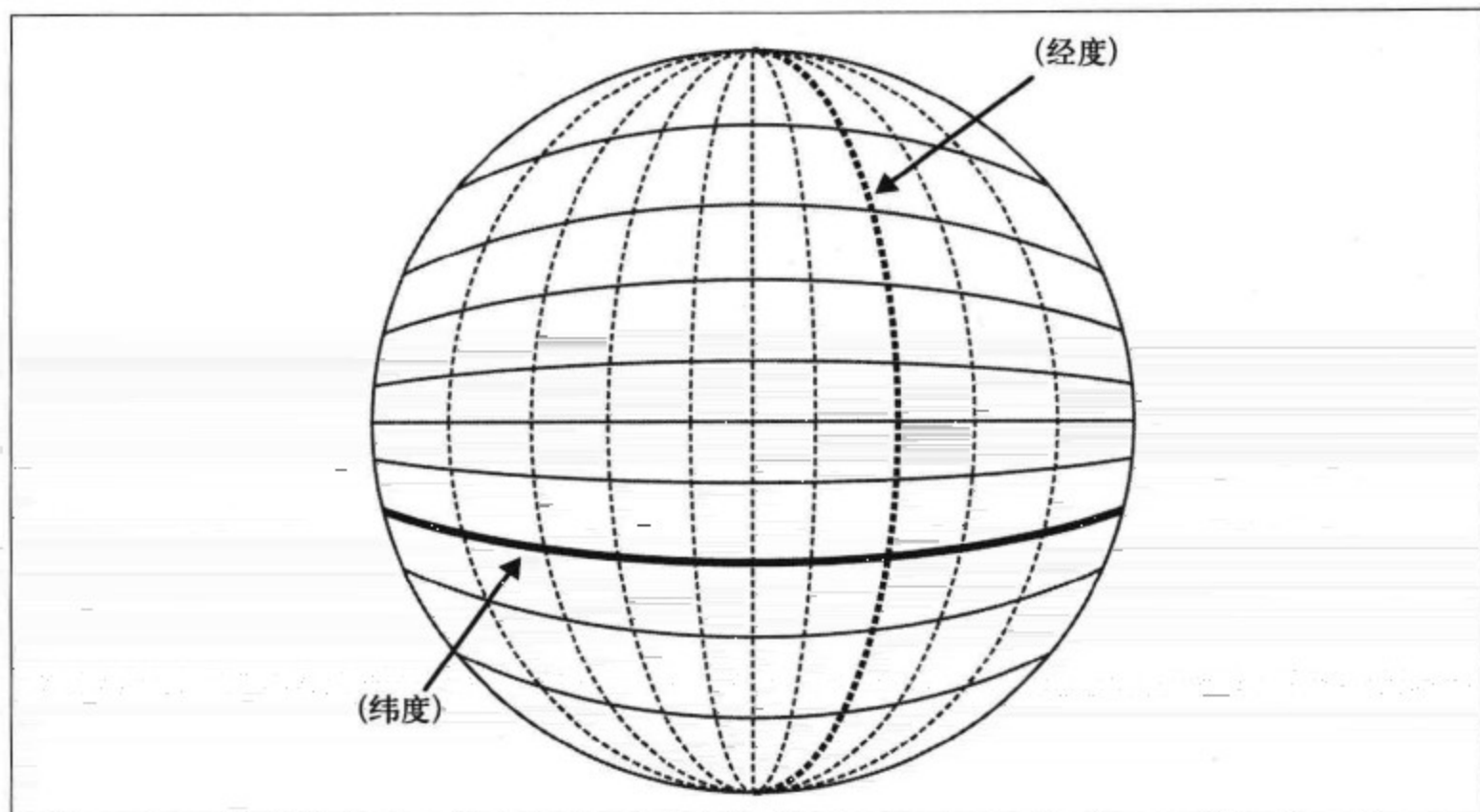
图 2-1 地球上的经、纬度示意图
