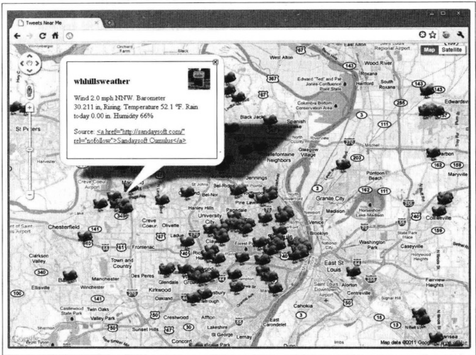
图 6-1 综合使用 W3C Geolocation API 和 Twitter Search API
