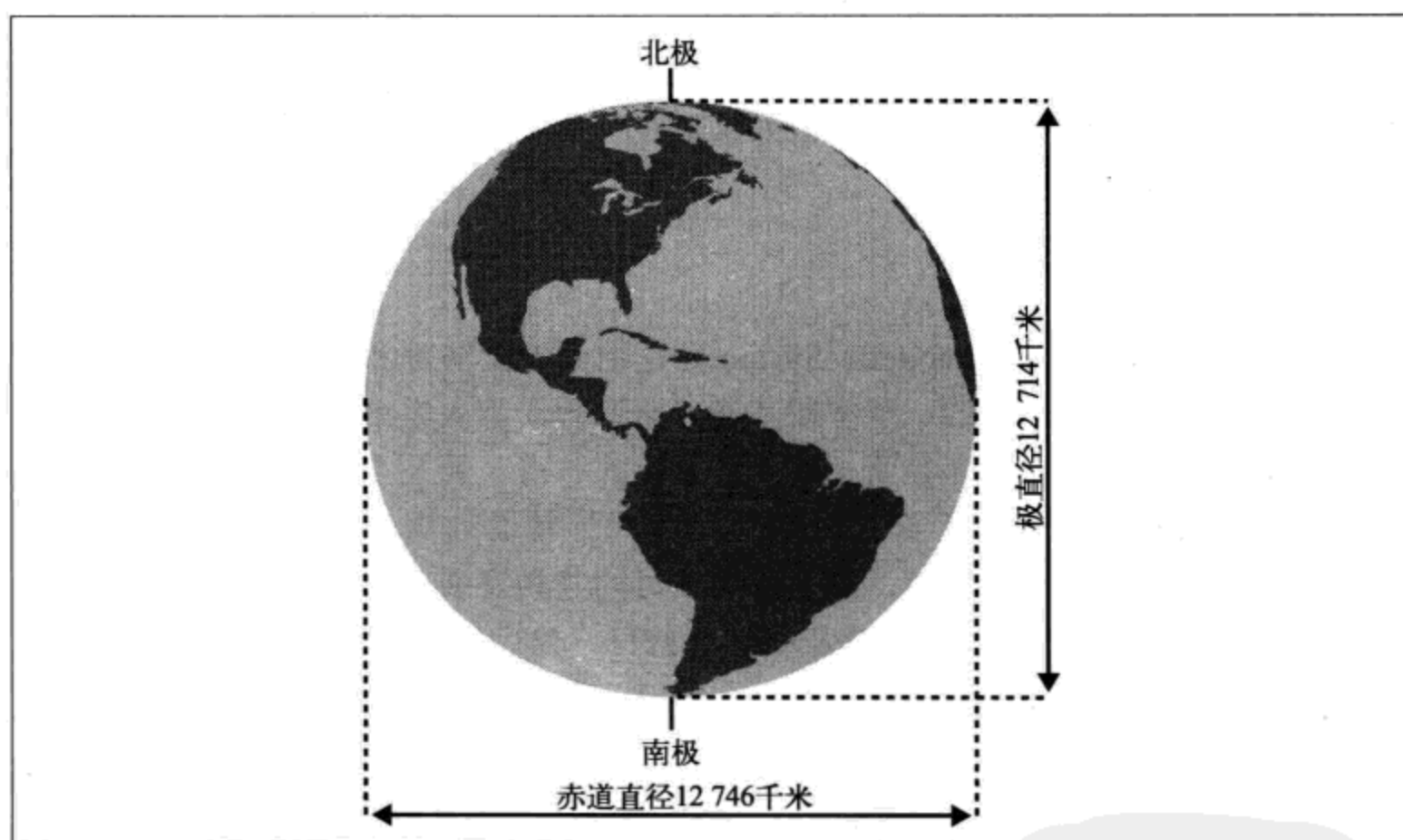
图 2-2 地球是椭球体
