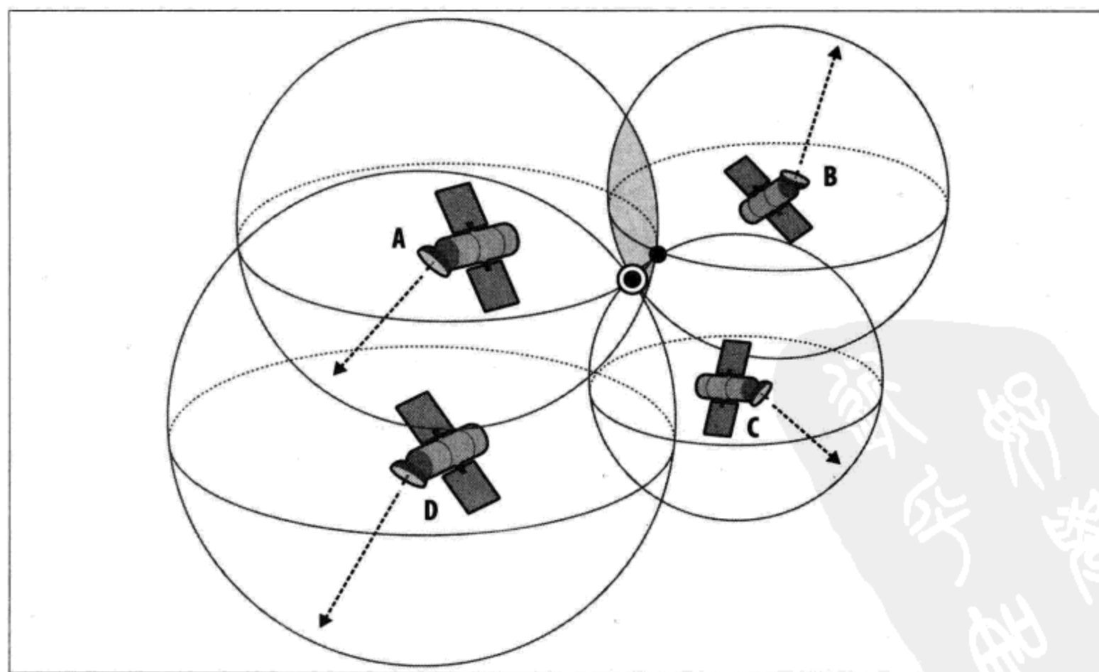
图 1-4 使用卫星的全球定位系统
