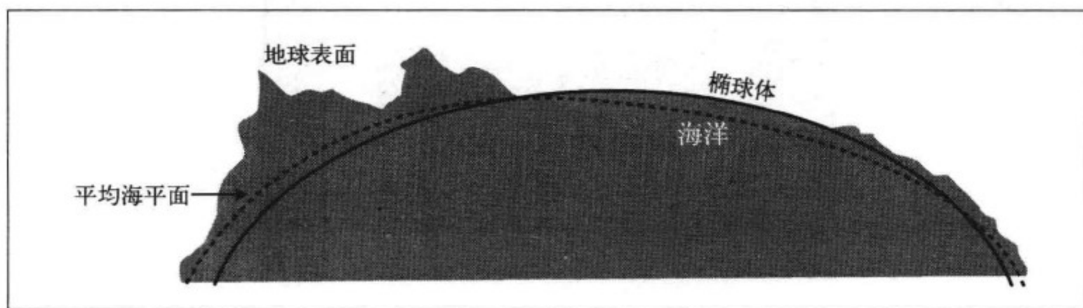
图 2-4 地球上任何一点的高度都不相同
