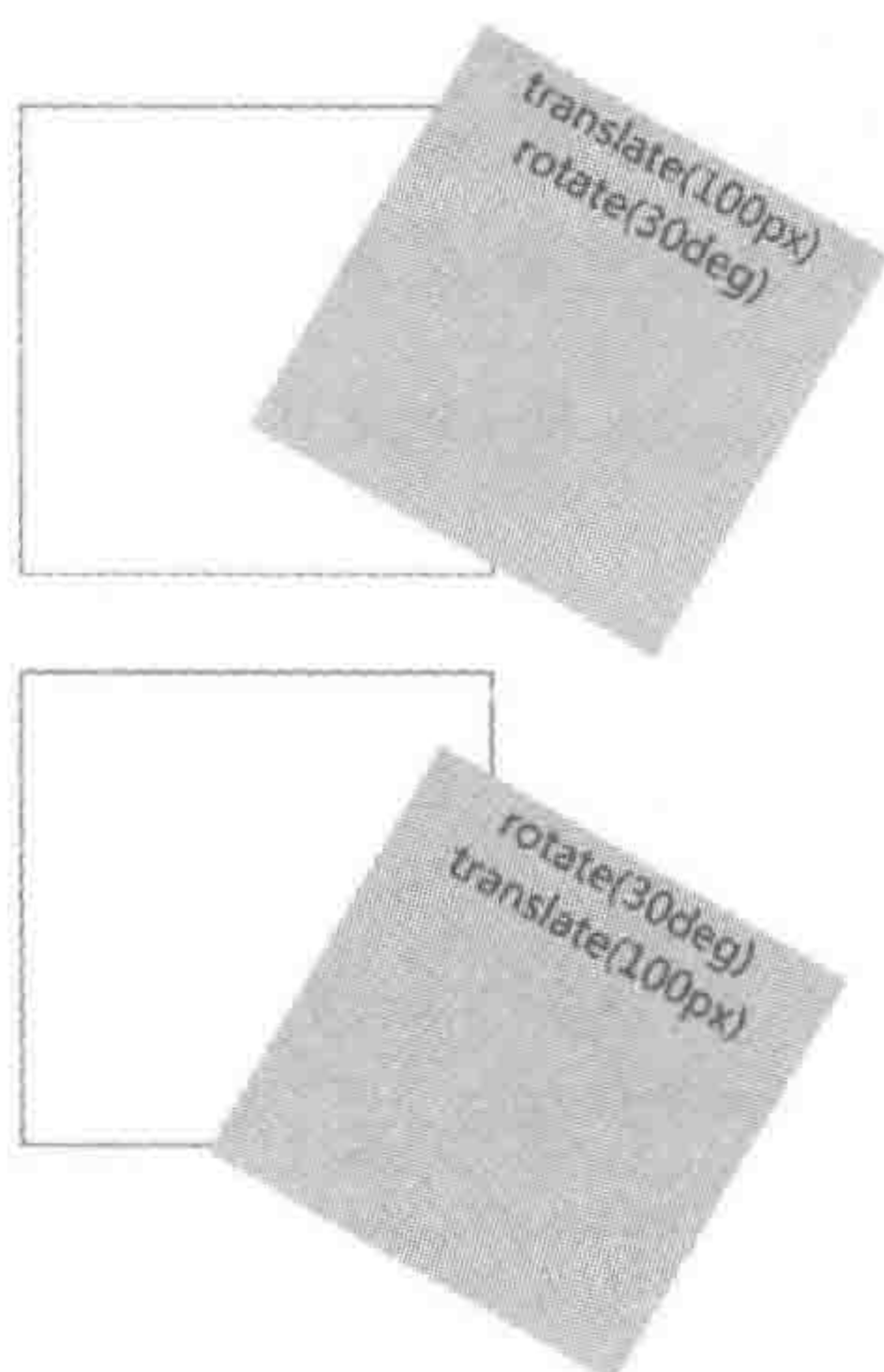
图 16.5 旋转平移——不同变形顺序的显示效果
