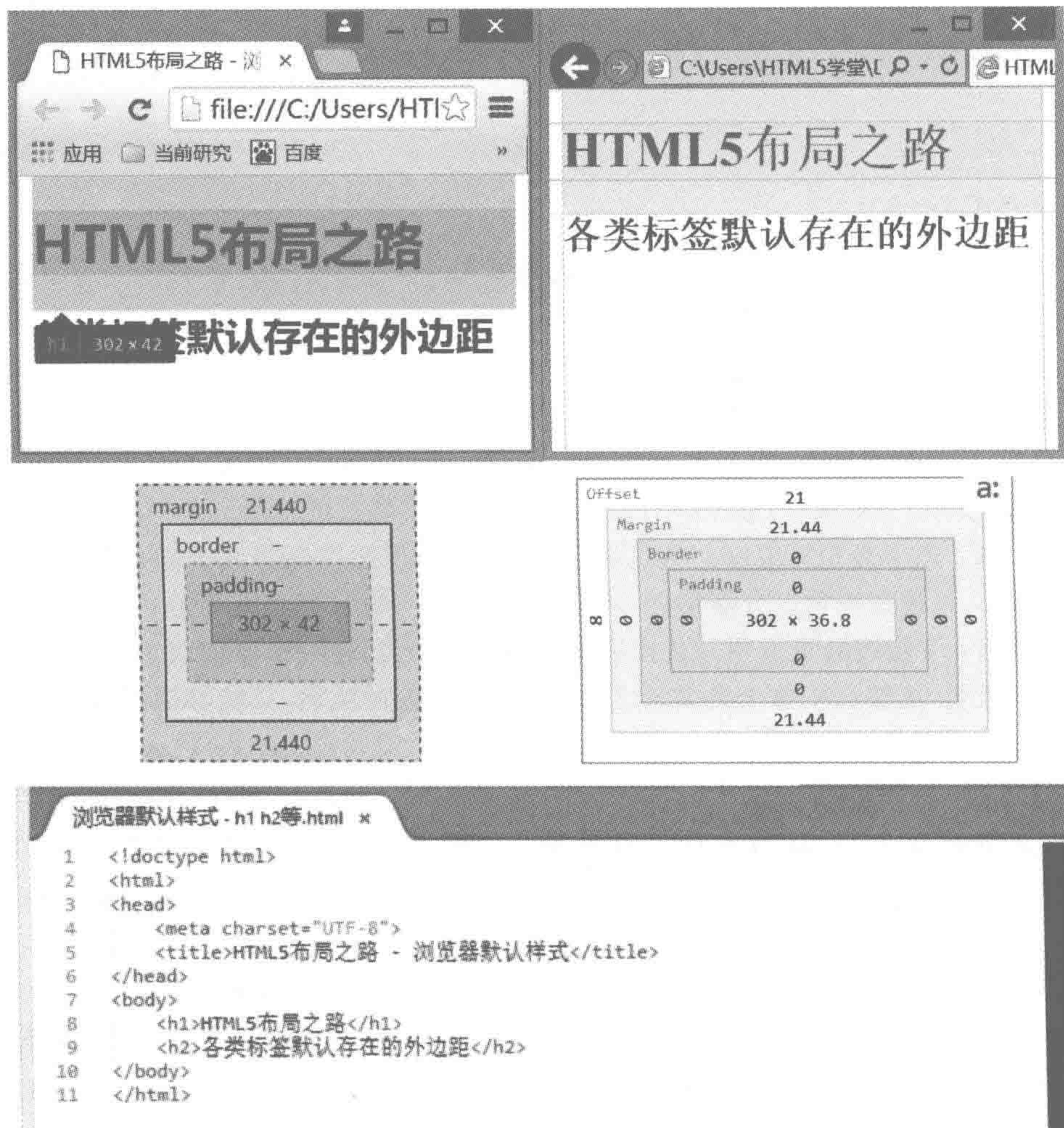
图 3.13 <h1>在各个浏览器中的默认样式
