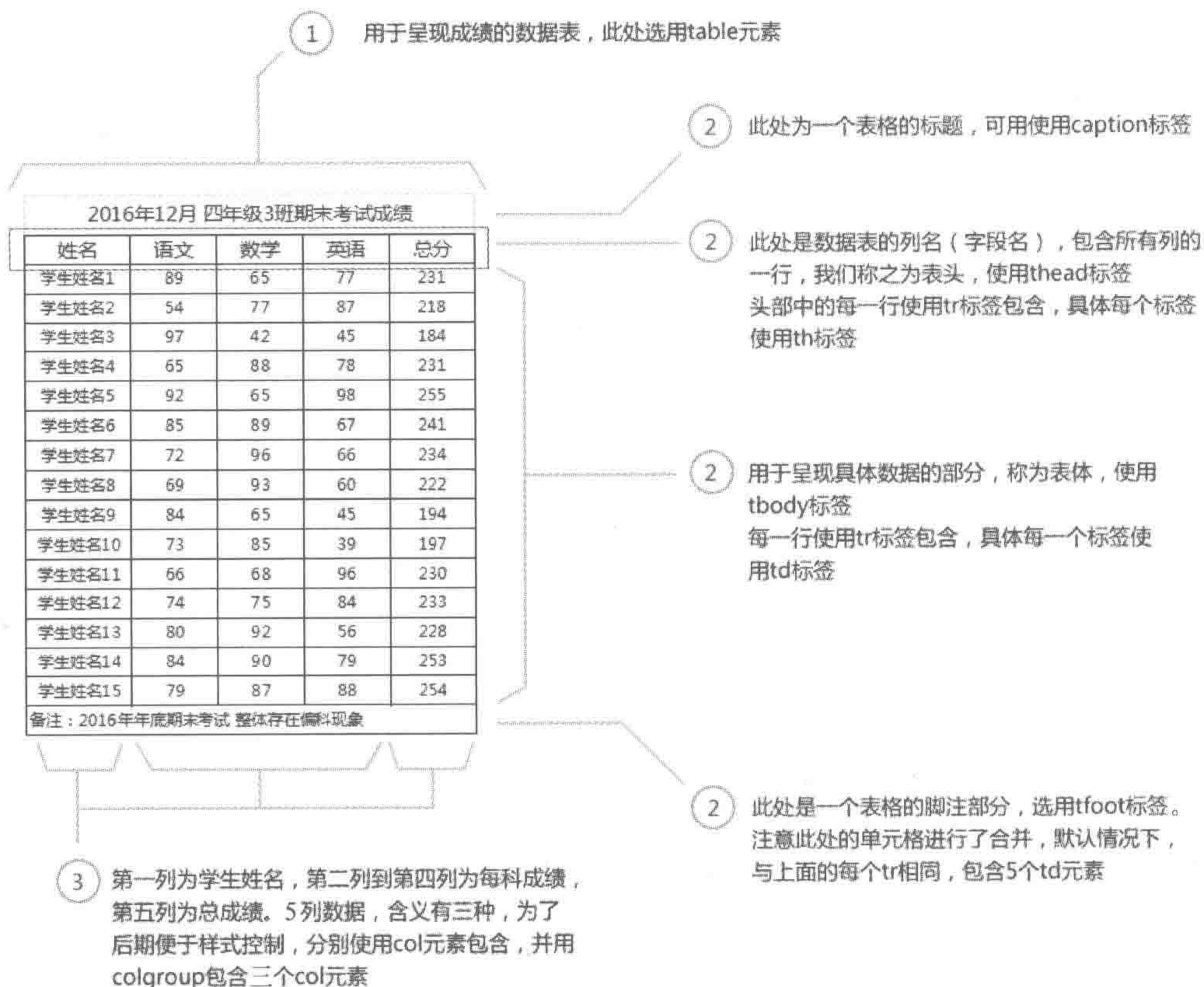
图 10.7 数据表需求分析
