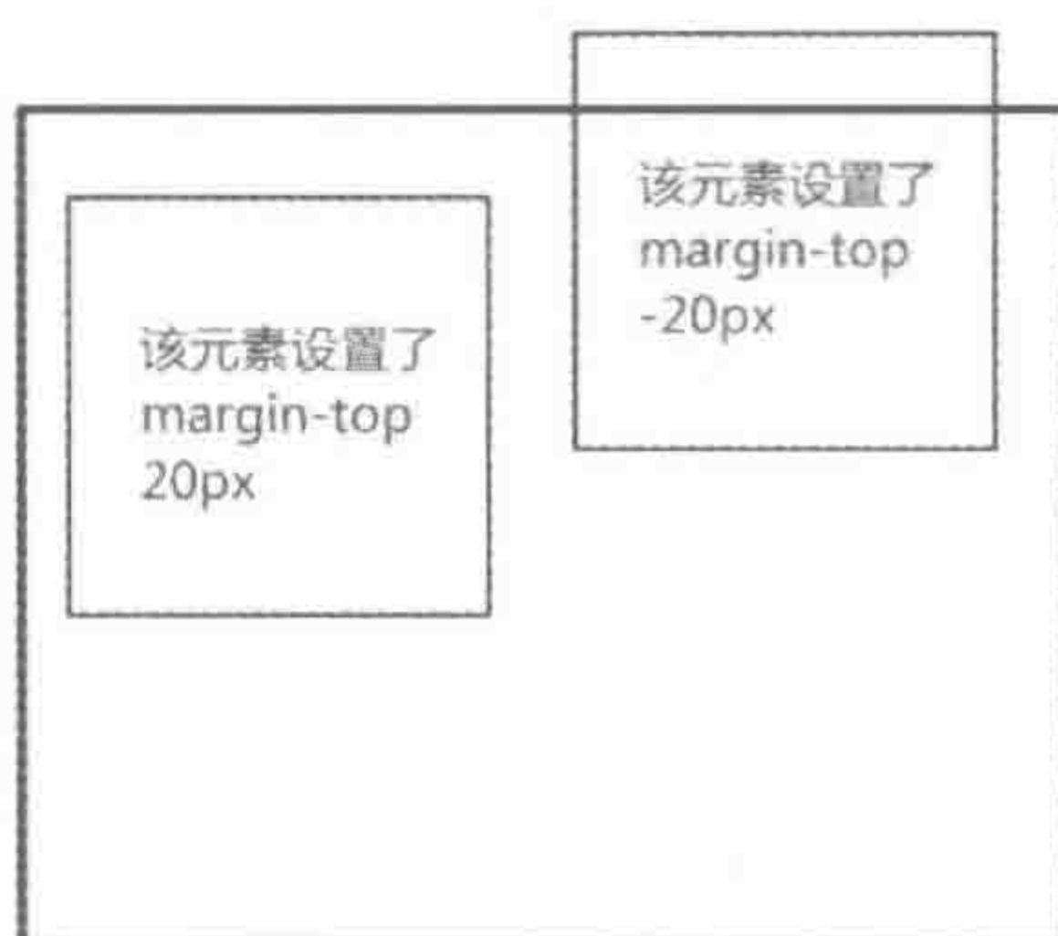
图 3.23 margin 设置负值时的效果
