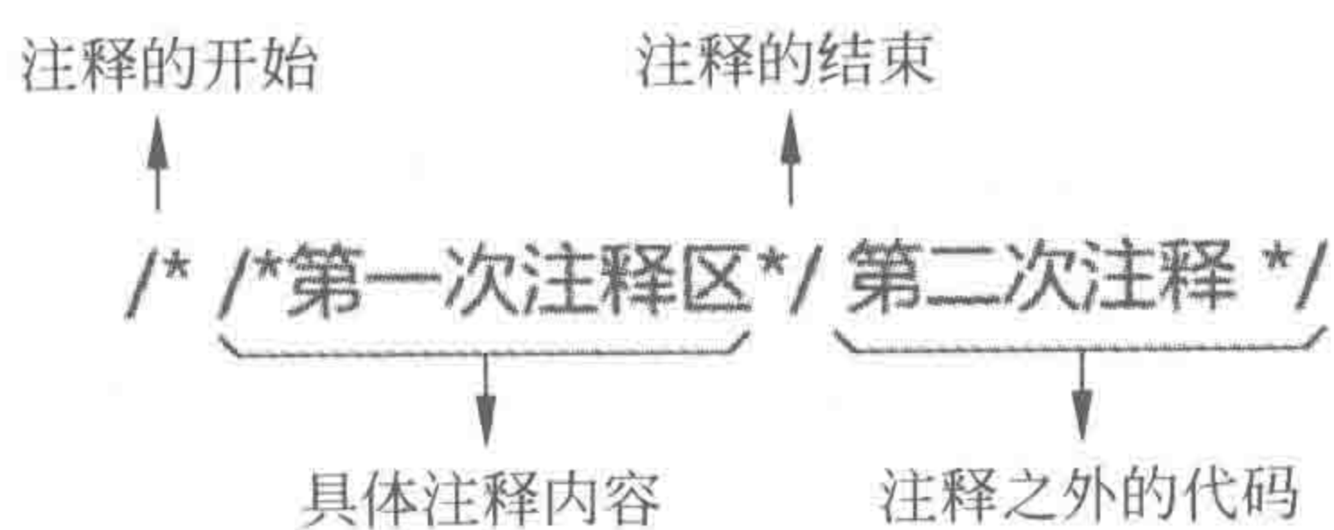
图 3.10 CSS 注释
