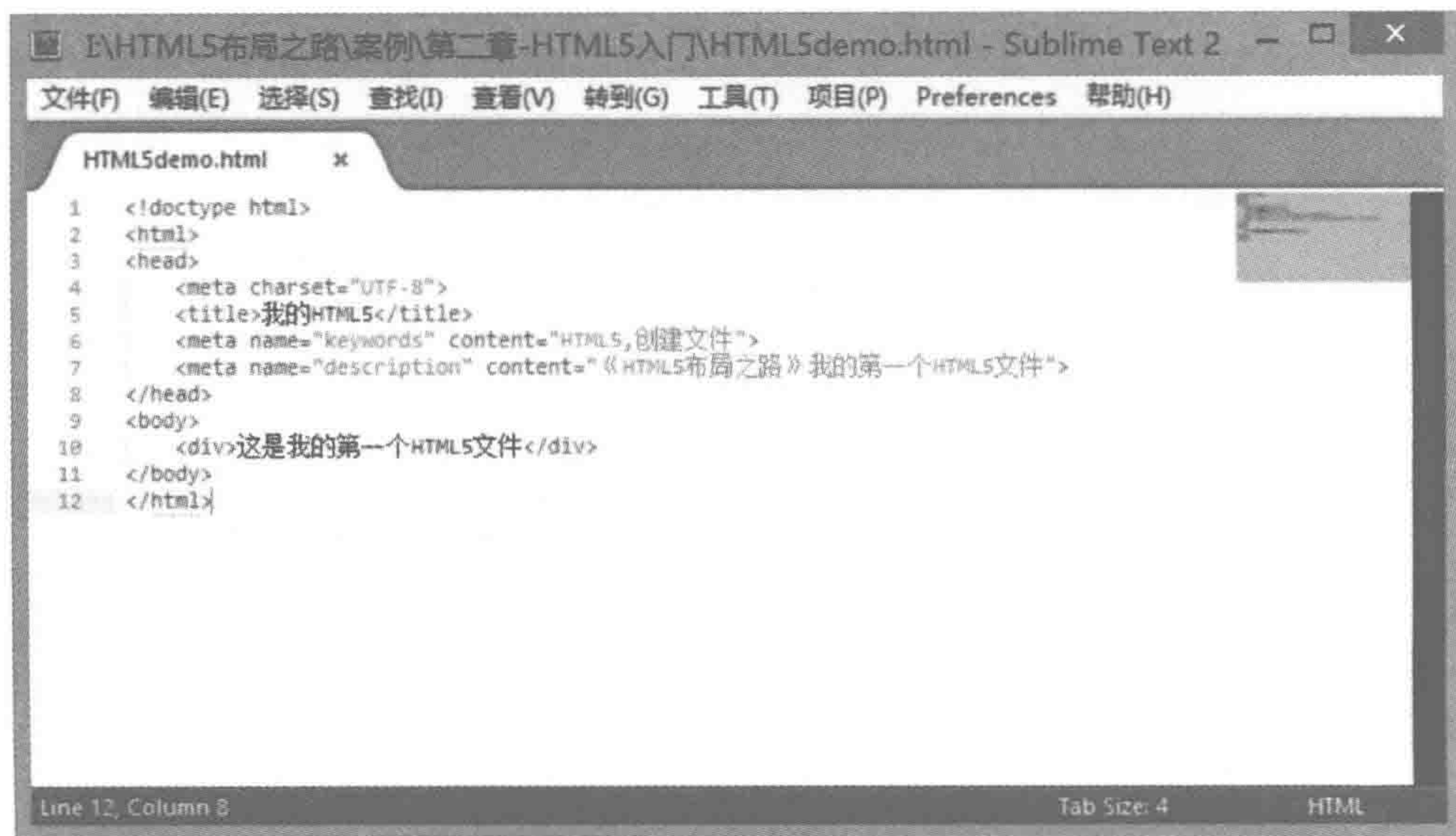
图 1.27 Sublime 界面
