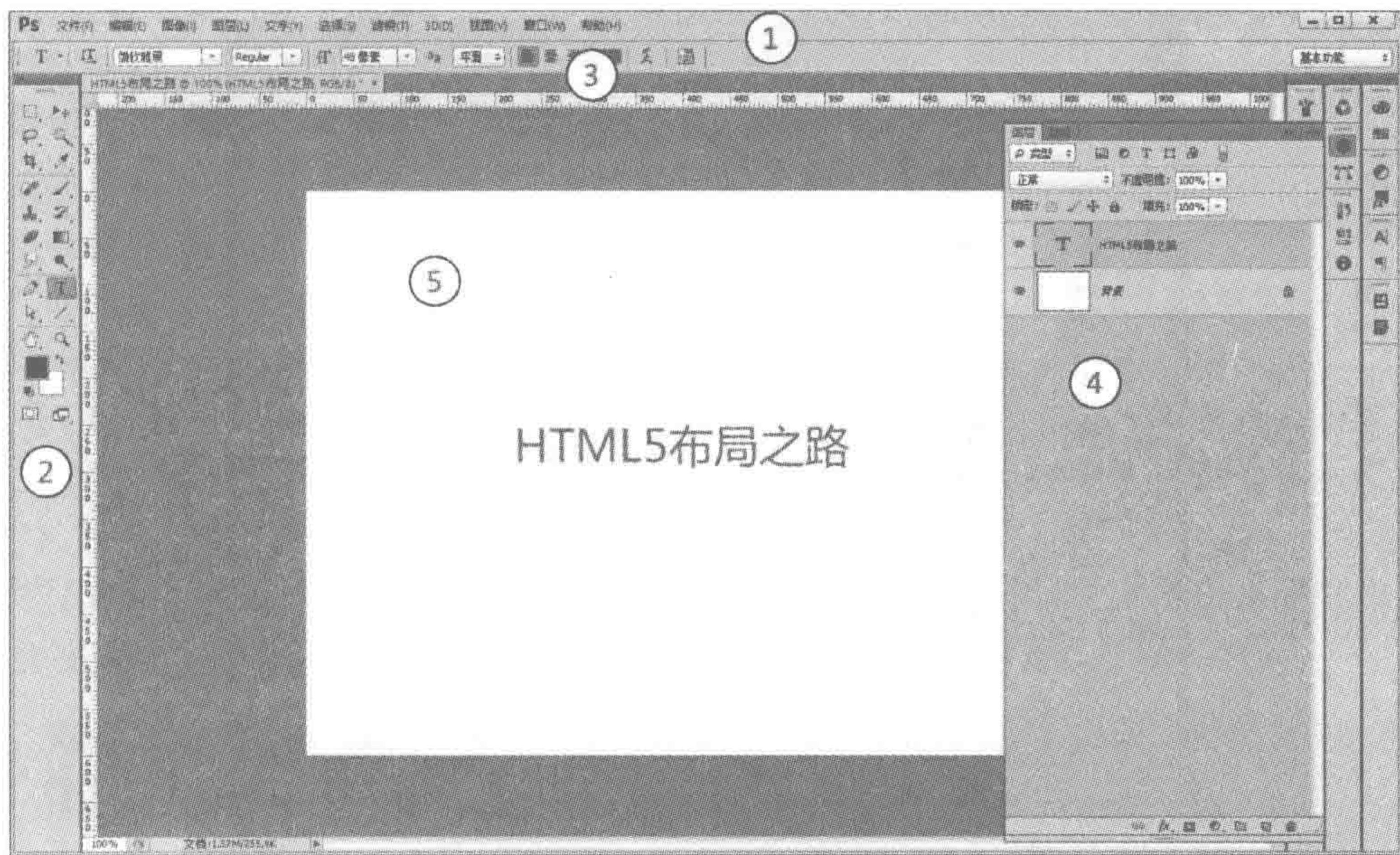
图 1.2 Photoshop 界面
