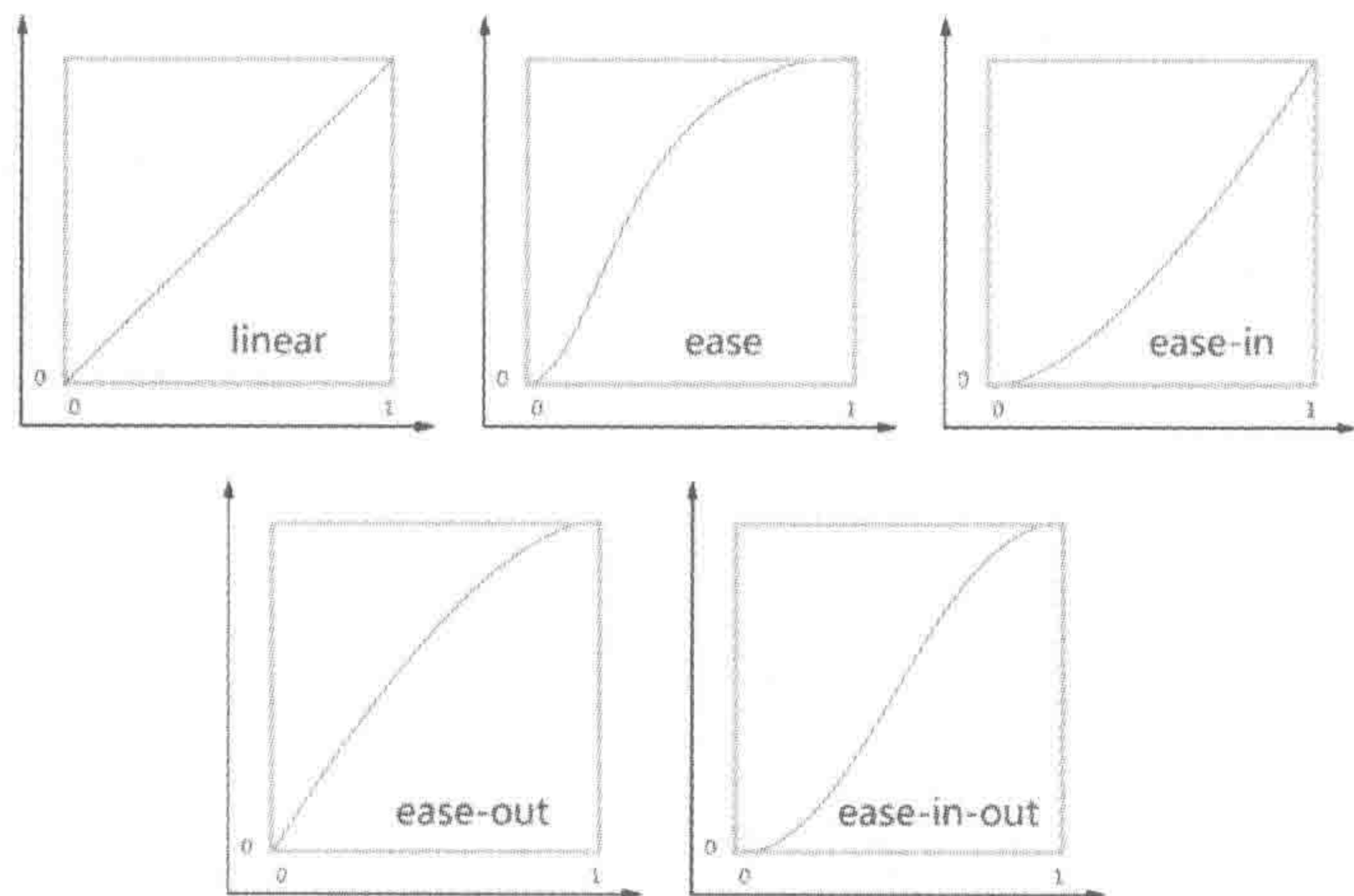
图 16.8 贝塞尔曲线图
