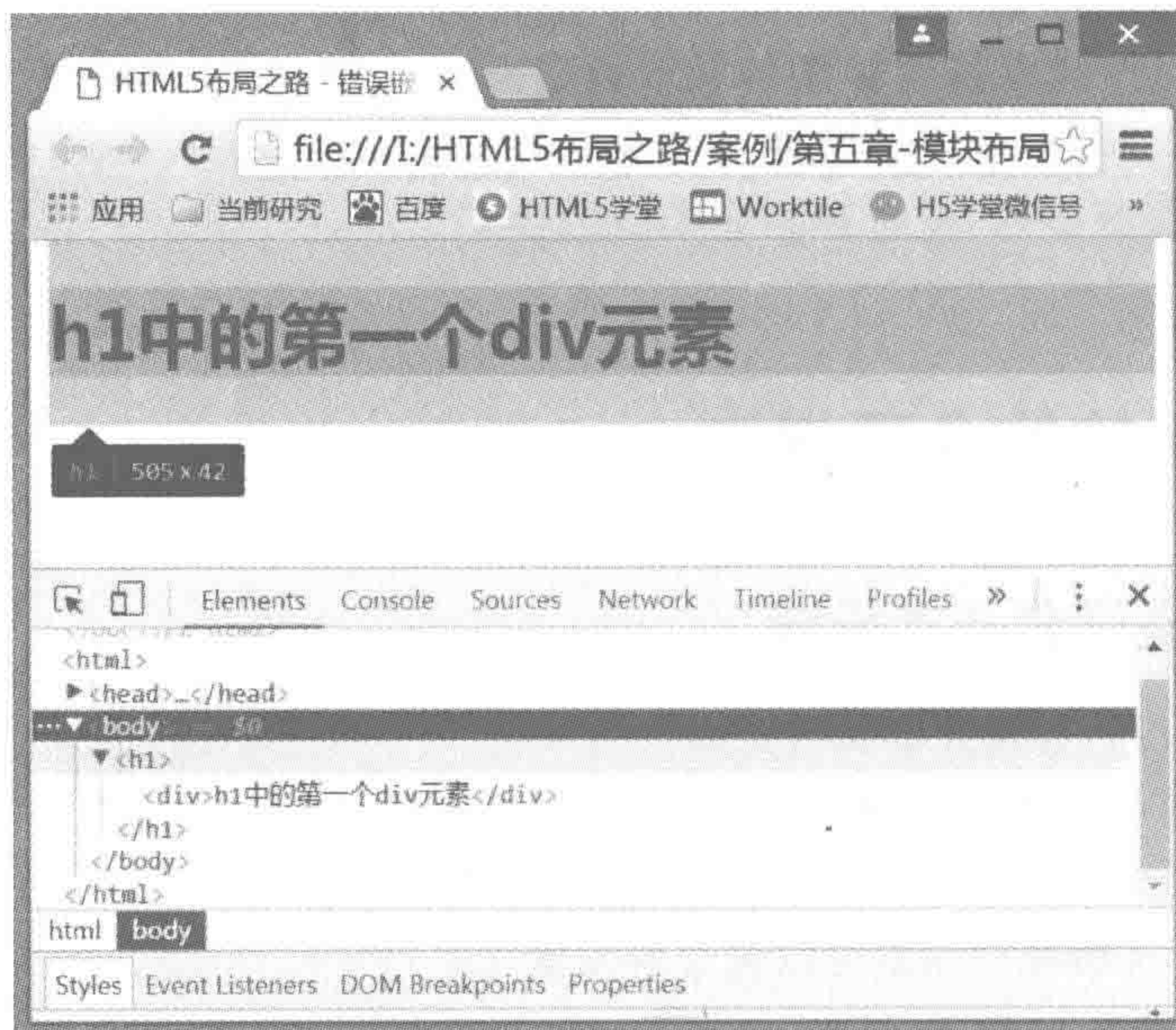
图 5.4 h1 标签中嵌套 div 的显示效果
