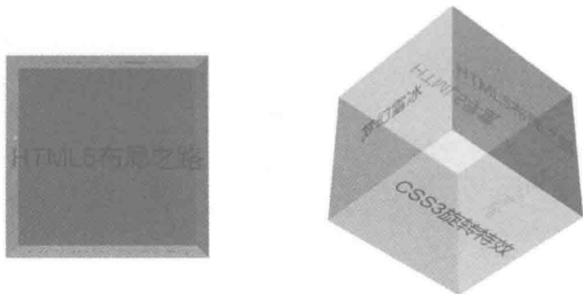
图 18.22 三维立方体
