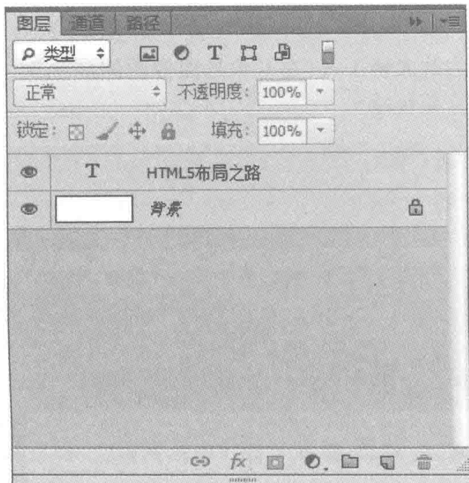
图 1.6 “图层”面板
