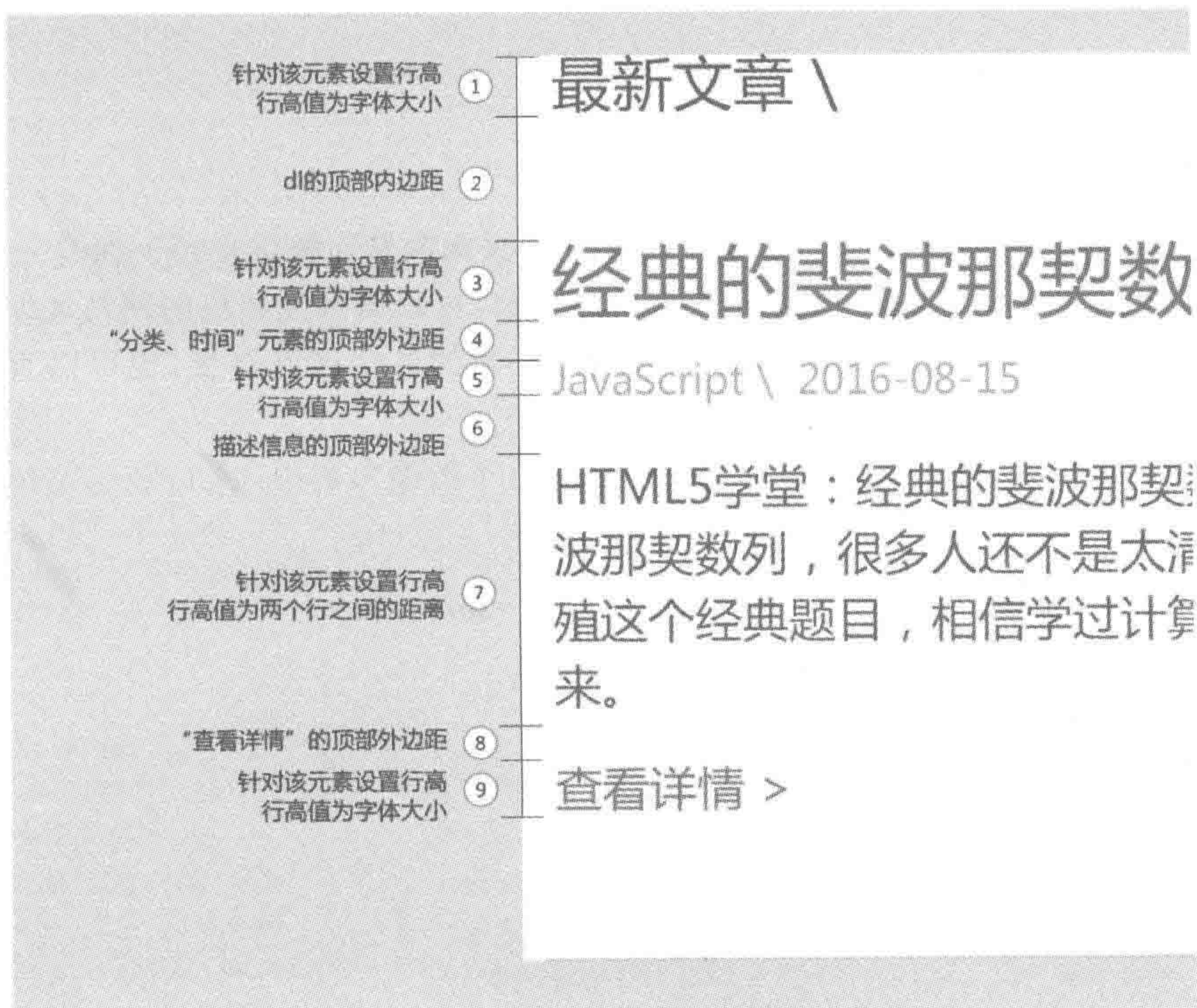
图 19.3 最新文章模块空隙设置方法 1
