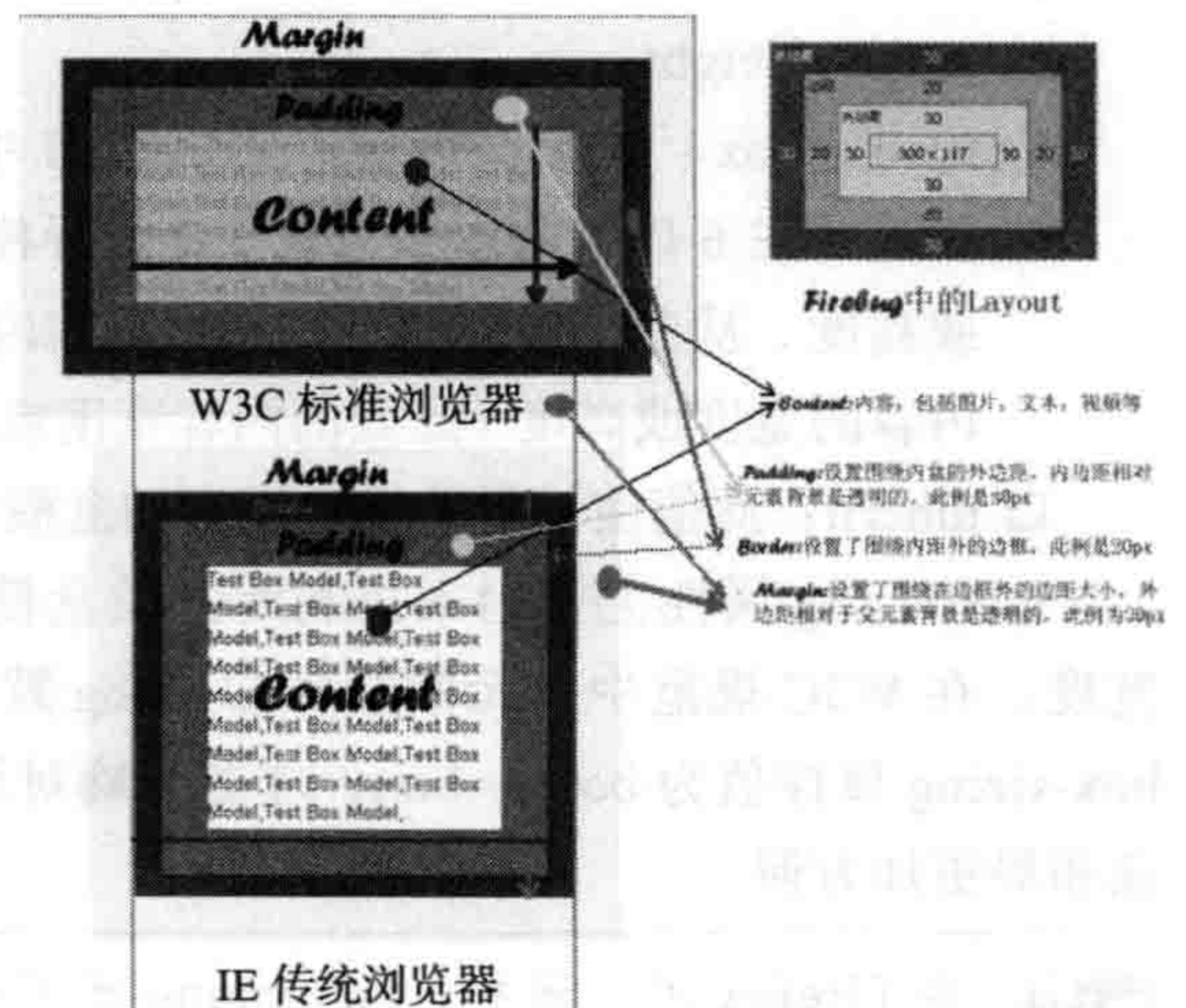
图 7-2 现代浏览器和传统浏览器 layout 截图
