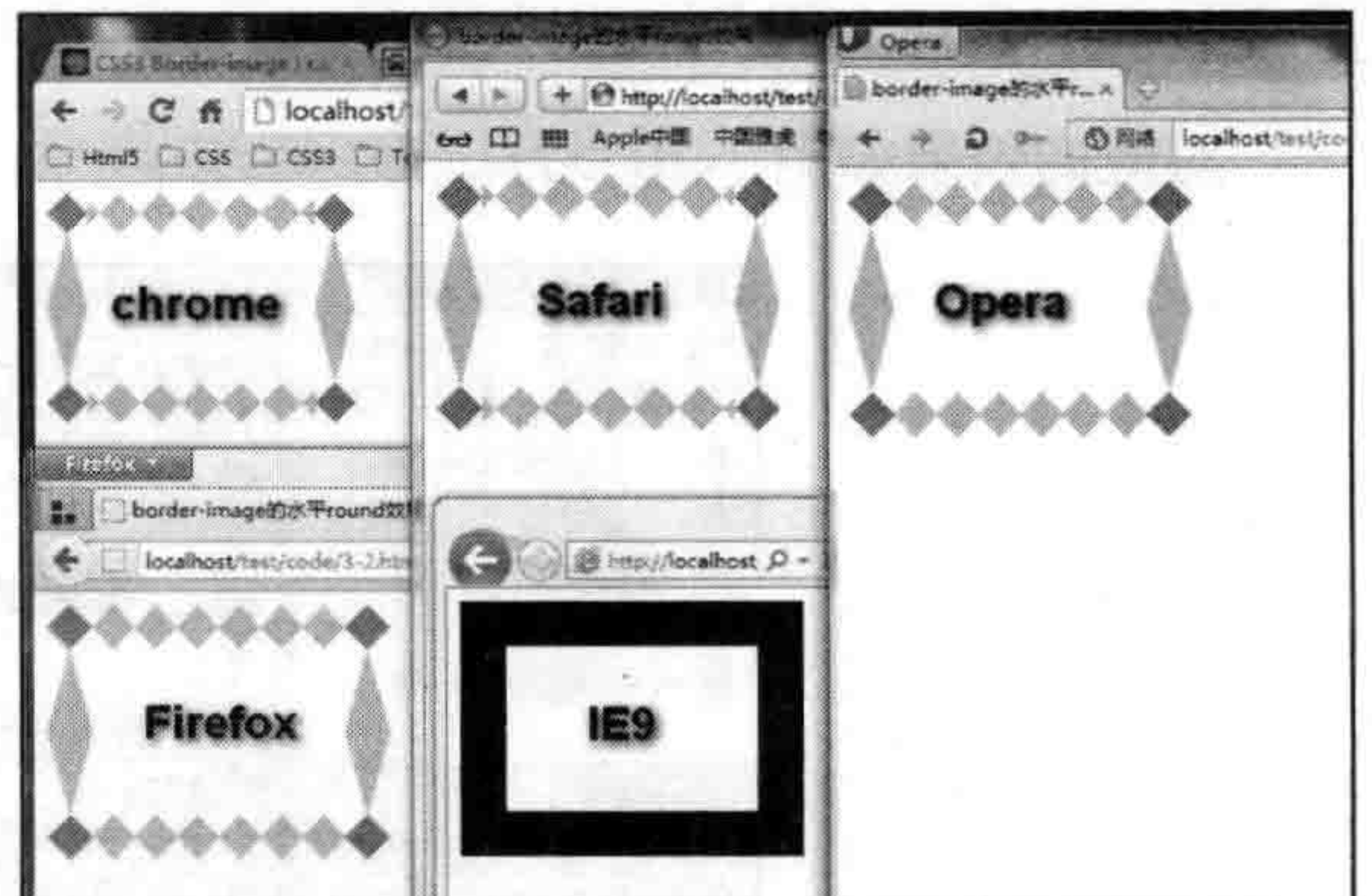
图 3-8 各浏览器下水平 round 演示效果
