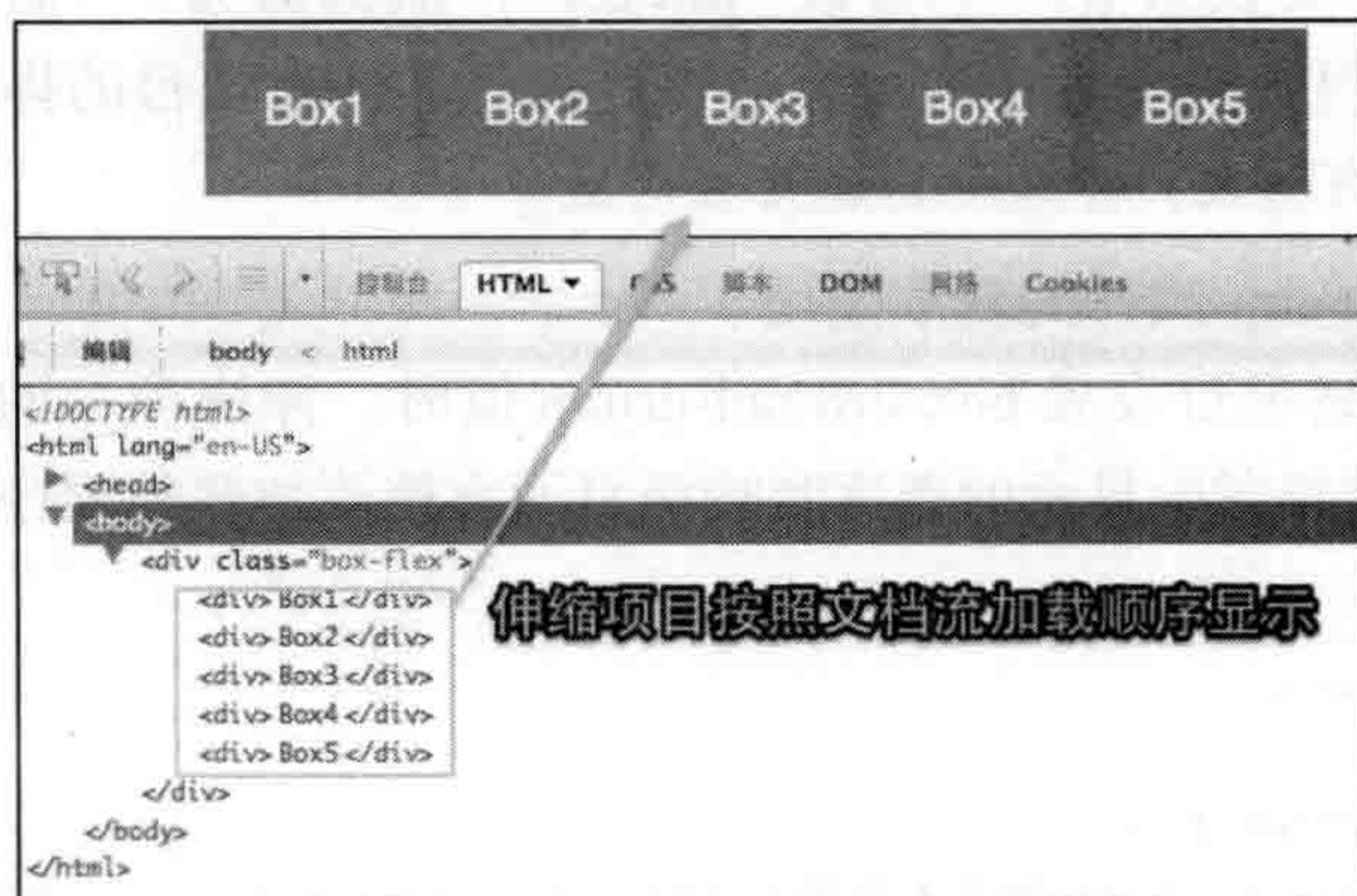
图 8-21 伸缩项目未显式设置 box-ordinal-group 值的效果
