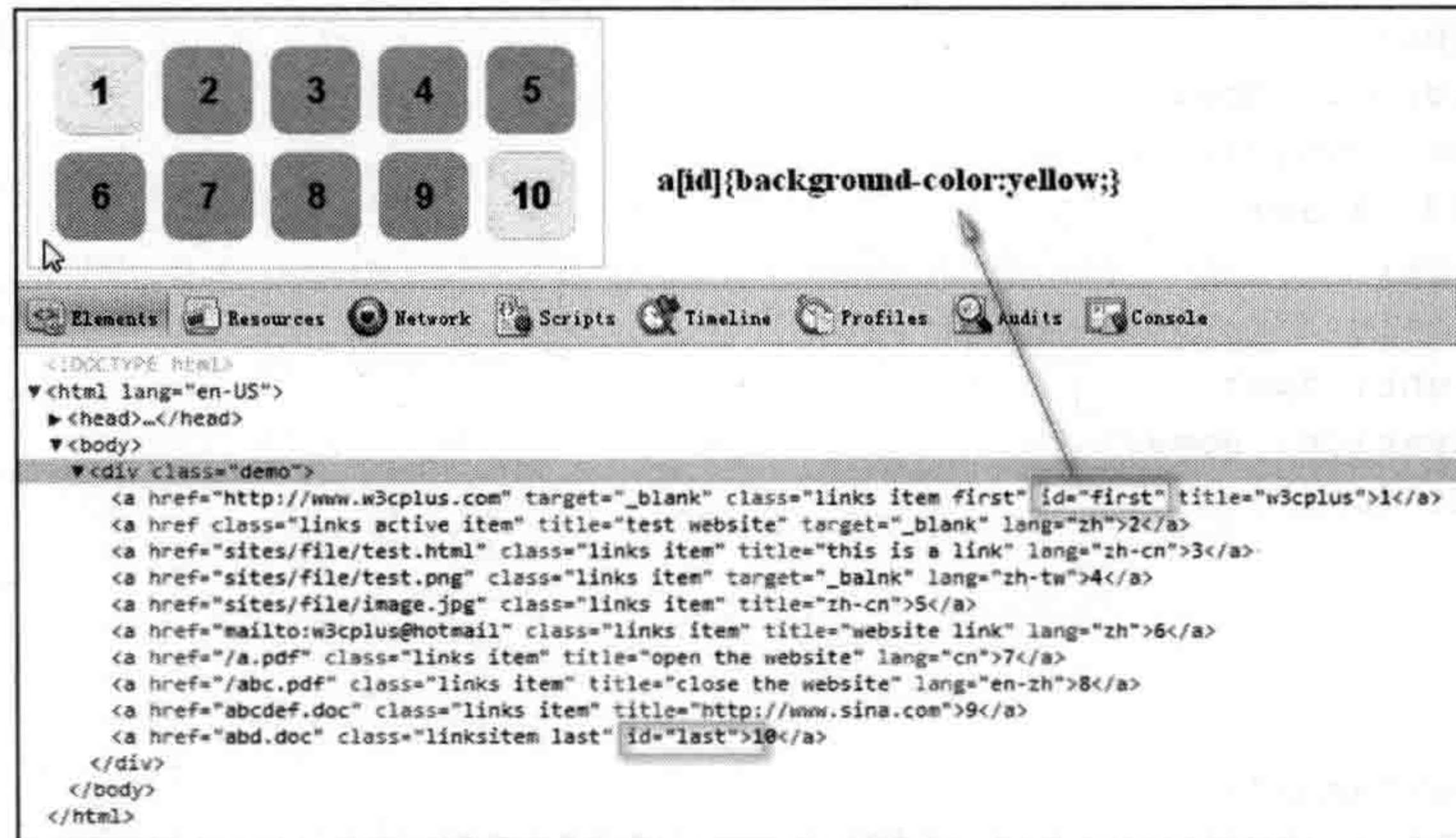
图 2-54 E[attr] 属性选择器的效果
