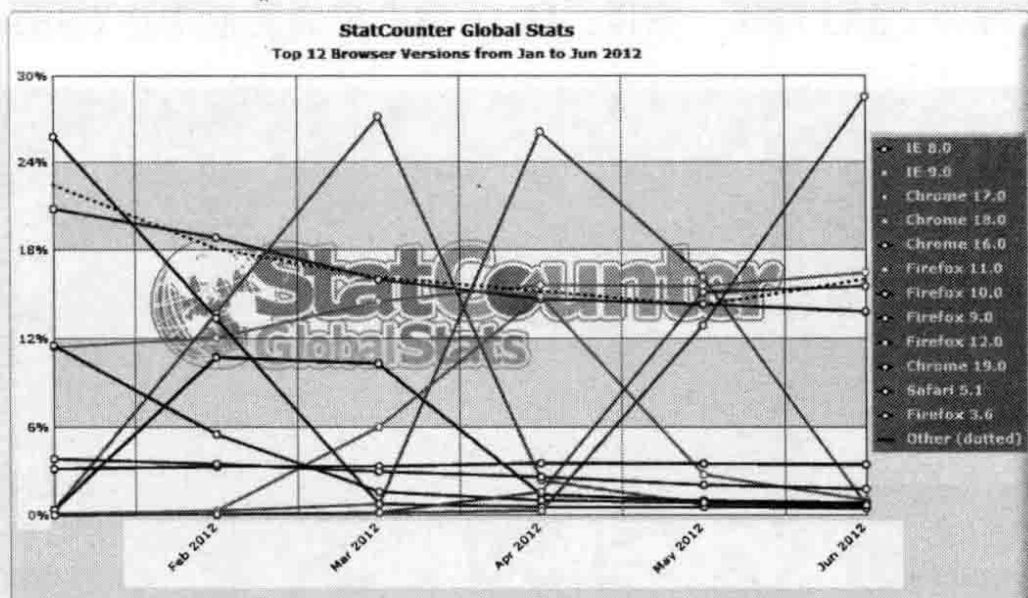
图 1-4 主流浏览器市场份额（2012 年 1 月～2012 年 6 月）
