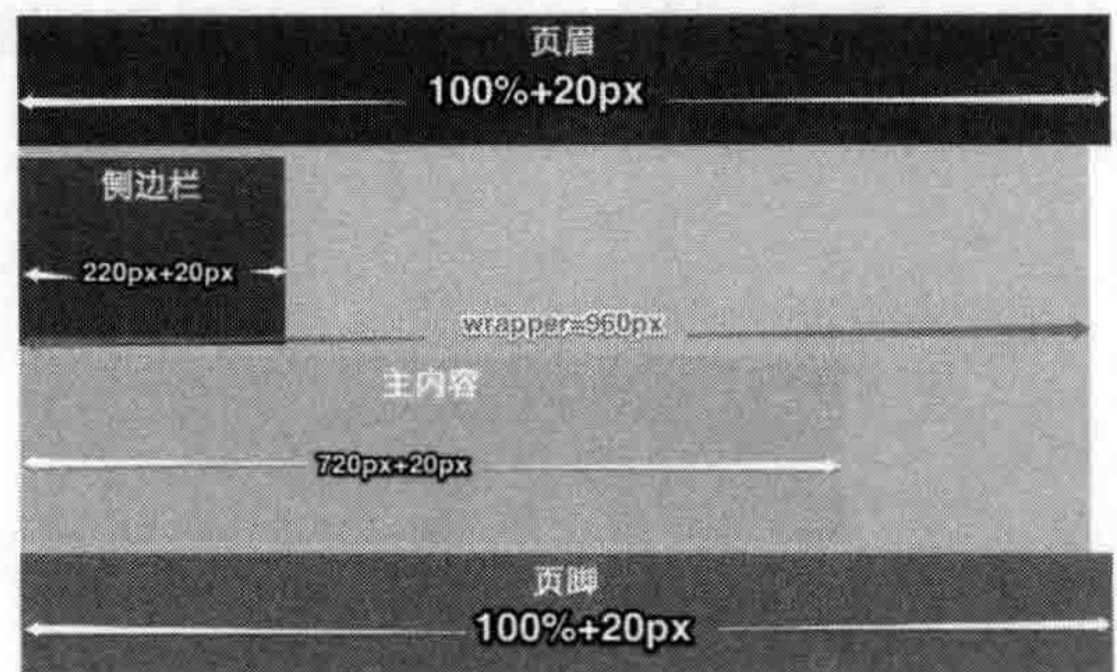
图 7-5 内距打破布局的效果
