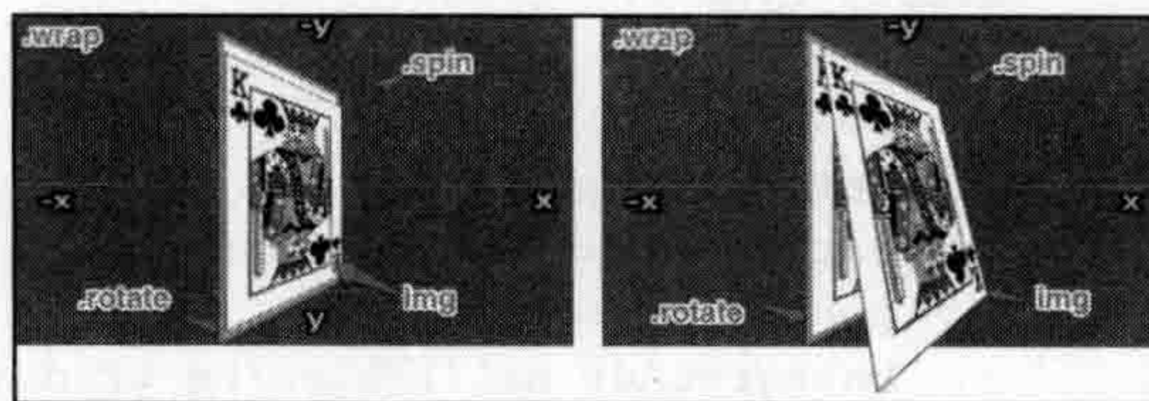
图 11-9 transform-style 设置 flat (左) 和 preserve-3d (右) 的旋转位移效果
