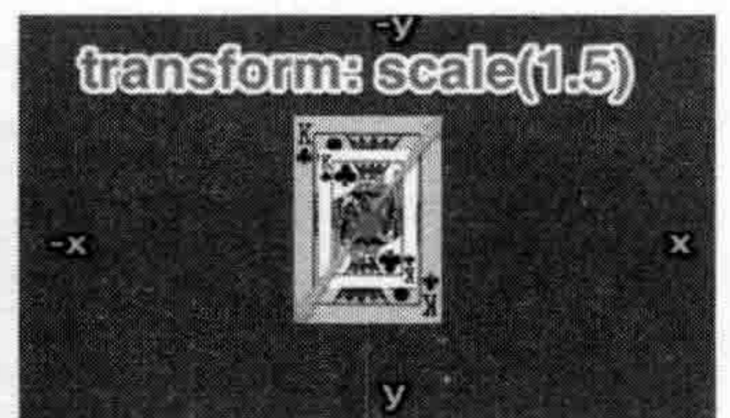
图 11-27 scale() 函数放大元素
