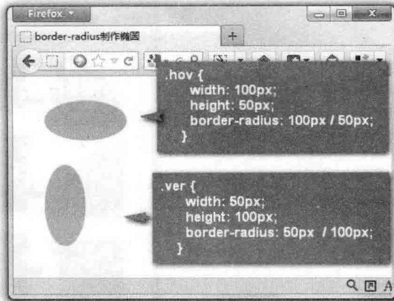
图 3-37 border-radius 制作椭圆
