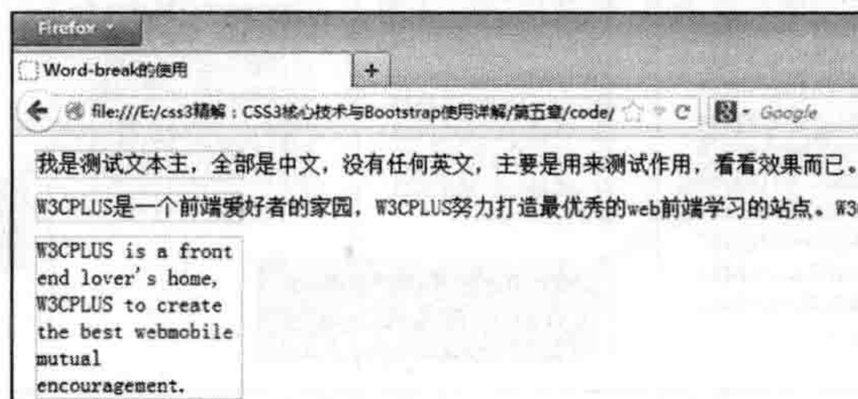
图 5-11 word-break:keep-all 在 Firefox 下效果
