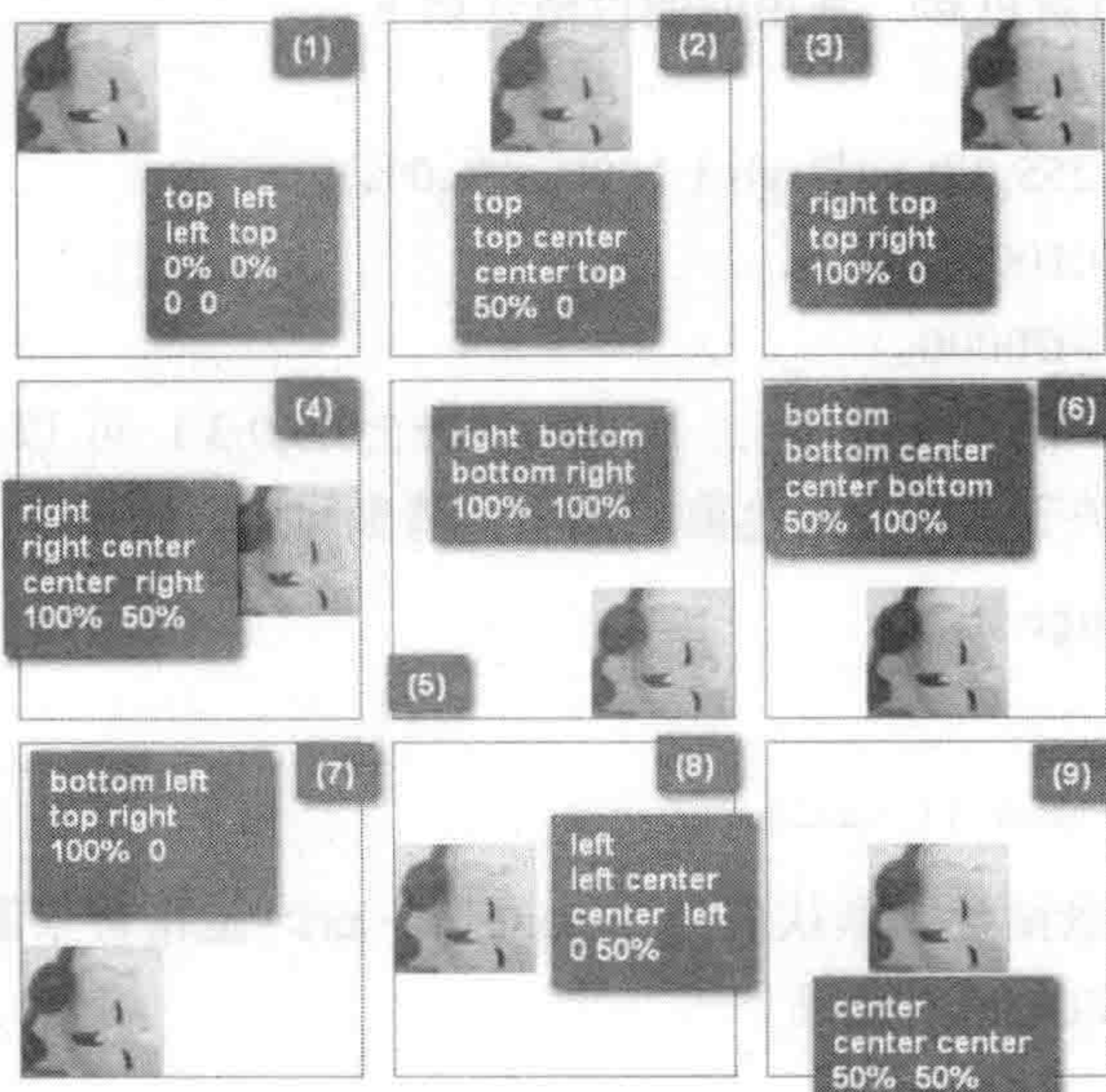
图 4-1 background-position 演示效果
