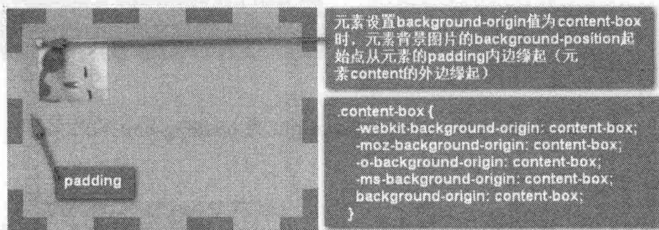
图 4-5 元素设置 background-origin 值为 content-box 的效果
