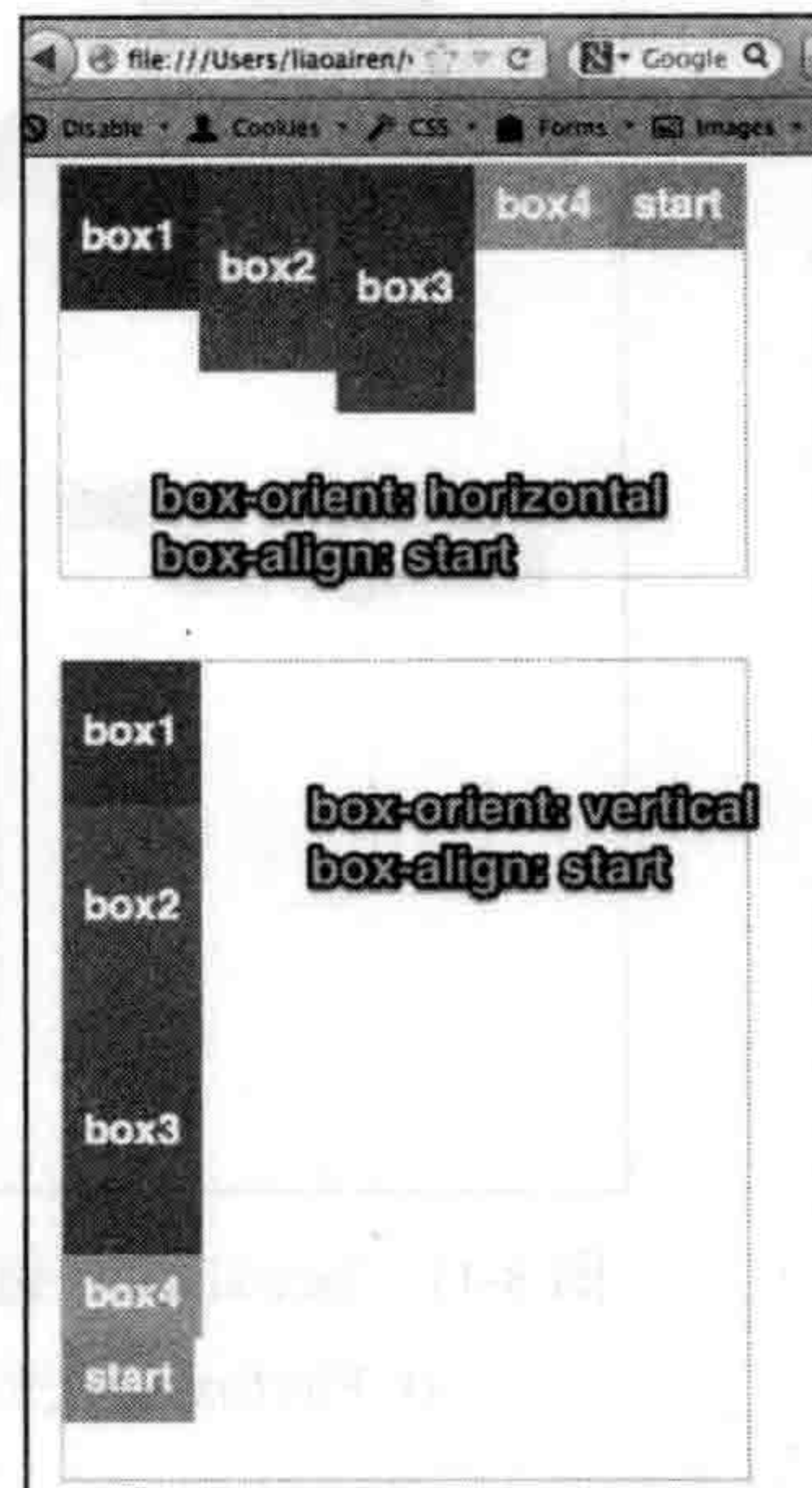
图 8-10 box-align 取值为 start 在 Firefox 的效果
