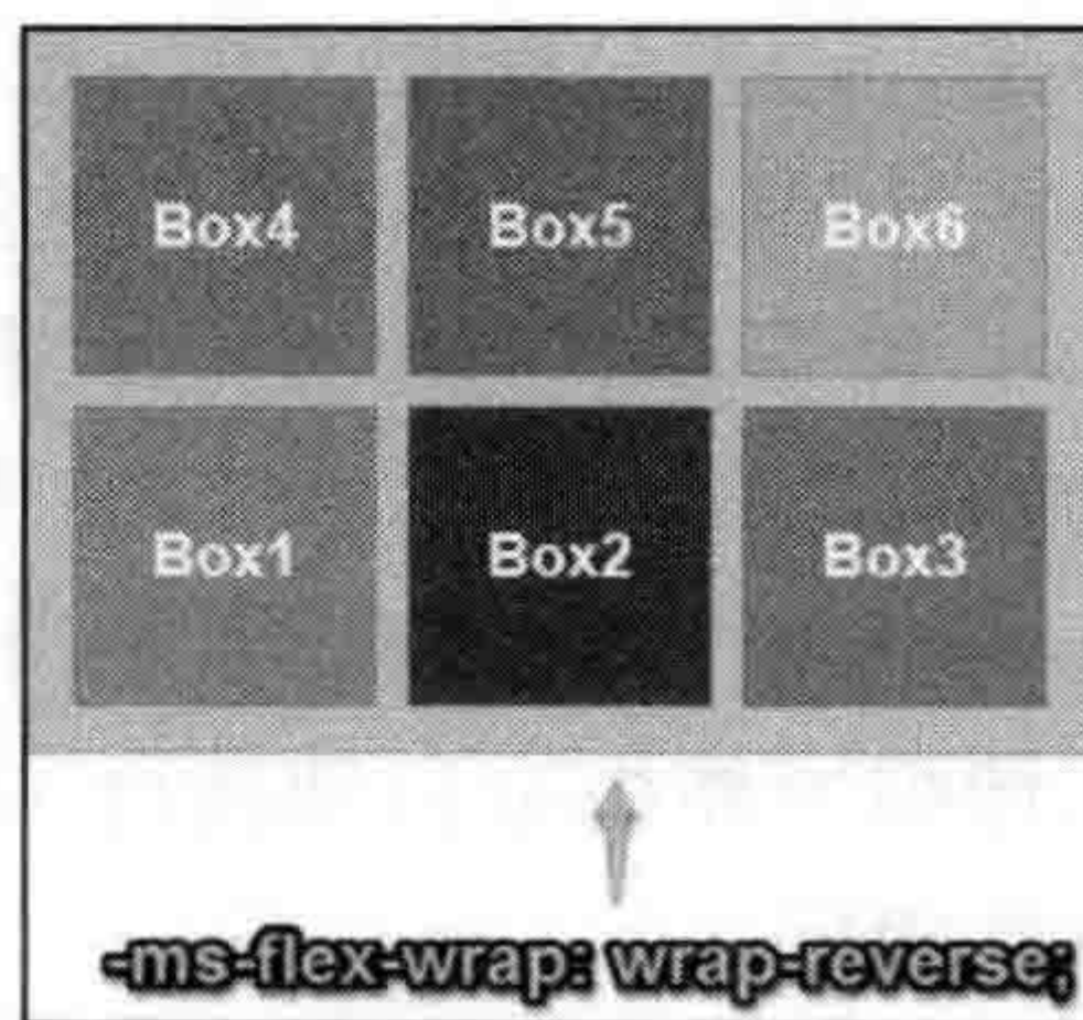
图 8-33 flex-wrap 取值为 wrap-reverse 的效果
