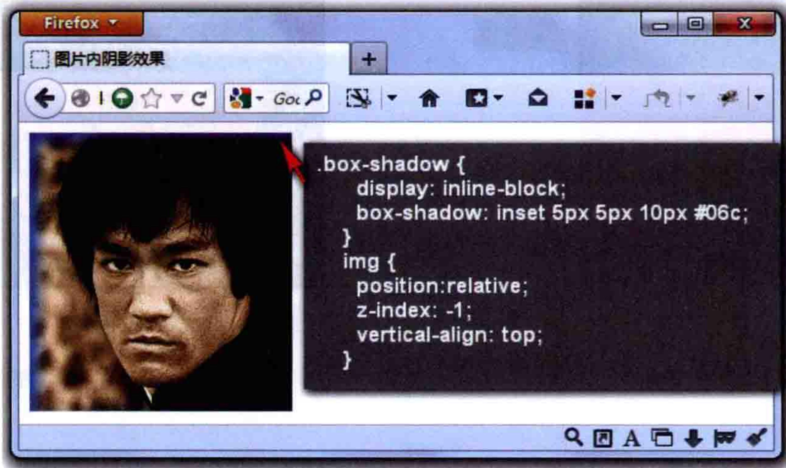
图 3-49 图片内阴影效果
