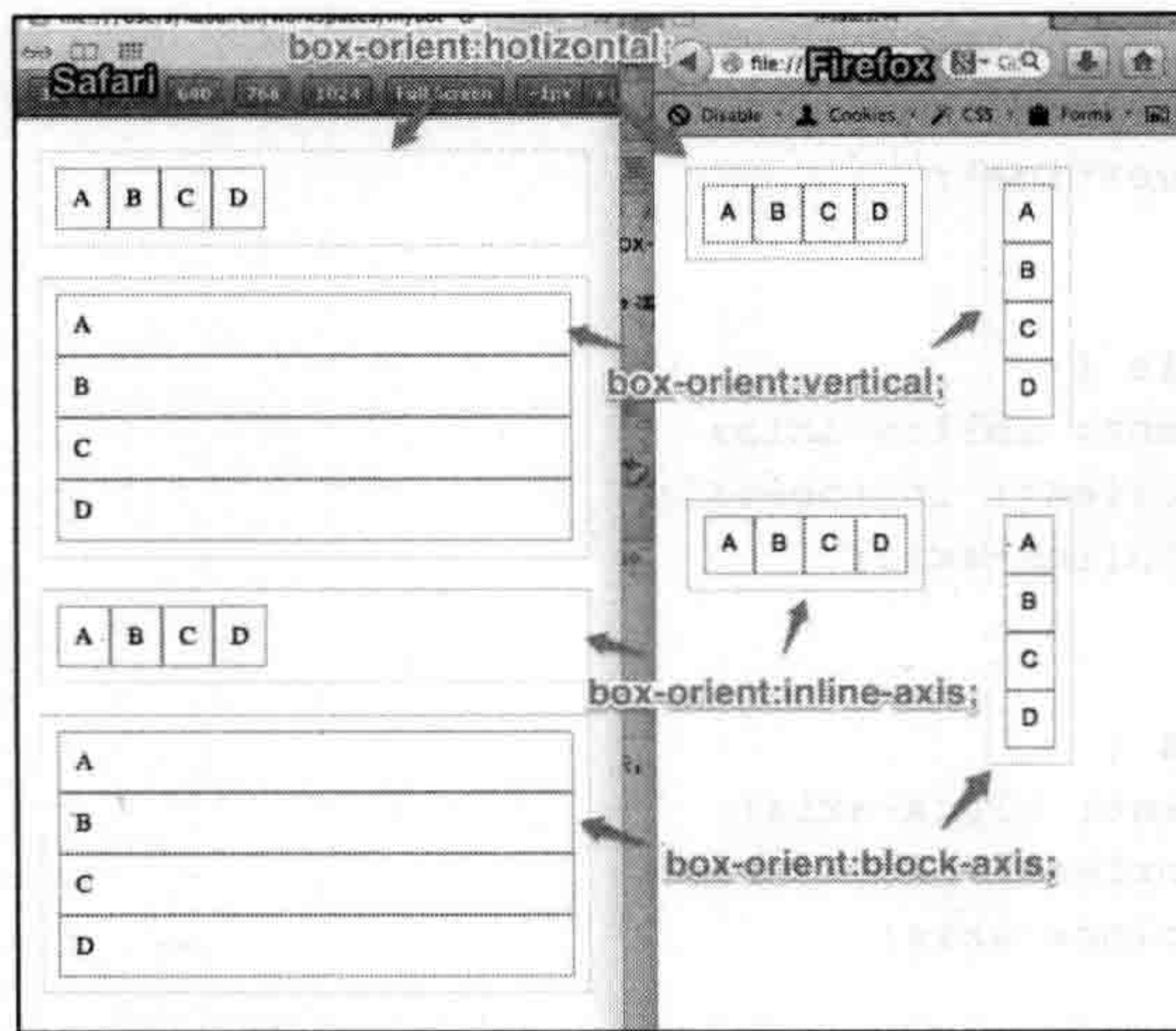
图 8-3 box-orient 在 Safari 和 Firefox 下的效果
