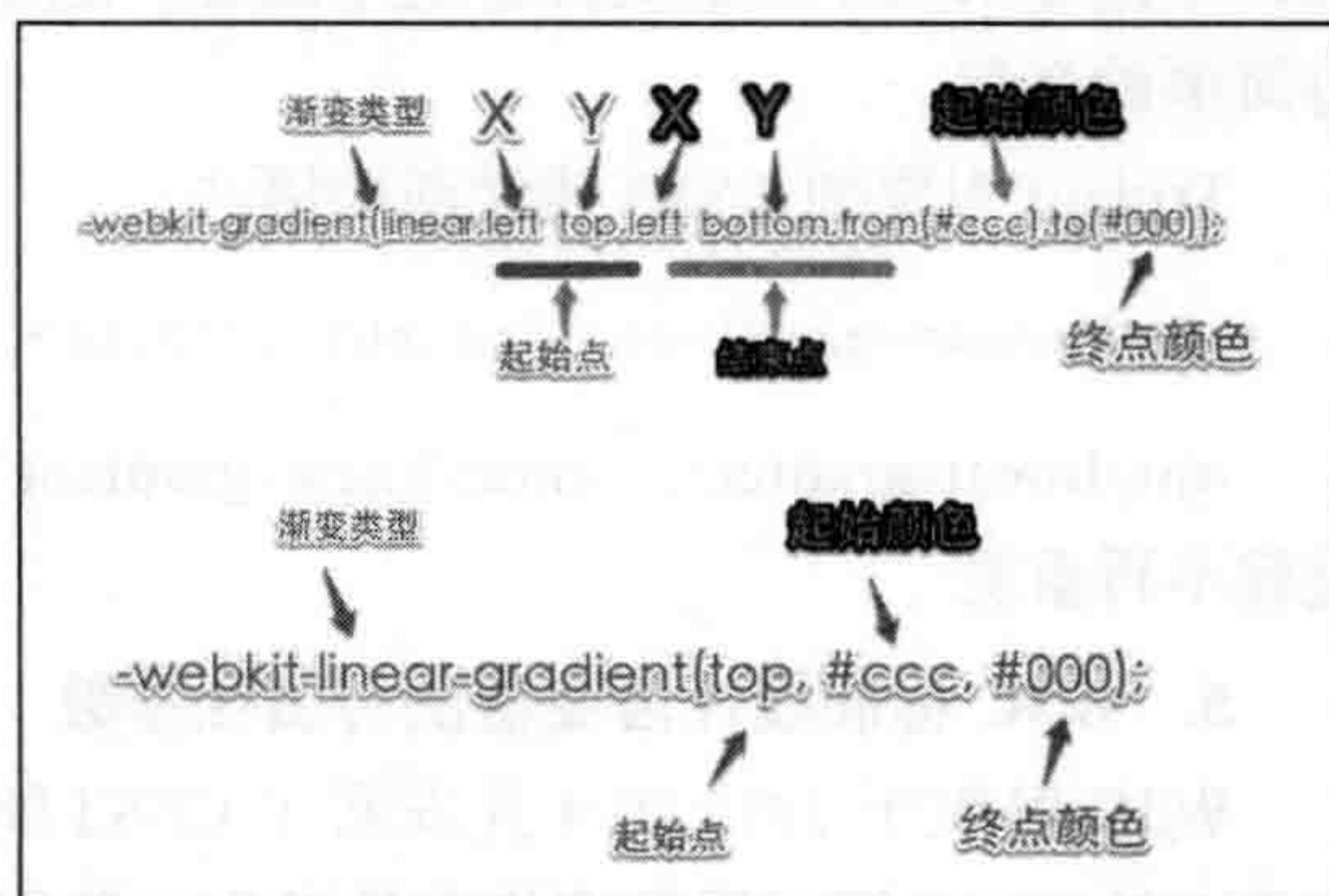
图 10-2 webkit 引擎的线性渐变语法
