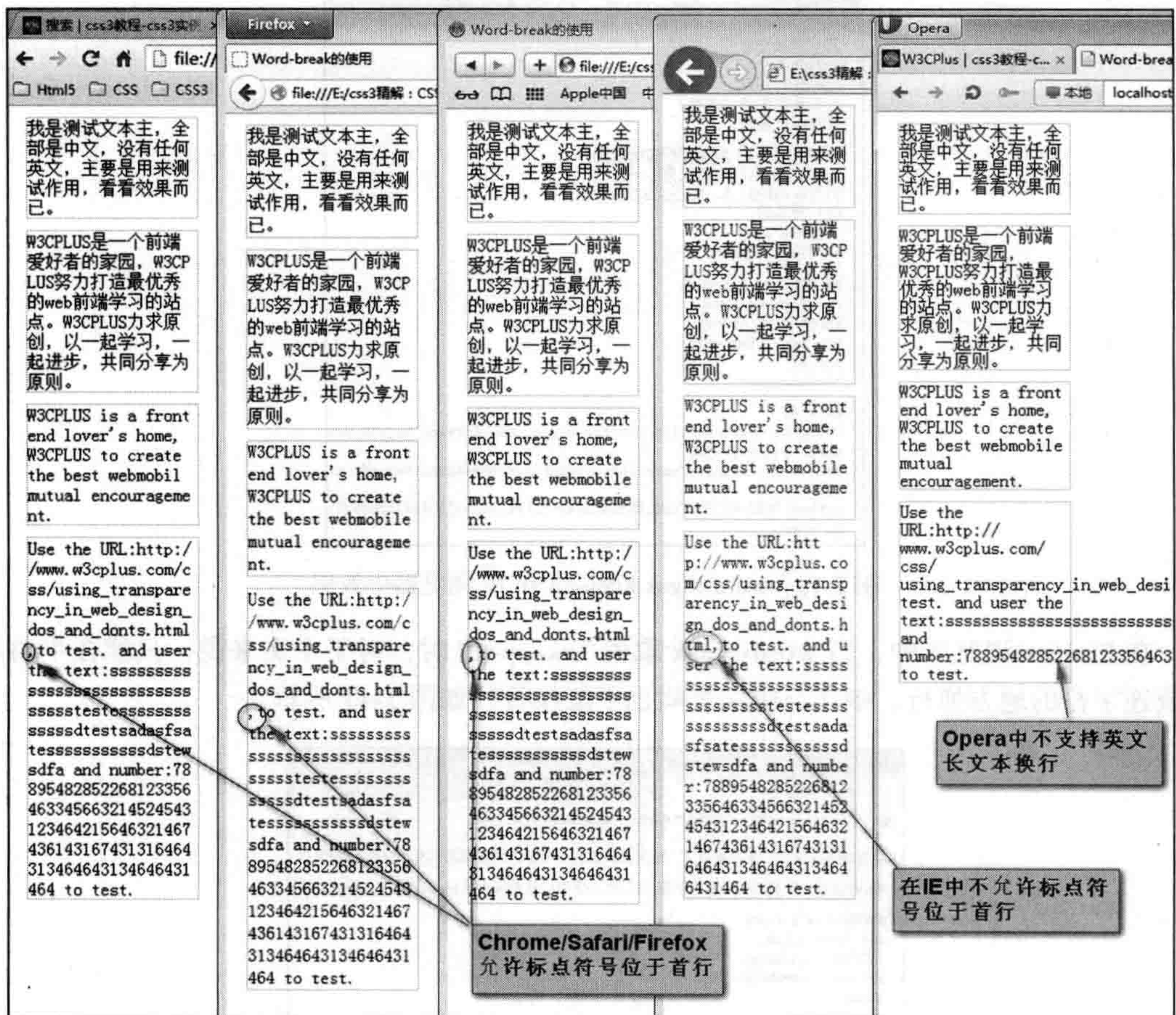
图 5-12 word-break: break-all 各浏览器下效果
