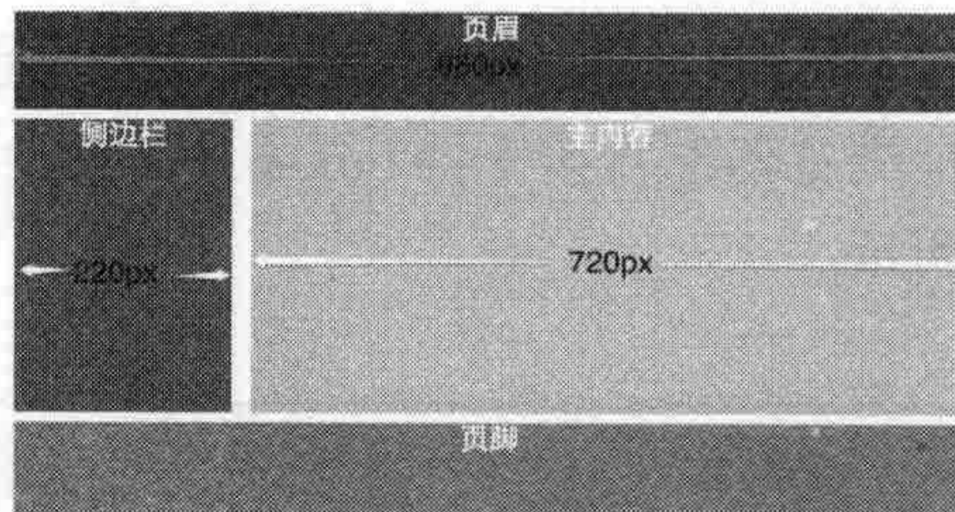
图 7-4 960px 固定两栏居中布局效果
