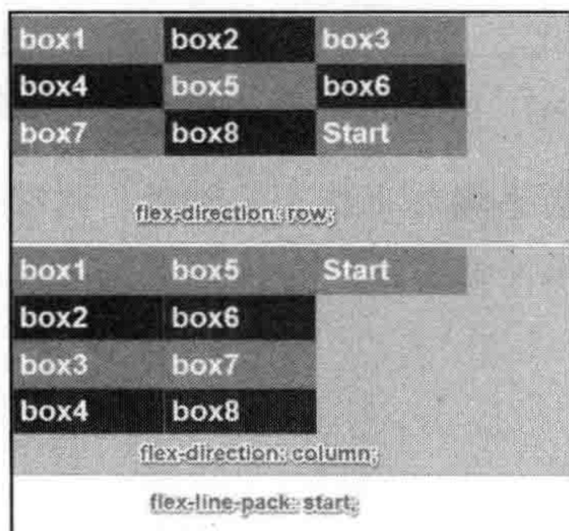
图 8-44 flex-line-pack 取值为 start 的效果
