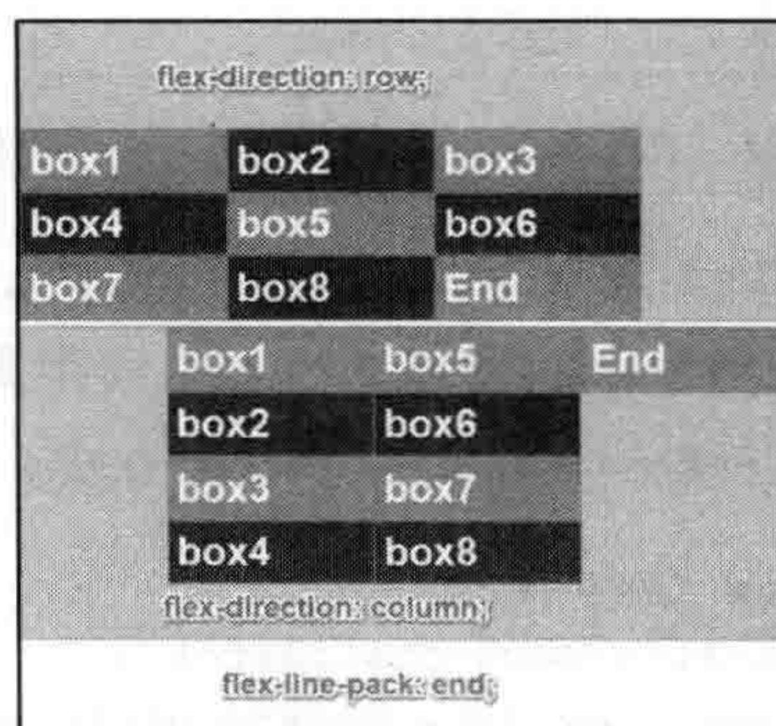
图 8-45 flex-line-pack 取值为 end 的效果
