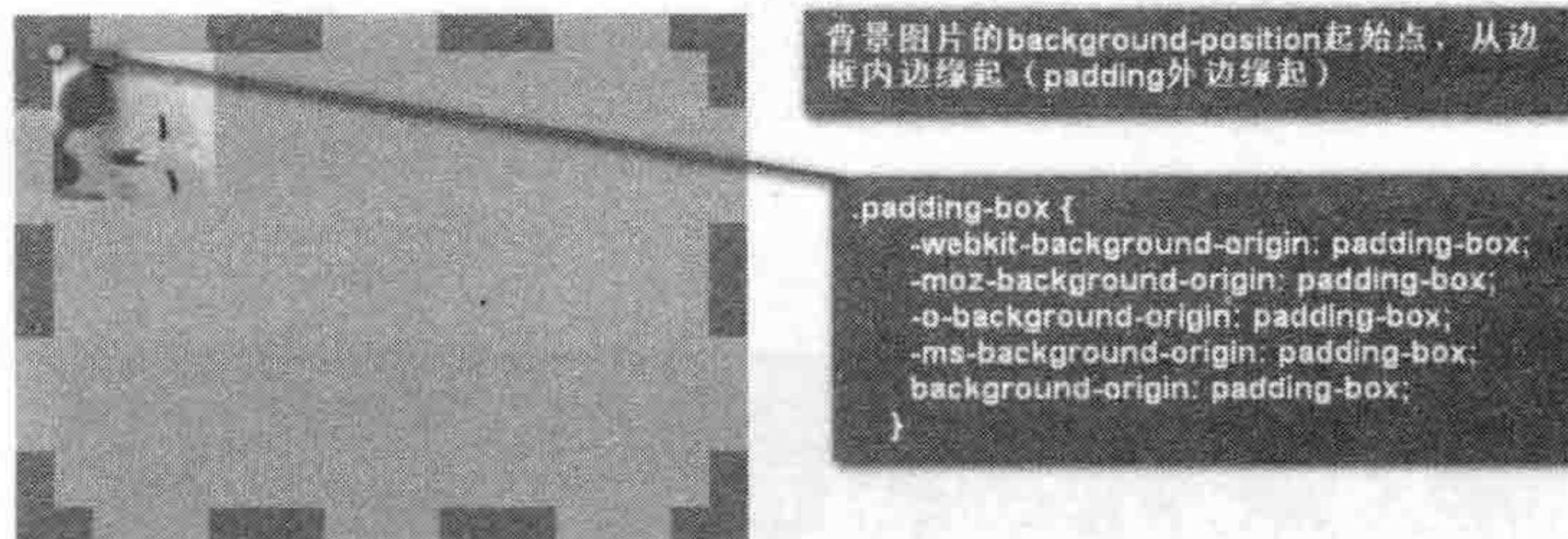
图 4-3 元素设置 background-origin 为 padding-box 的效果
