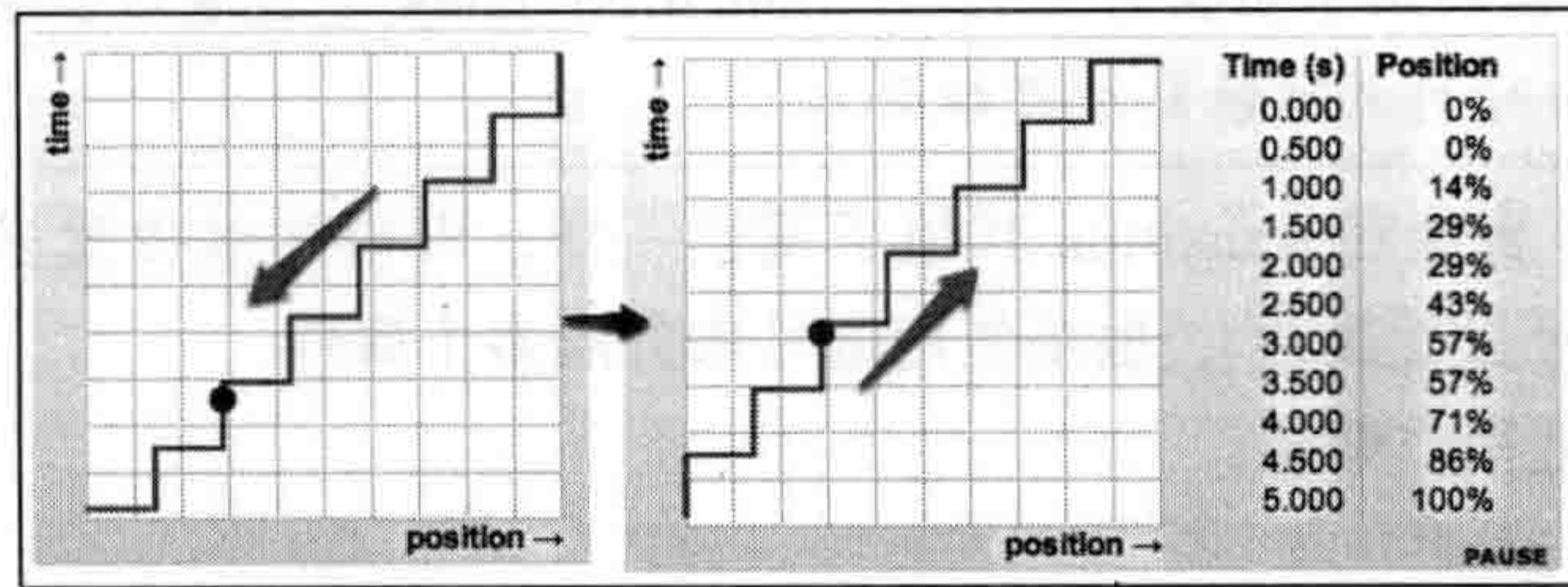
图 12-14 transition-timing-function 取值 step(7,end) 动画曲线
