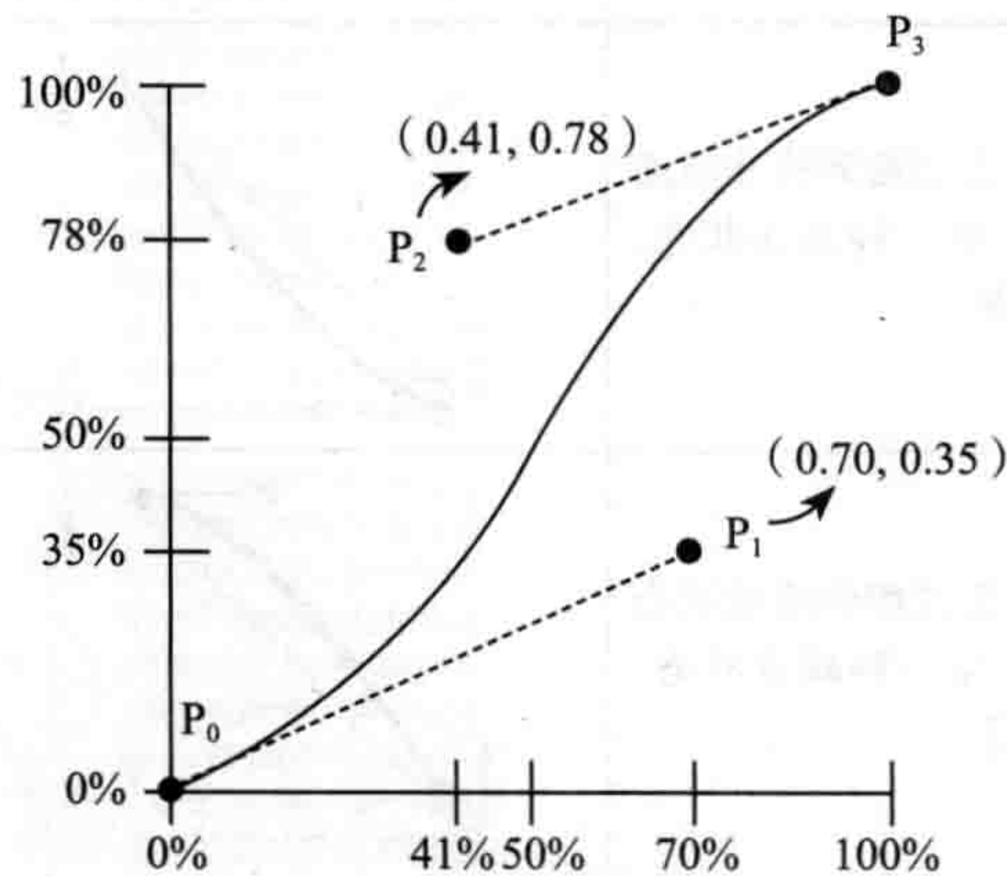
图 12-7 调整三次贝塞尔曲线
