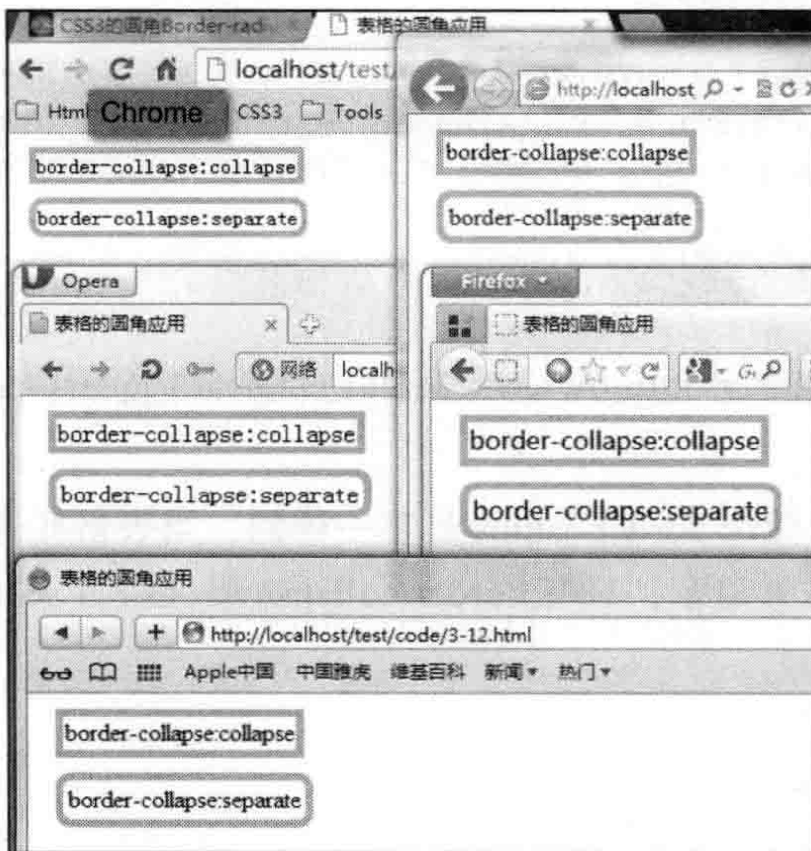
图 3-33 各浏览器下表格圆角边框效果
