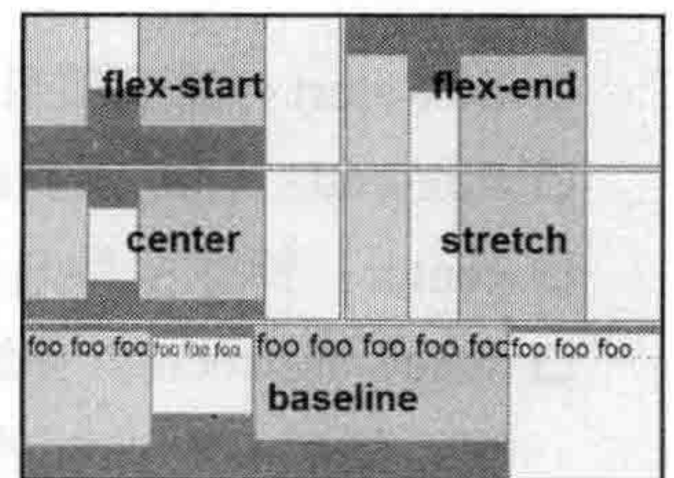
图 8-53 展示 align-items 属性各关键词对伸缩项目的效果
