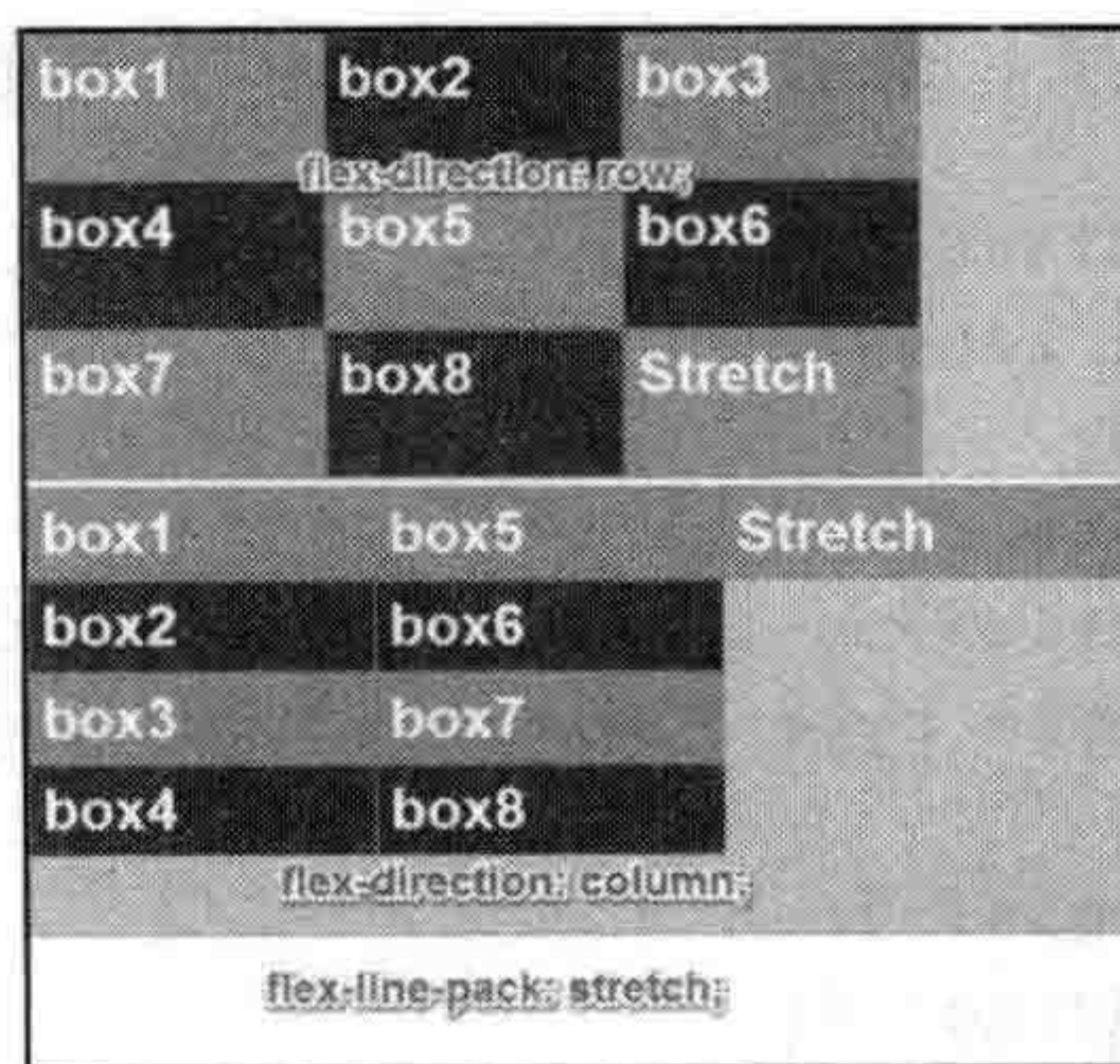
图 8-49 flex-line-pack 取值为 stretch 的效果
