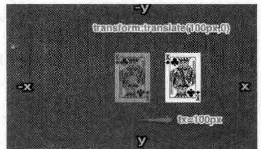
图 11-22 translate() 函数让元素向右移动
