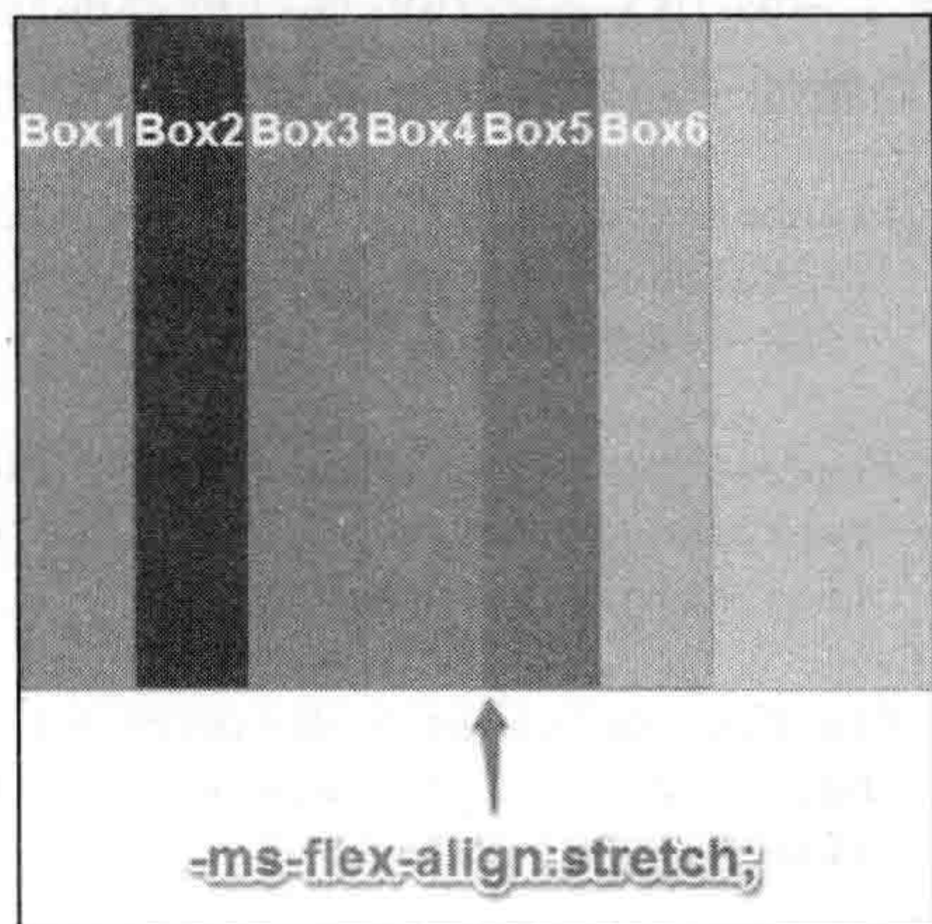
图 8-43 flex-align 取值为 stretch 的效果
