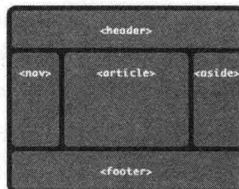
图 8-60 order 修改布局顺序
