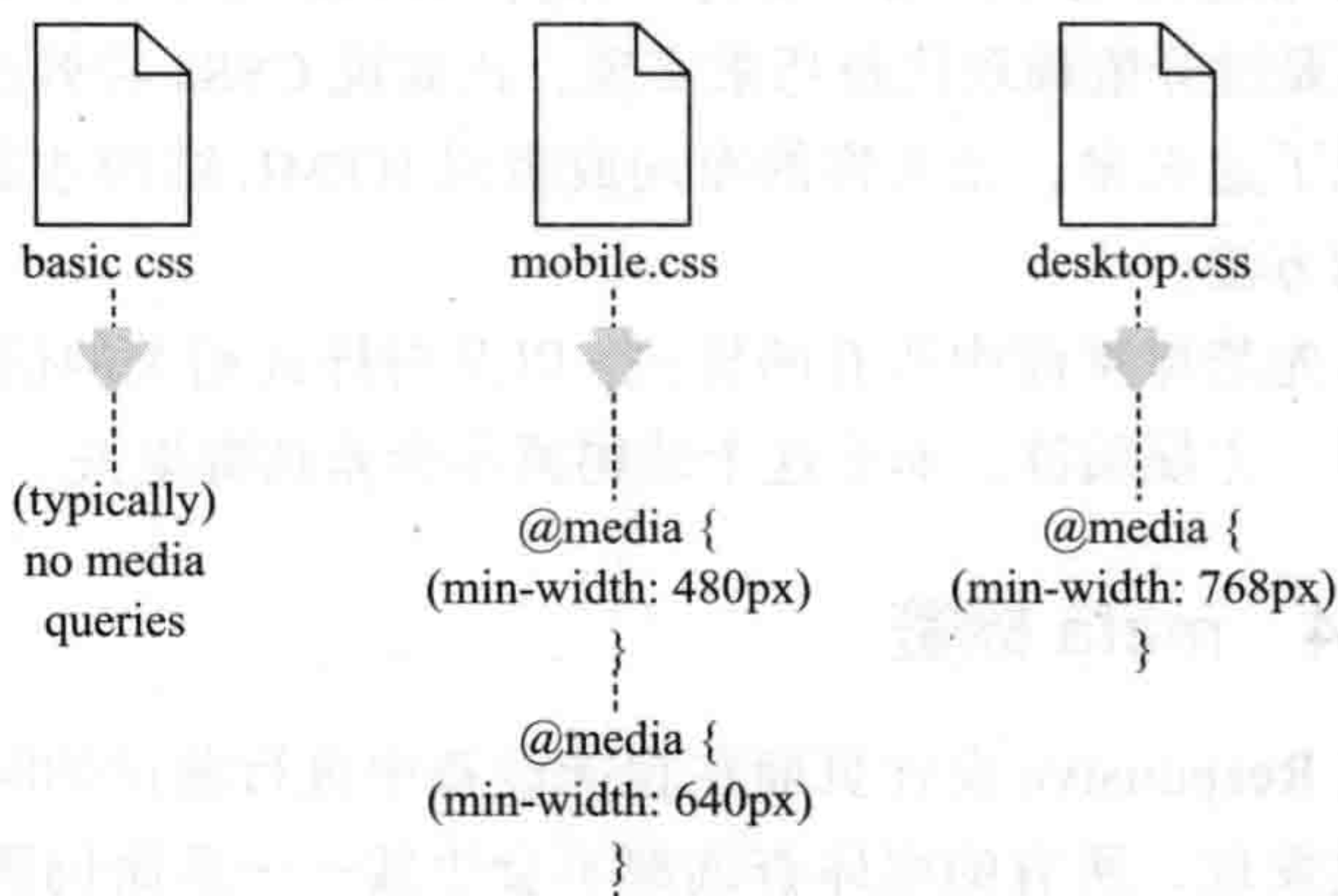
图 14-2 不同断点加载不同样式文件
