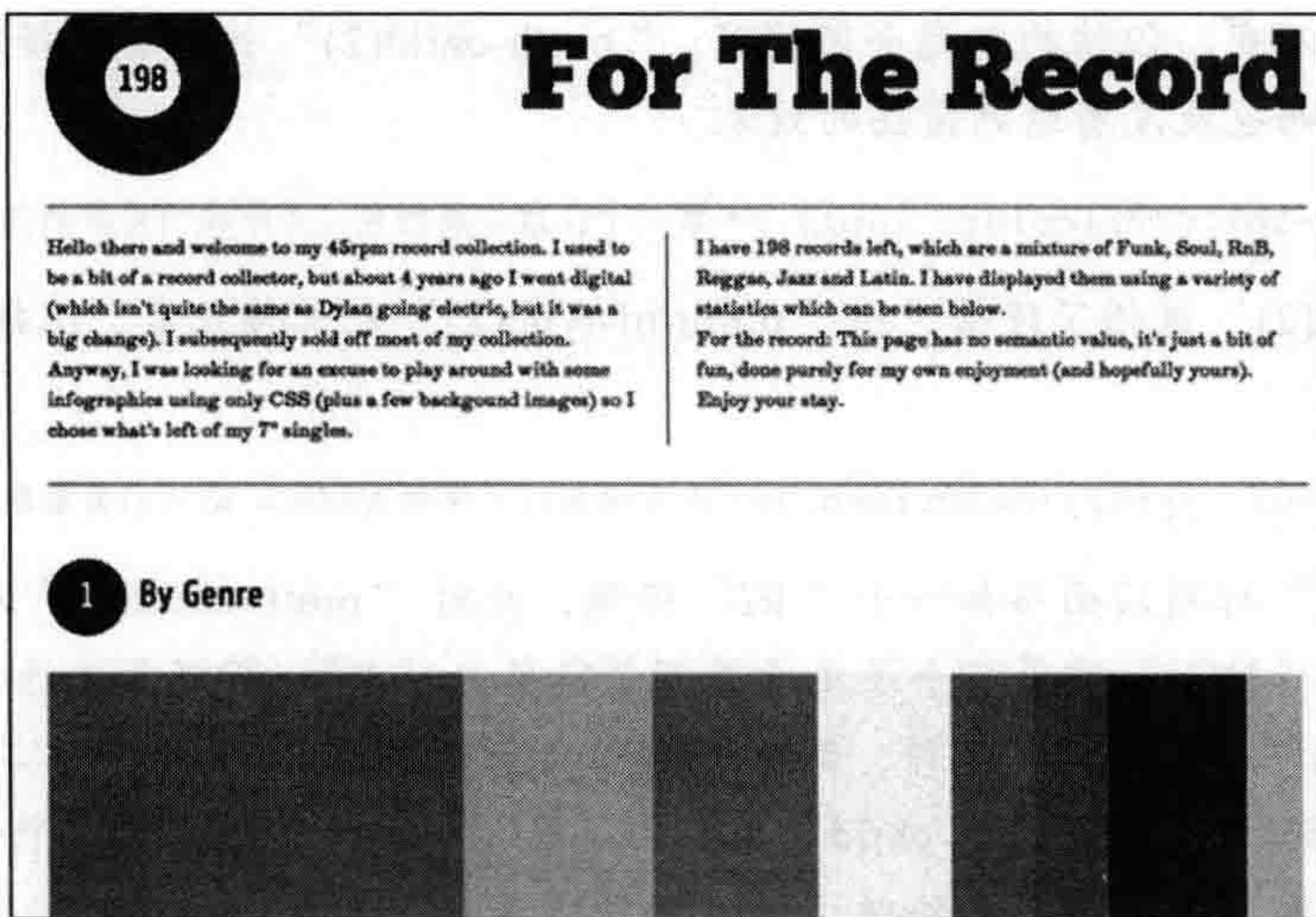
图 2-42 “For The Record” 站点使用 :nth-of-type 的效果
