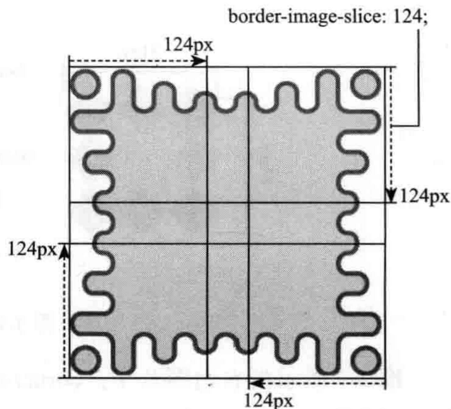
图 3-5 border-image-slice 以 124px 位置切图
