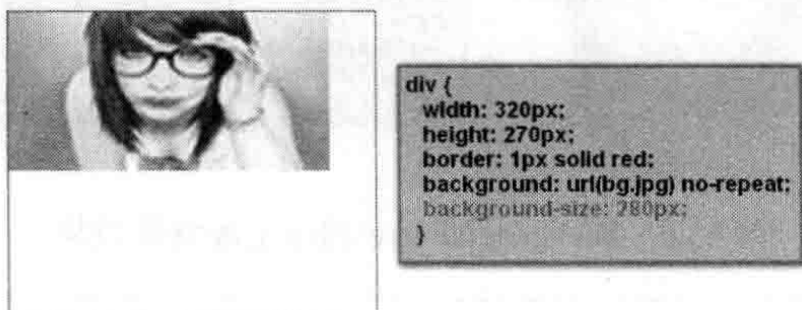
图 4-17 background-size 取一个值的效果
