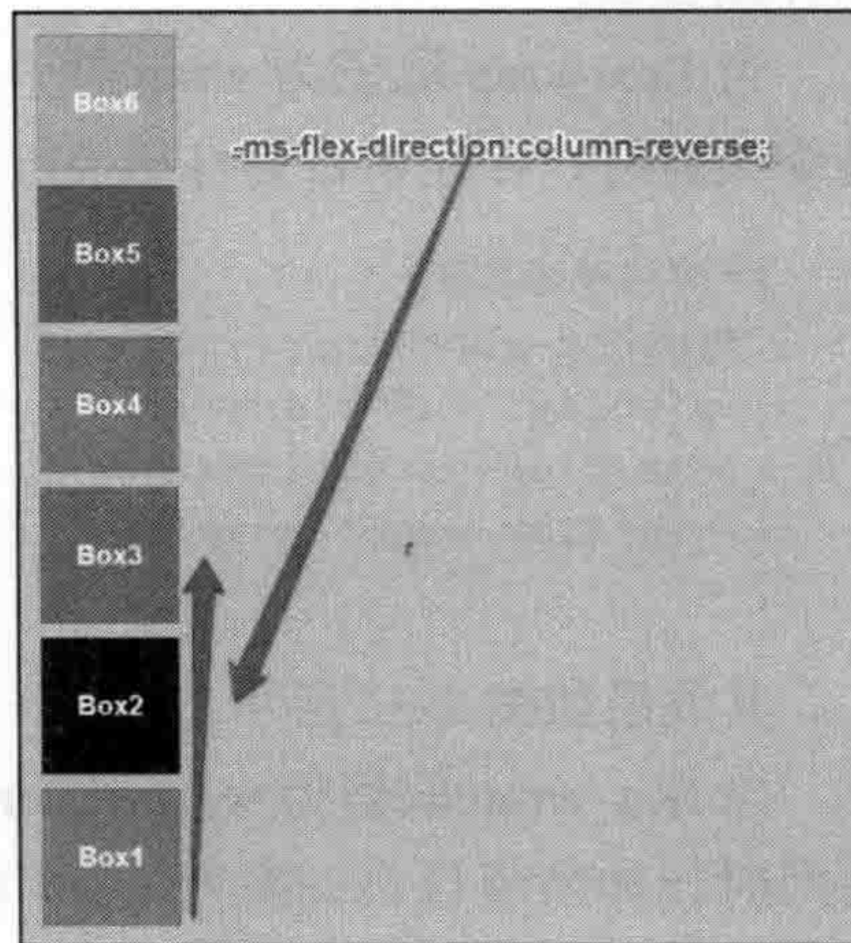
图 8-30 flex-direction 取值为 column-reverse 的效果
