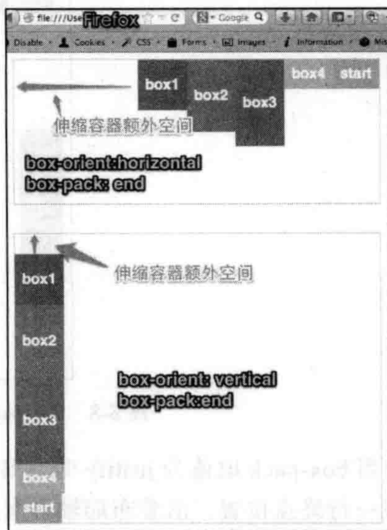
图 8-7 box-pack 取值为 end 在 Firefox 的效果
