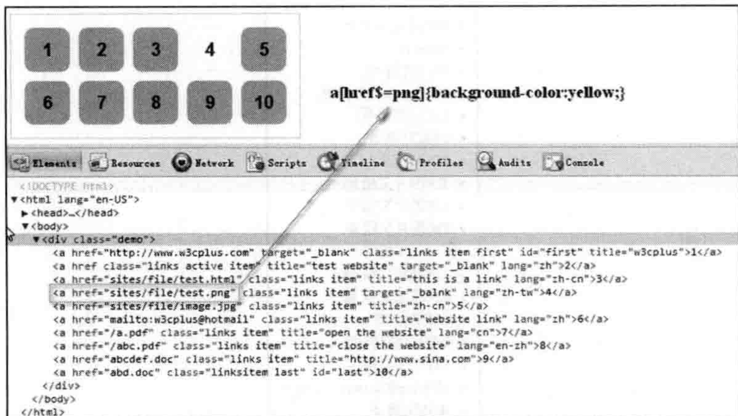
图 2-61 E[attr$=val] 属性选择器的使用效果
