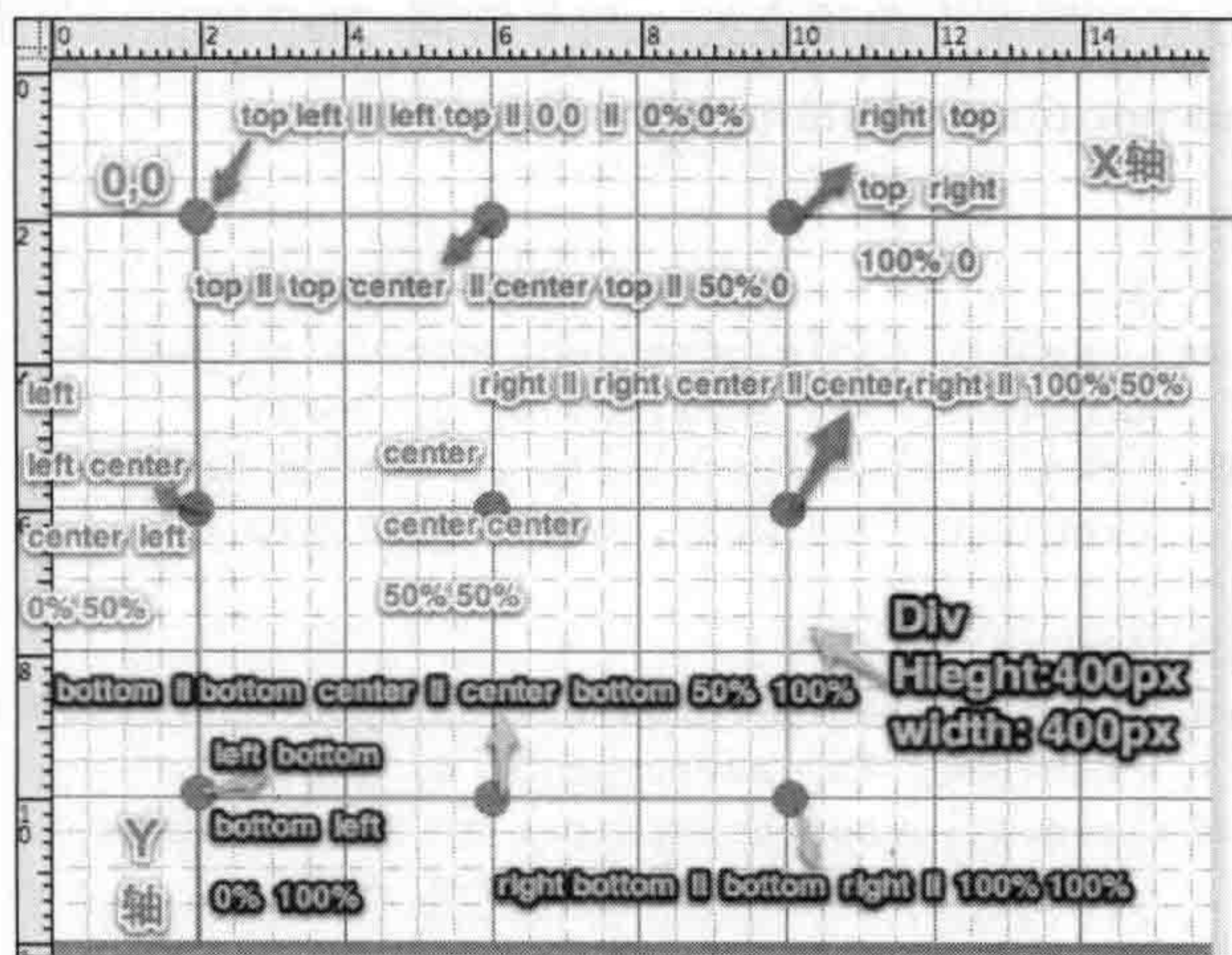
图 10-39 设置径向渐变圆心位置关键词对照
