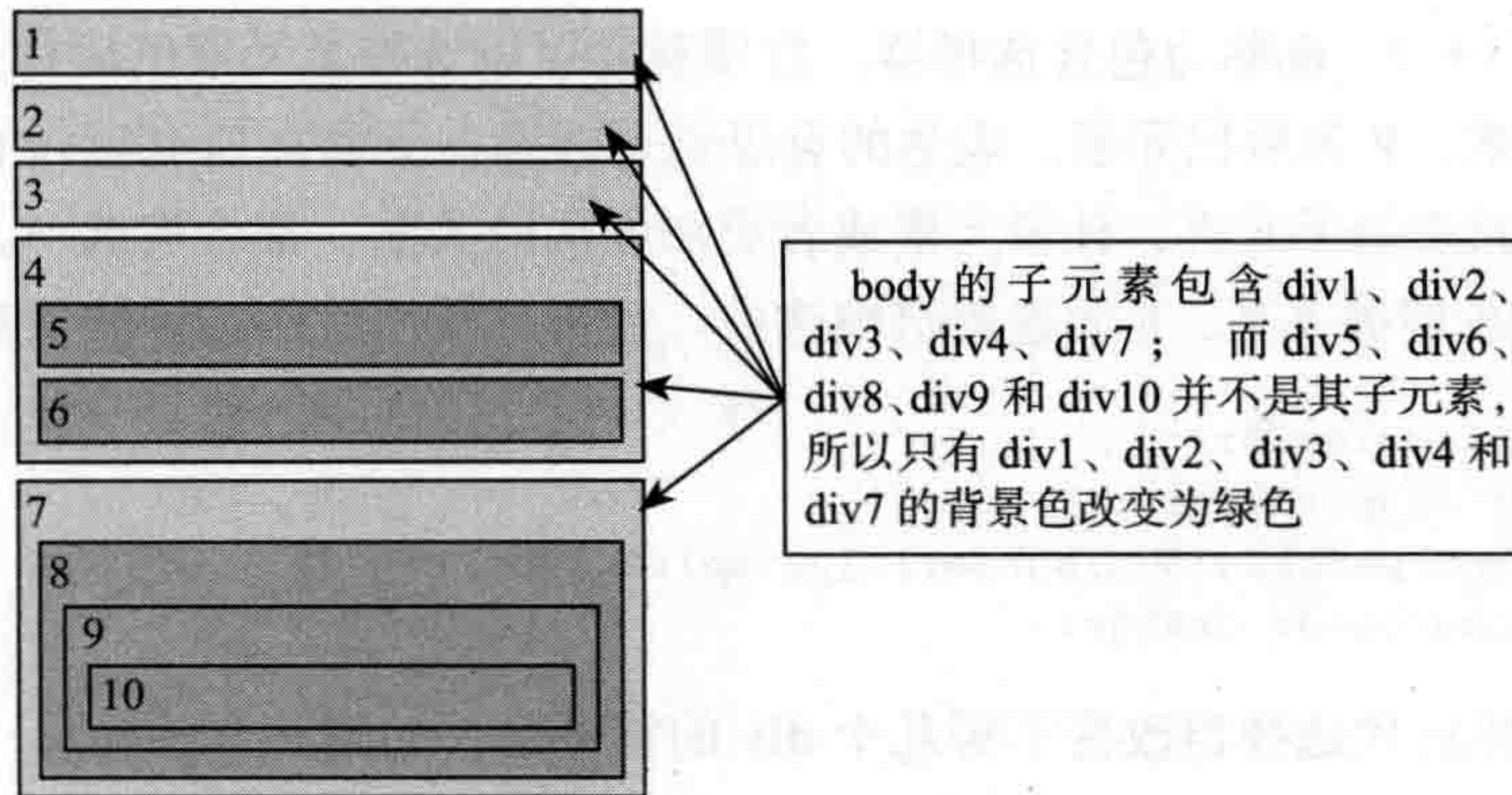
图 2-11 使用子选择器的效果
