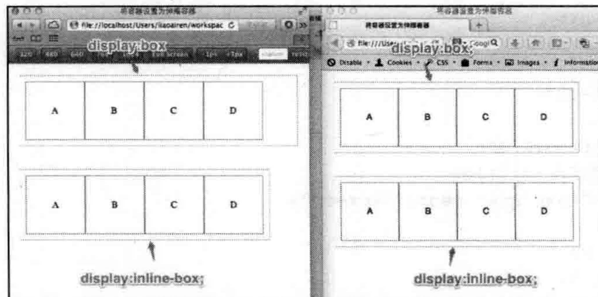
图 8-2 Safari 和 Firefox 下伸缩器的设置效果
