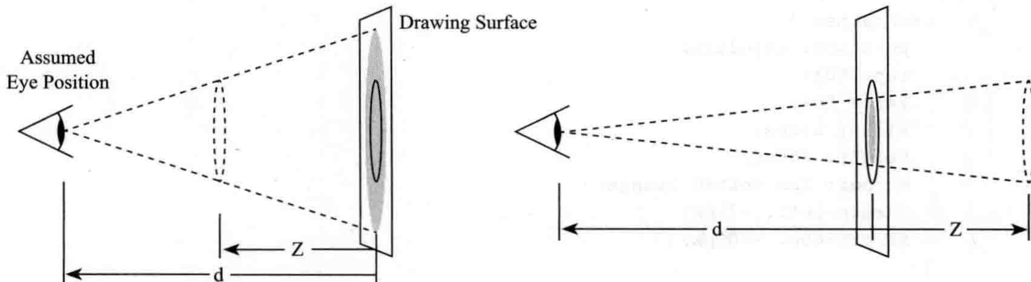
图 11-13 perspective 和 translateZ 的关系
