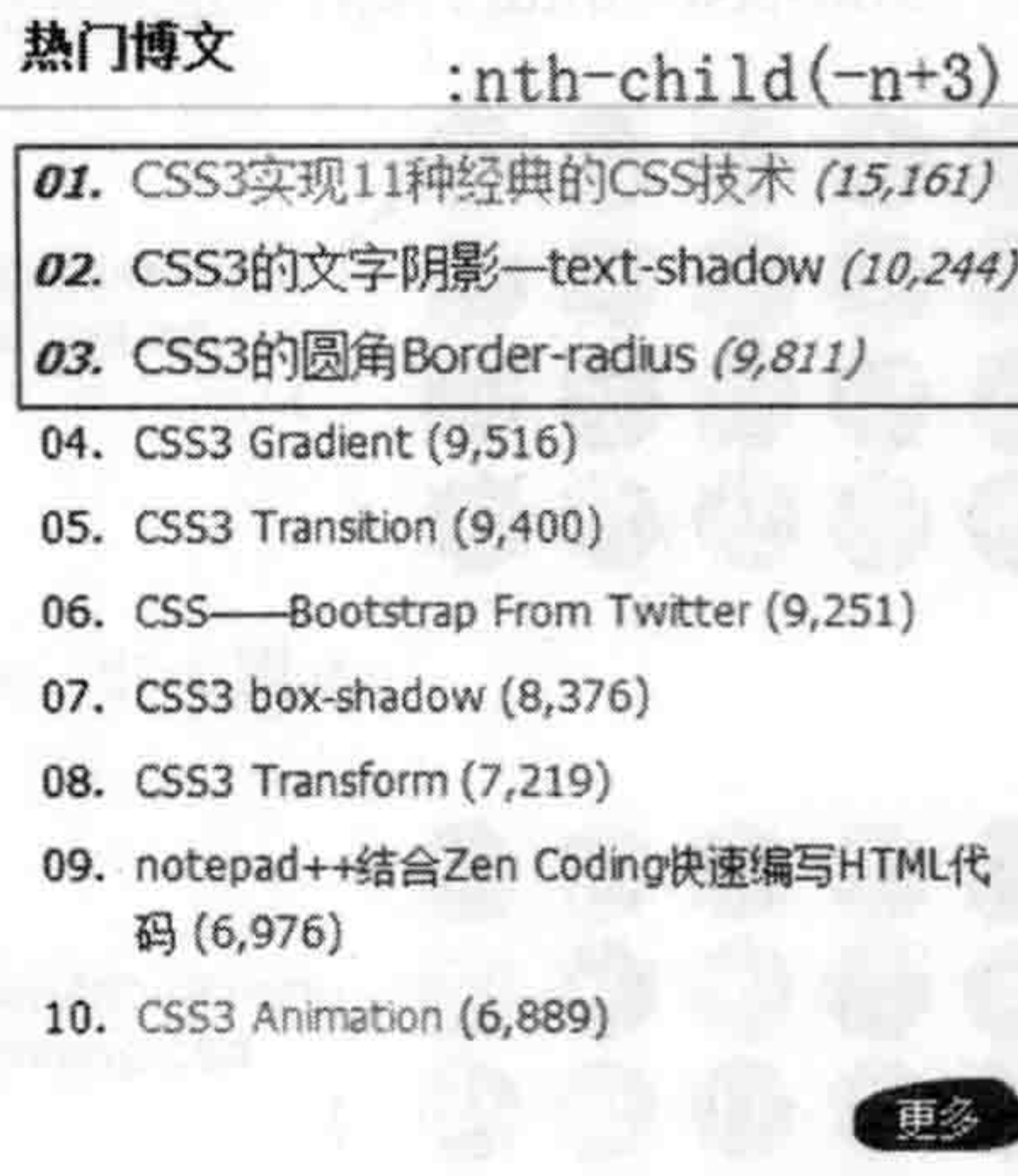
图 2-35 热点博文排在前三的特殊效果
