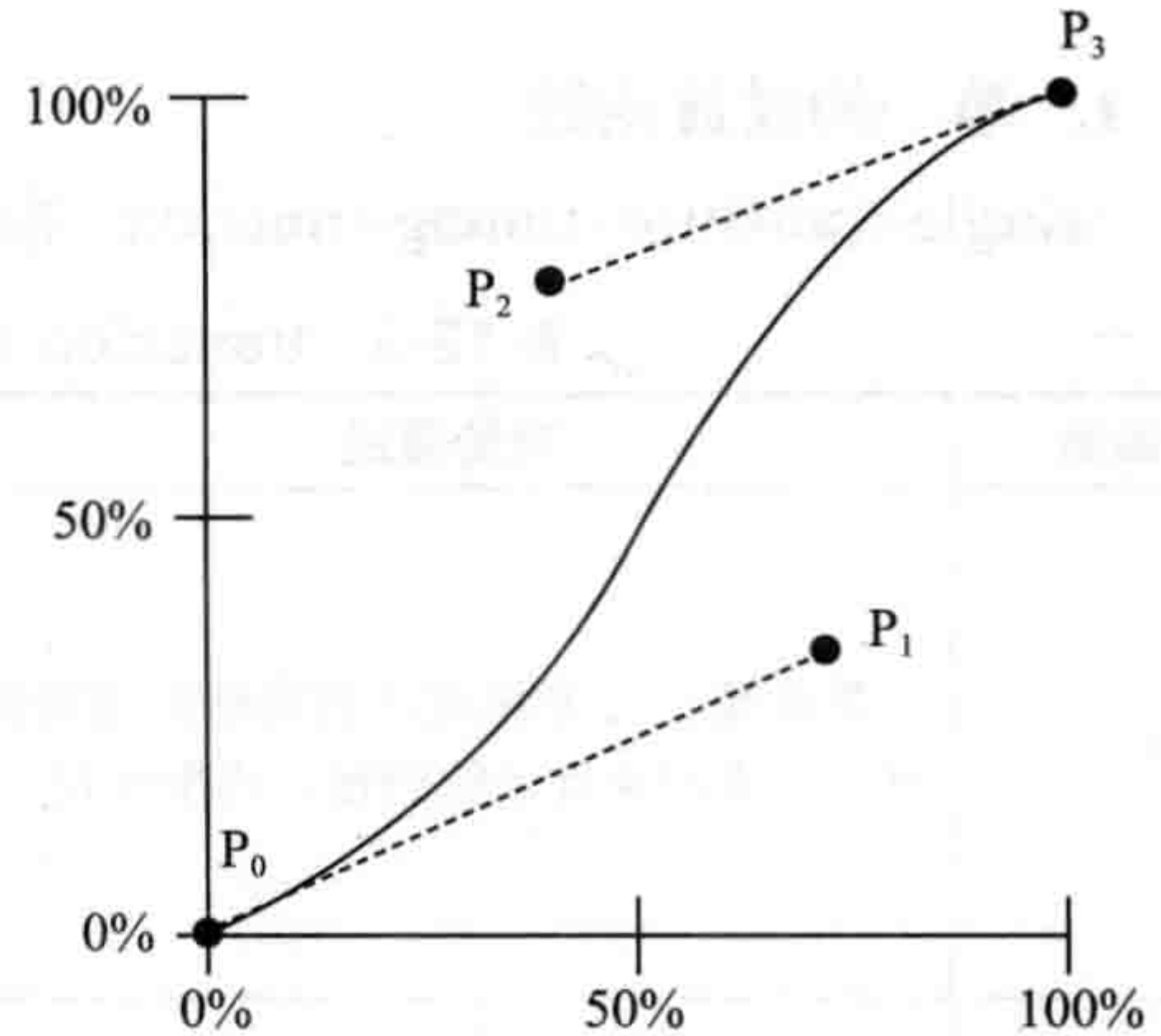
图 12-6 带有控制点的三次贝塞尔曲线
