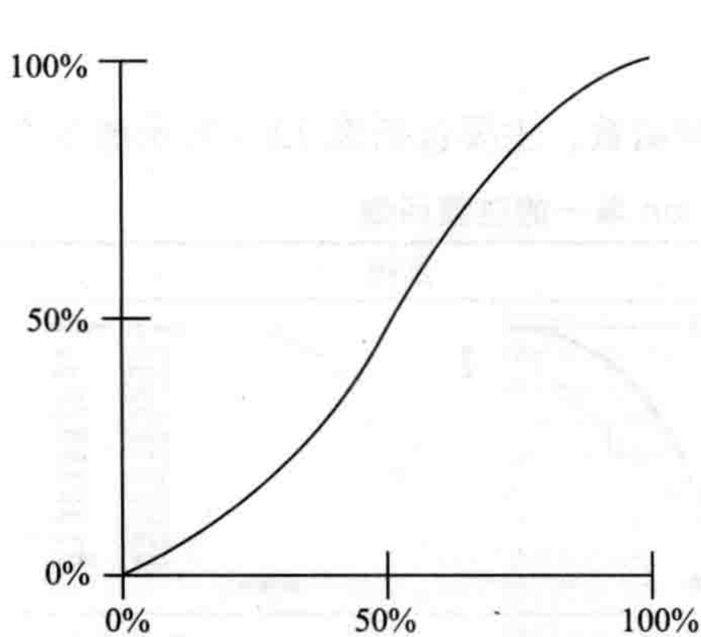
图 12-5 三次贝塞尔曲线
