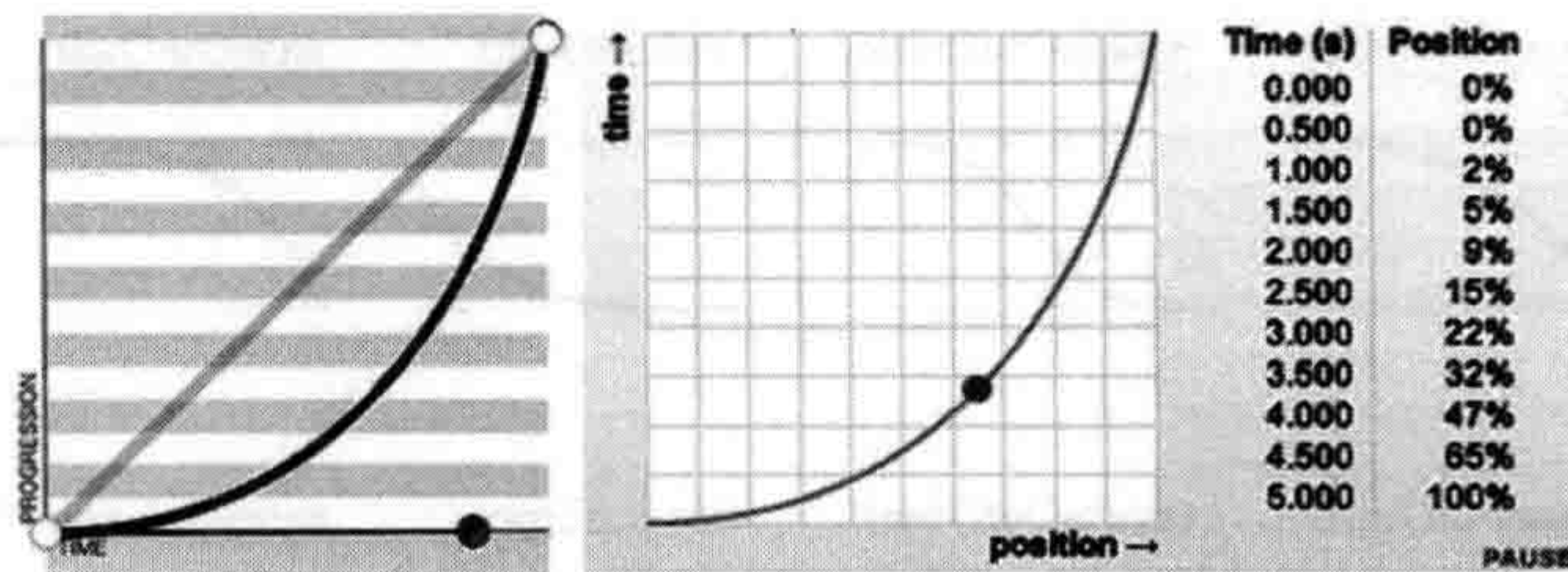
图 12-9 transition-timing-function 取值为 cubic-bezier (.85, 0, 1, 1) 的运动曲线
