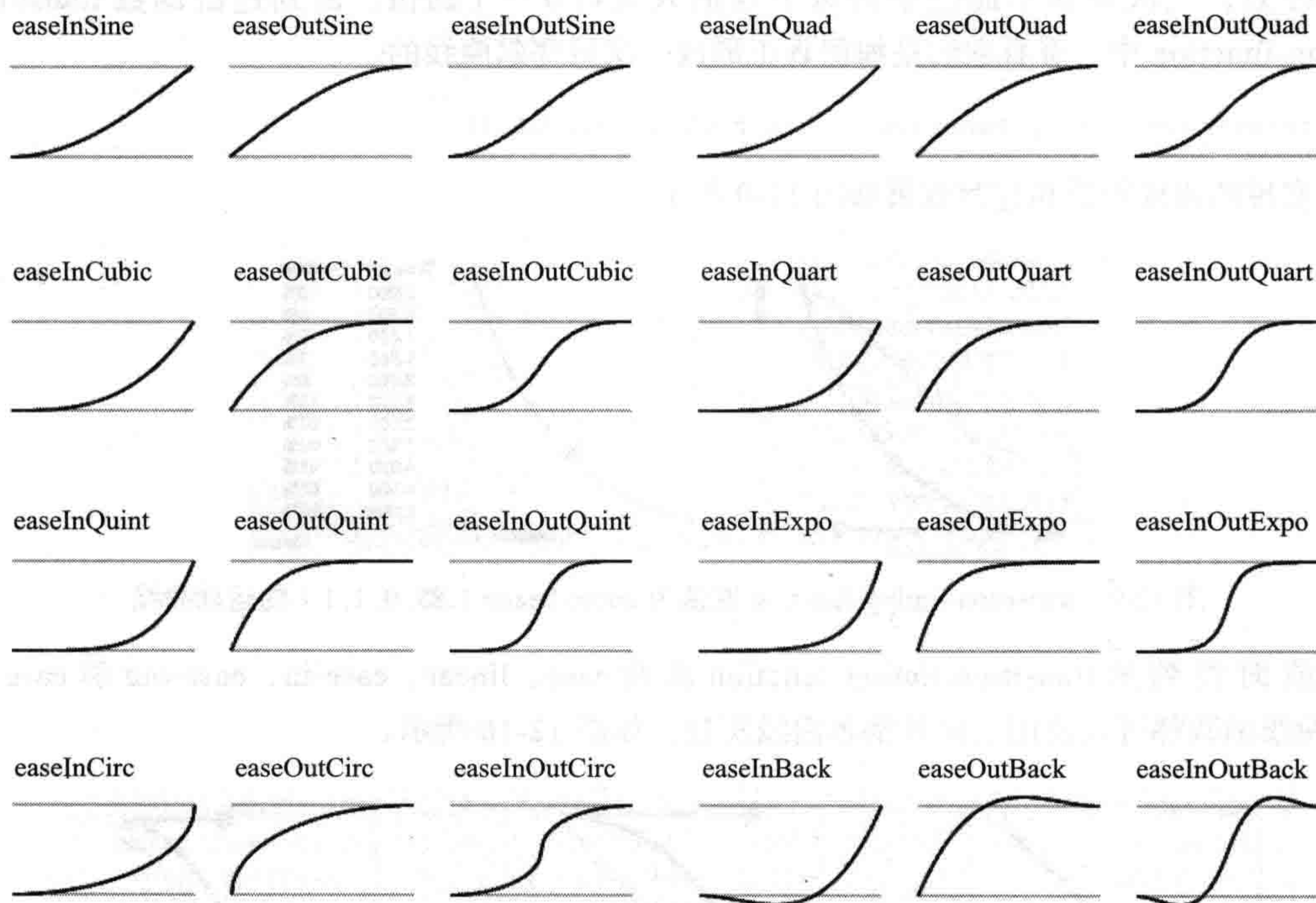
图 12-11 easing function 曲线
