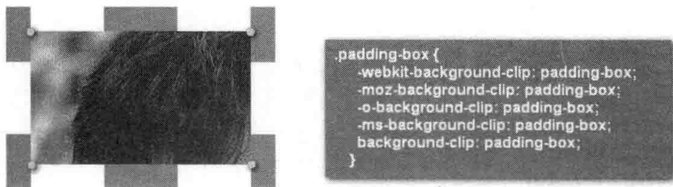
图 4-10 background-clip 的属性设置为 padding-box 的效果
