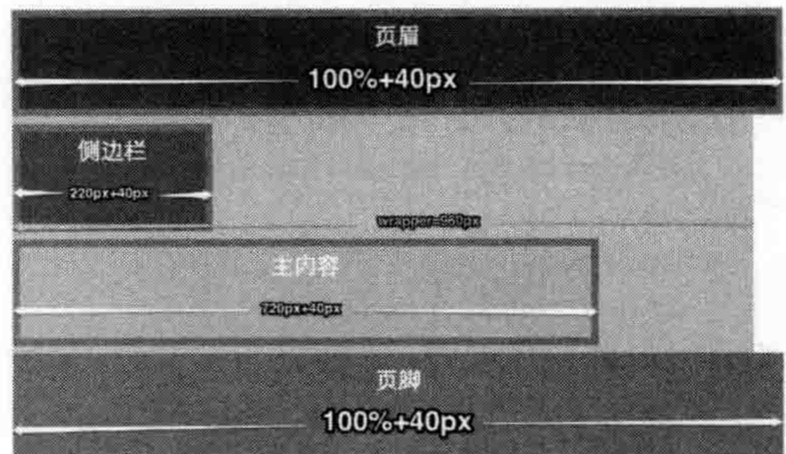
图 7-7 padding 和 border 撑破布局
