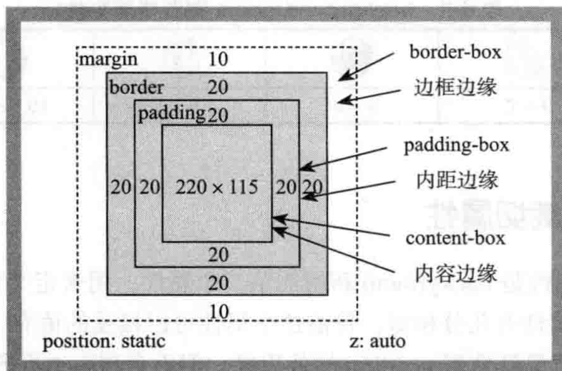
图 4-6 具有背景的元素盒子模型
