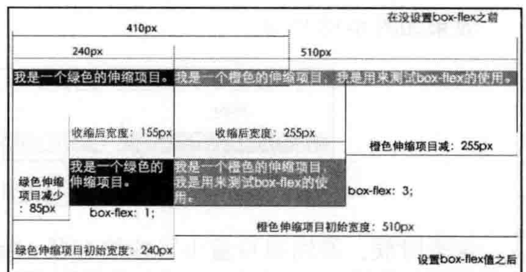
图 8-20 box-flex 的比例 3 : 1，伸缩项目收缩的效果
