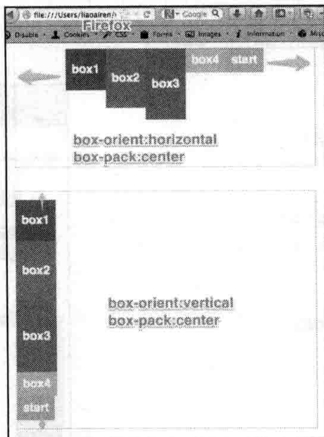
图 8-8 box-pack 取值为 center 在 Firefox 的效果
