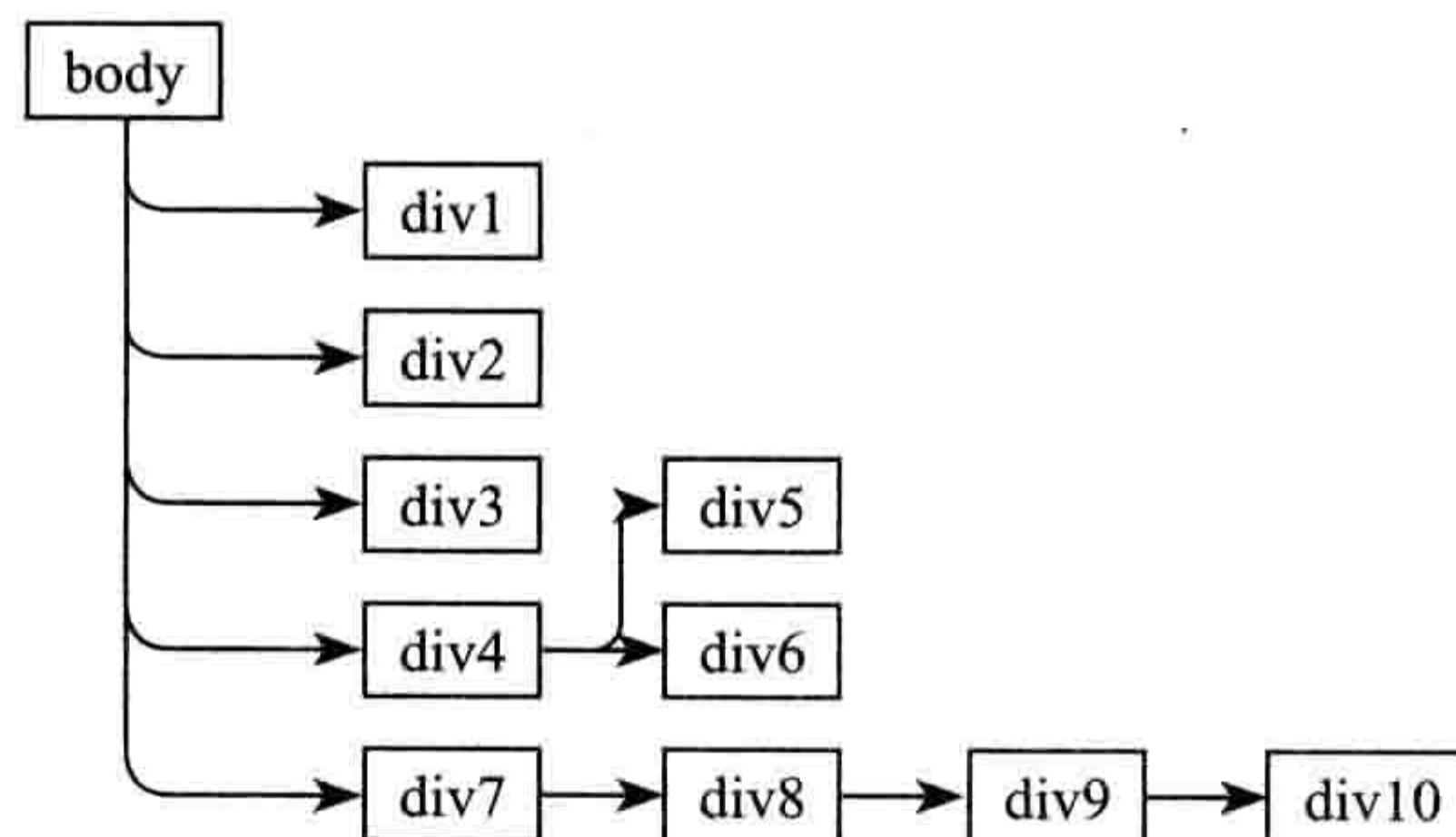
图 2-9 body 的树形结构
