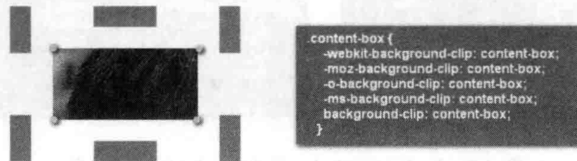
图 4-11 background-clip 设置为 content-box 的效果
