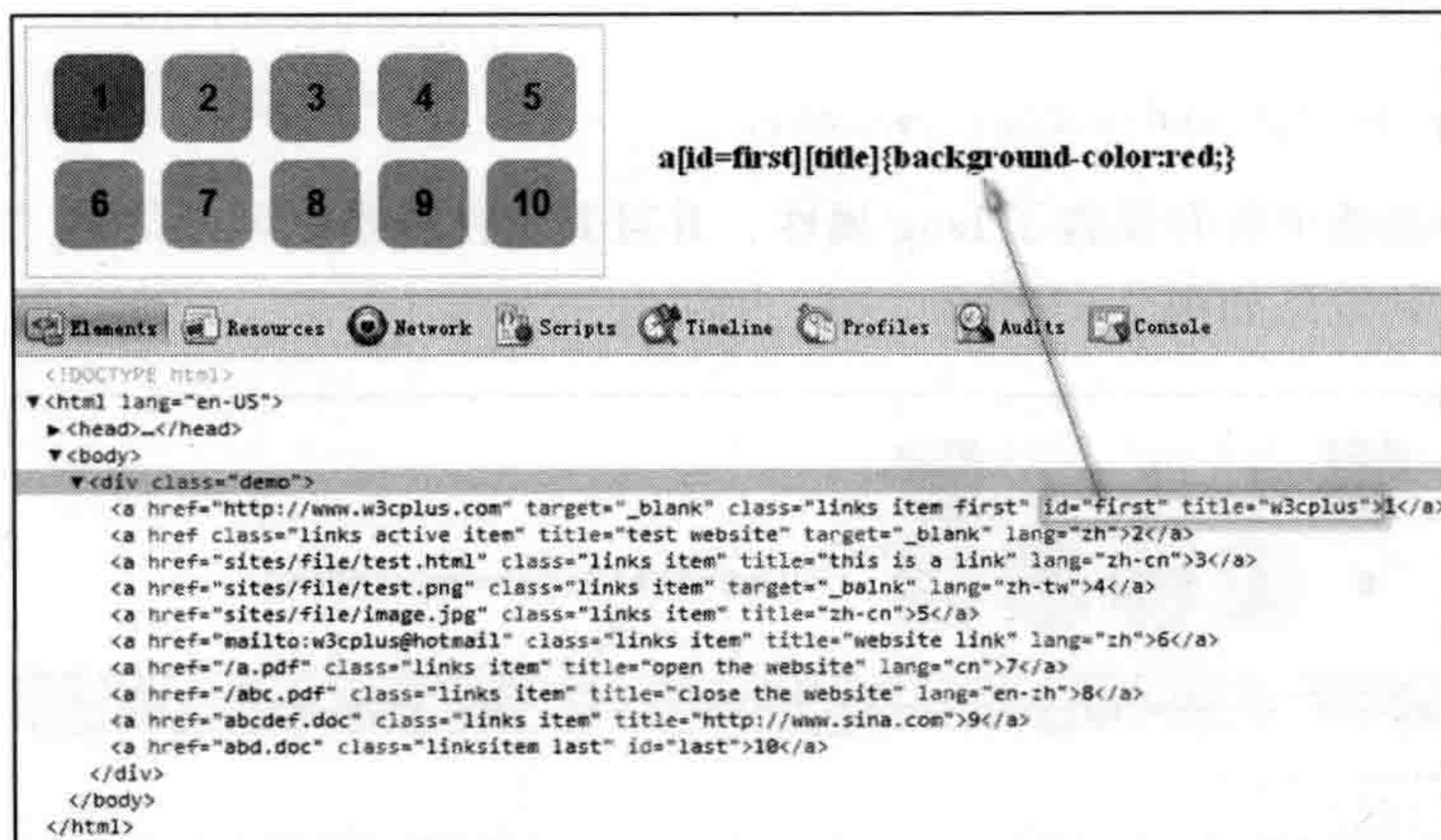
图 2-55 E[attr1][attr2] 多属性选择器使用效果
