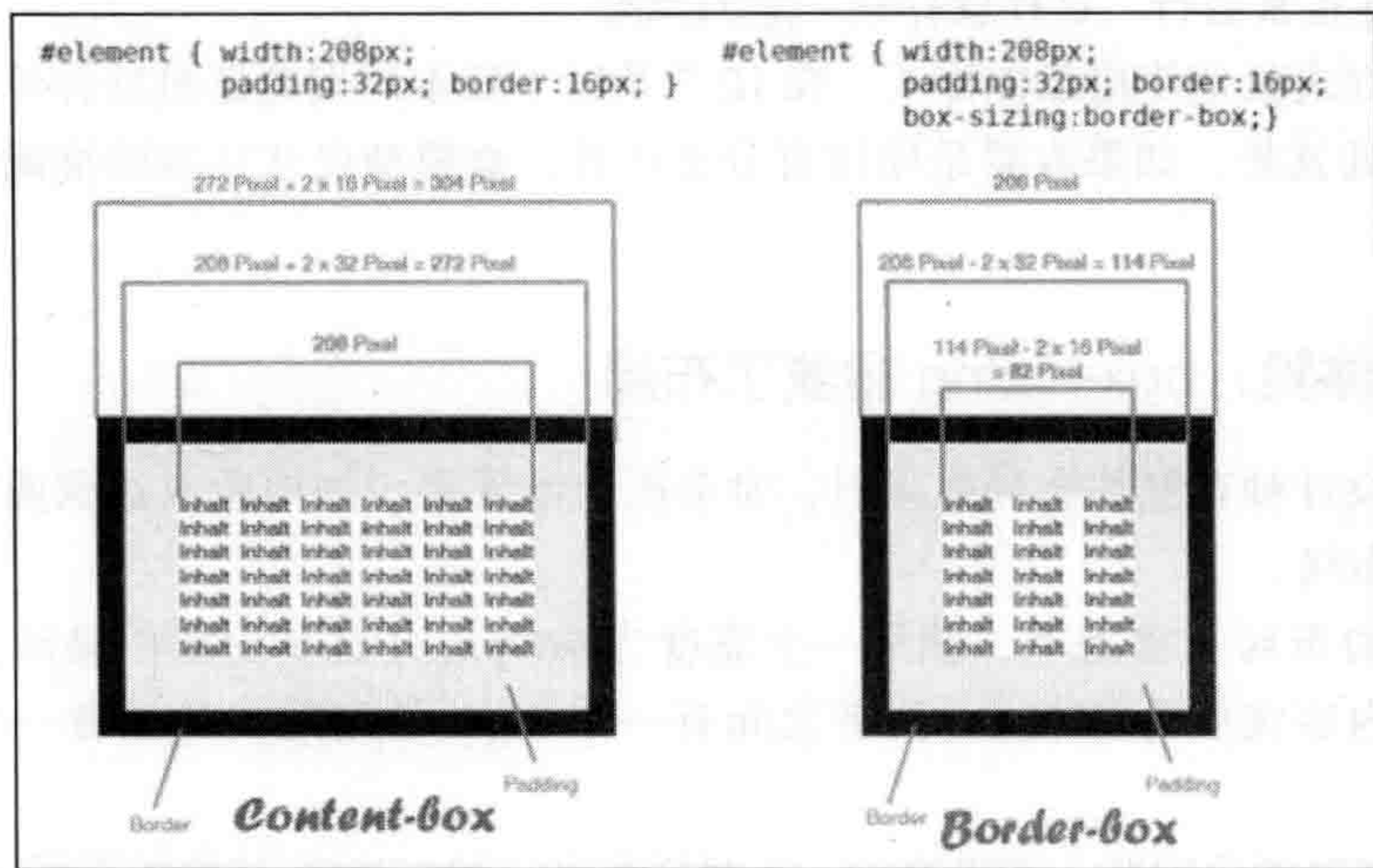
图 7-3 box-sizing 中 content-box 和 border-box 解析模式的对比
