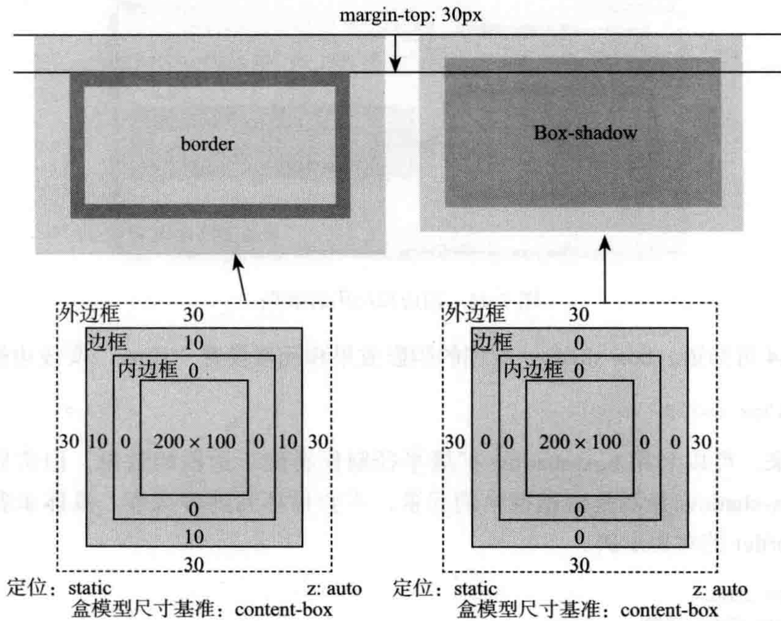
图 3-45 border 与 box-shadow 制作边框效果对比
