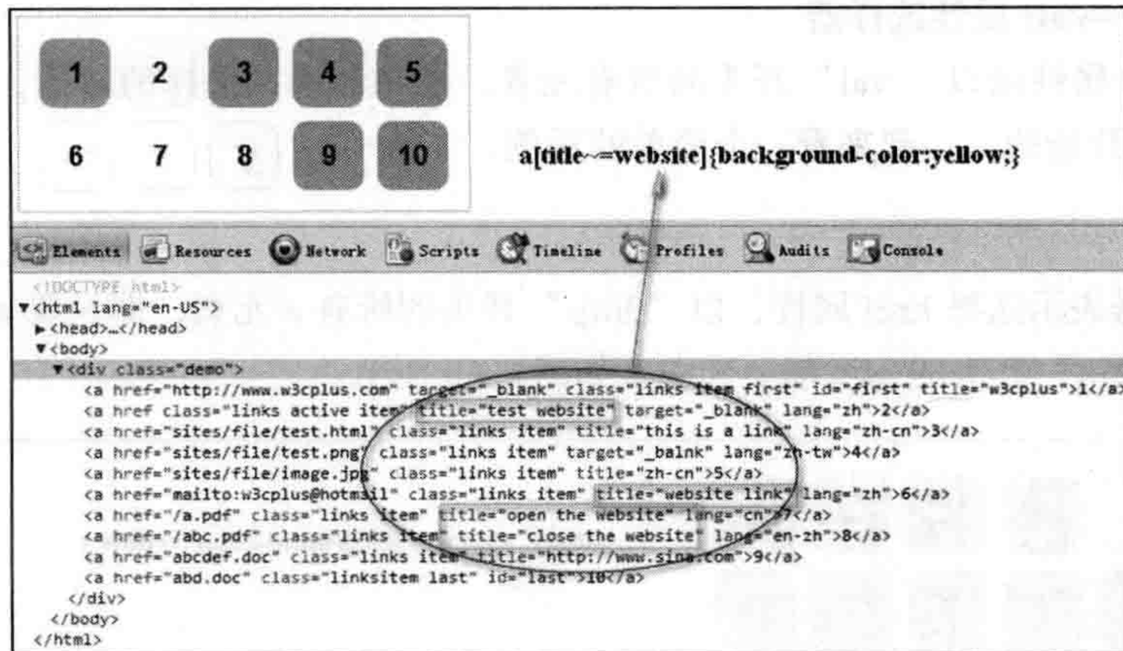
图 2-58 E[attr~='val'] 选择器的使用效果
