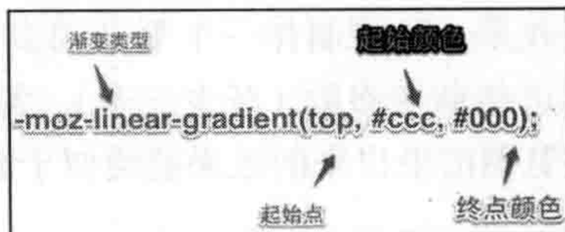
图 10-3 Gecko 引擎的线性渐变语法
