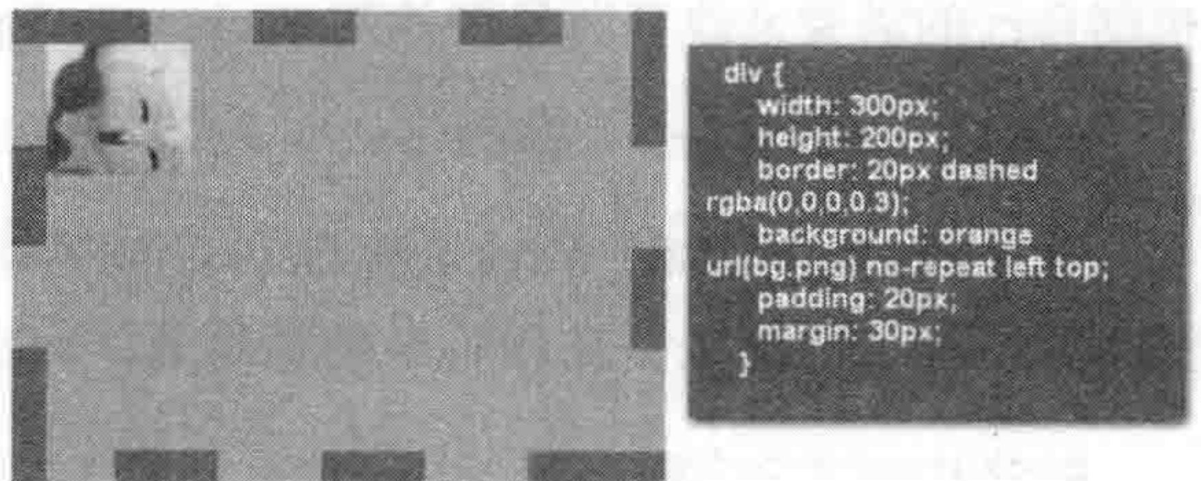
图 4-2 div 默认背景图片设置效果
