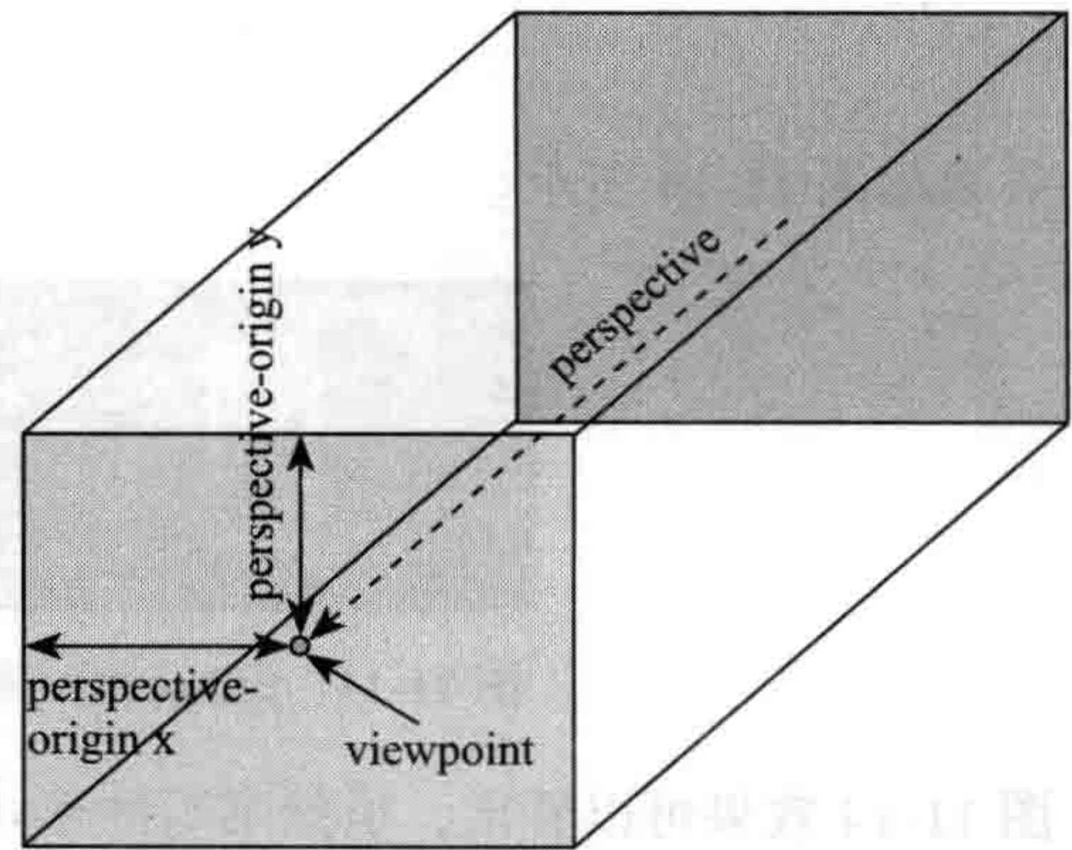
图 11-15 perspective-origin 与 perspective 结合使用示意图
