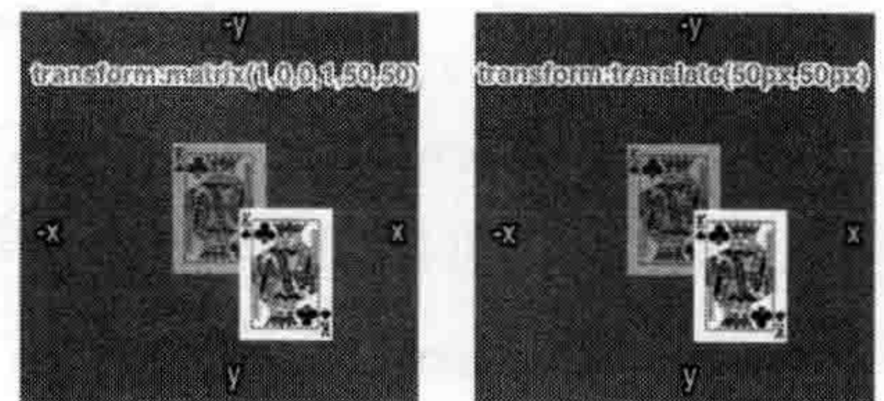
图 11-39 matrix(1,0,0,1,50,50) 和 translate(50px,50px) 效果对比
