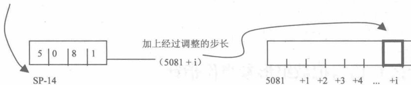
图 9-3 下标形式的数组形参是如何引用的
