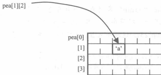
图 10-1 假想中的二维数组内存布局
