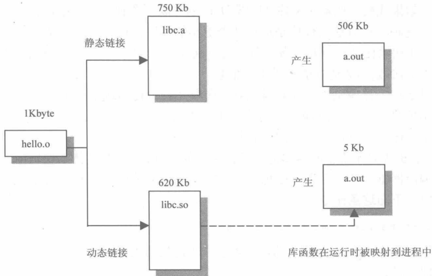
图 5-2 静态链接与动态链接
