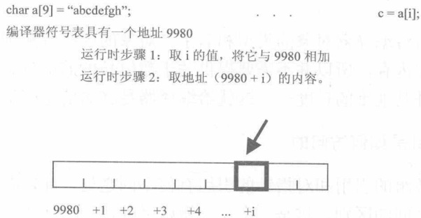
图 A 数组的下标引用
