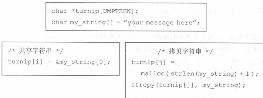
图 10-5 创建一个锯齿状数组
