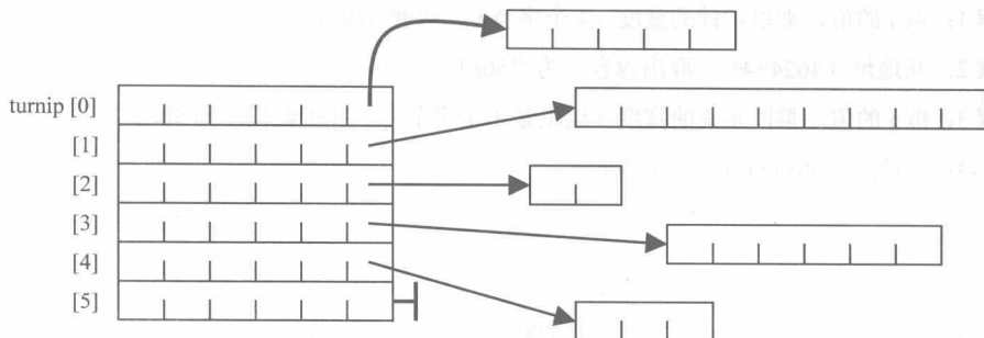
图 10-4 锯齿状字符串数组
