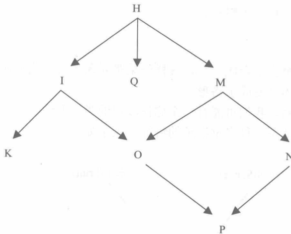
图 11-3 多重继承
