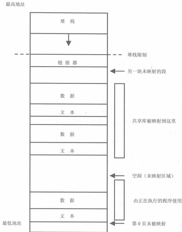
图 6-3 显示共享库的虚拟地址空间布局
