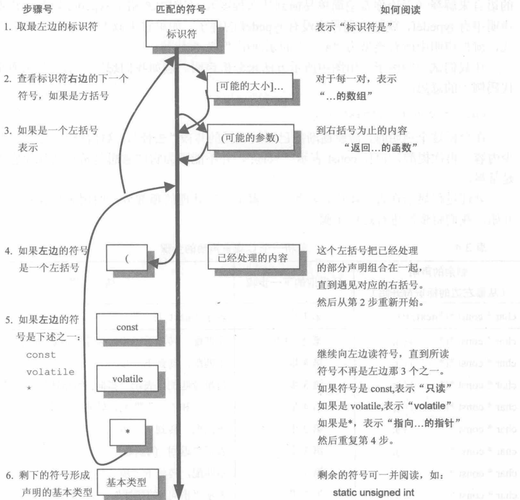
图 3-1 如何解析 C 语言的声明
