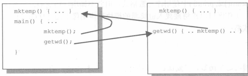
图 5-3 Interpositioning 和缺省全局作用域示意图
