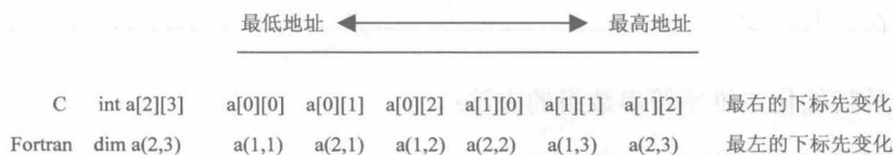
图 9-9 行主序 vs.列主序
