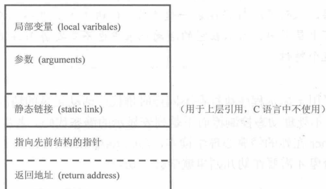
图 6-4 过程活动记录的规范描述
