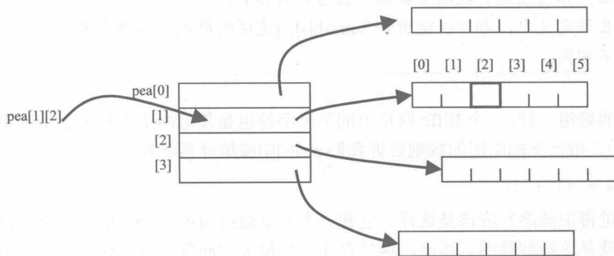
图 10-3 指向字符串的指针数组
